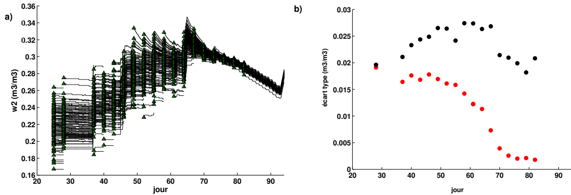
FIG. 4.7: a) Evolution temporelle et effondrement d'un ensemble de 100 membres avec la méthode EnKF "pure". A chaque observation, les membres de l'ensemble corrigé sont dessinés en triangles verts. La trajectoire de chaque ensemble entre deux observations est représentée par une ligne continue noire. b) Ecart type de l'ensemble avec la méthode EnKF "pure" (points rouges) et avec l'EnKF avec un facteur d'inflation (points noirs).
