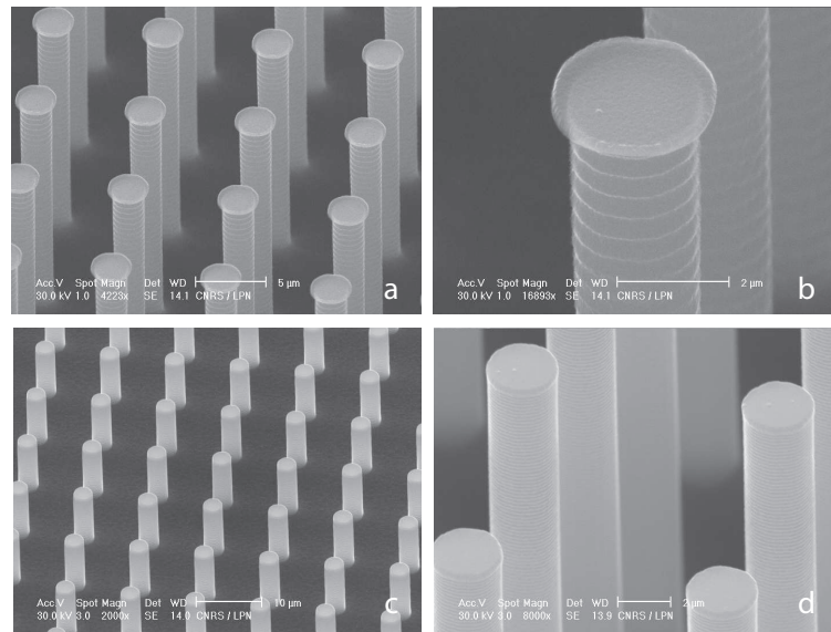
FIG. 2.7: Images MEB d'échantillons texturés. a et b : Premiers échantillons obtenus par DRIE. On observe une sous-gravure sous le masque d'aluminium ainsi qu'une forte rugosité de surface le long des piliers. c et d : Amélioration du procédé de gravure. La sous-gravure a disparu et les flancs sont beaucoup plus lisses.
