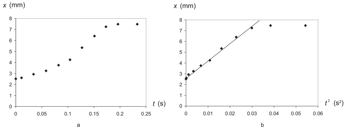
FIG. 6.7: Évolution de la position au cours du temps (a) d'une goutte de 10\ \mu\text{L} sur un gradient de 5.8\%/mm oscillant à 43\ \text{Hz} . (b) Le tracé de x en fonction de t^2 permet de voir que la goutte avance avec une accélération constante avant d'être arrêtée brusquement. La pente de la droite pointillée nous donne l'accélération de la goutte, qui vaut ici 140\ \text{mm/s}^2 .
