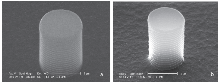
FIG. 2.16: Comparaison d'un plot en silicium de 3\ \mu\text{m} de diamètre et de 4\ \mu\text{m} de haut (a) avec sa réplique polymère (b).
