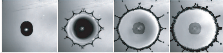
FIG. 5.44: Vue aérienne d'un impact de goutte d'eau lâchée de 38.5 cm de haut ( V = 2.6 \text{ m/s} , R_0 = 1.9 \text{ mm} , p = 10 \mu\text{m} , h = 10 \mu\text{m} ). Les images sont espacées de 1 ms. La figure d'impact laisse apparaître une figure à 12 branches.
