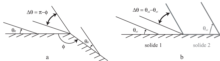
FIG. 1.4: Accrochage de la ligne de contact sur un défaut physique (a) ou chimique (b). La ligne de contact au niveau de l'angle peut basculer et l'angle de contact au niveau de ce défaut peut prendre plusieurs valeurs dans l'intervalle schématisé par la double flèche.
