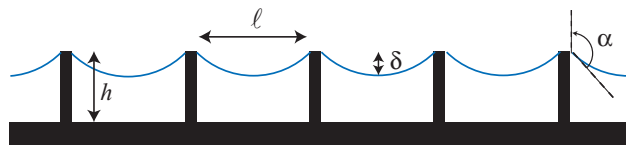
FIG. 4.11: Schéma de l'interface liquide/vapeur sous une goutte en état fakir. On note \delta la distance entre le bas de l'interface et le sommet des micropiliers et \alpha l'angle entre la verticale et la tangente à l'interface au niveau d'un angle de pilier.
