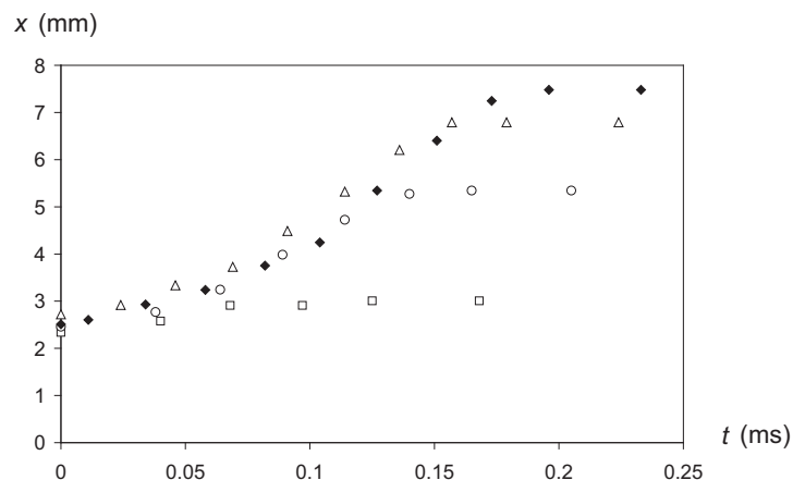
FIG. 6.8: Position d'une goutte de 10\ \mu\text{L} sur un gradient de 5.8\%/mm en fonction du temps, pour des oscillations d'une fréquence de 35\ \text{Hz} \square , 39\ \text{Hz} \circ , 43\ \text{Hz} \blacklozenge et 45\ \text{Hz} \triangle .
