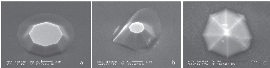
FIG. 2.14: Images MEB de plots issus de la gravure chimique au TMAH. a : pyramide de 15 \mu\text{m} de haut, 55 \mu\text{m} de diamètre supérieur. Le masque initial de silice faisait 100 \mu\text{m} de diamètre et la gravure a duré 20 minutes. b : Même échantillon gravé plus longtemps (30 minutes). La hauteur du plot fait 22 \mu\text{m} , le diamètre supérieur 30 \mu\text{m} . On voit que la couche de silice d'épaisseur 200 nm s'est effondrée. c : Échantillon issu d'un masque de 70 \mu\text{m} de diamètre, gravé 30 minutes. Les plans atomiques se sont rejoints et le masque est tombé!
