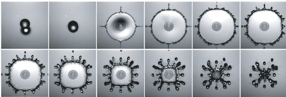
FIG. 5.33: Vue aérienne d'un impact de goutte d'eau lâchée de 45 cm de haut ( V = 2.8 m/s, R_0 = 1.9 mm, p = 10 \mu m, h = 18 \mu m). Les images sont espacées de 1 ms. Les éjections de gouttes, qui sont plus marquées, se font toujours dans les directions du réseau. À la rétraction, le bourrelet acquiert une forme carrée.
