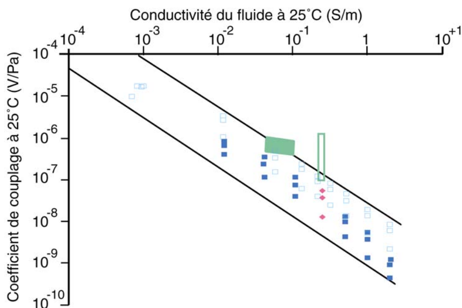
Figure 40: Comparaison des valeurs absolues des coefficients de couplage mesurés sur le Misti par Thouret et coll. (2001) (paralléogrammes verts) avec les valeurs de coefficients de couplage électrocinétiques mesurés en laboratoire. Sur la figure b) sont représentés des coefficients de couplage électrocinétiques mesurés sur des échantillons de cendres andésitiques du Misti (Carré bleu foncé avec une solution de \text{CaCl}_2 , carré bleu ciel avec une solution de \text{NaCl} , losange rose avec une eau synthétique ayant les propriétés de l'eau du captage sur le Misti (cf. texte et tableau 6.2 pour détails)).
