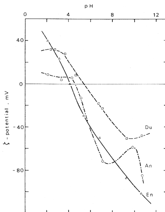
Figure 6: Evolution du potentiel zéta en fonction du pH d'une solution de 10^{-3} mol/L de \text{KNO}_3 pour différents minéraux (An : anorthite ; En : enstatite) et une roche (Du : dunité). Température de mesure 45^\circ\text{C} . D'après Ishido et Mizutani (1981).
