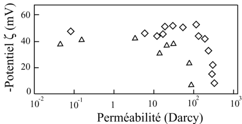
Figure 8: Evolution du potentiel de surface pour des grès de Fontainebleau broyés en fonction de la perméabilité de l'échantillon. Les losanges sont obtenus avec une solution de KCl de résistivité électrique égale à 400 \Omega.m et un pH=7, les triangles sont obtenus avec une solution de KCl de résistivité électrique égale à 1000 \Omega.m et un pH=5.7, d'après Lorne et coll. (1999 a).
