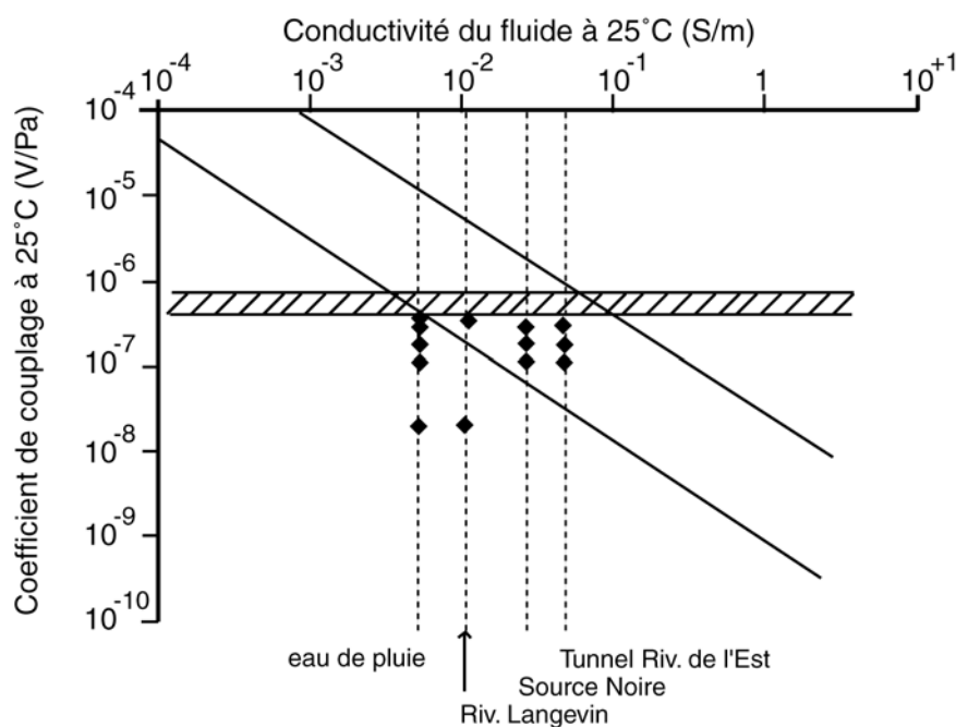
Figure 46: Comparaison des valeurs absolues des coefficients de couplage mesurés sur le Piton de la Fournaise par Lénat et coll. (2000) dans l'Enclos Fouqué (Losanges, cf. texte pour détails) avec les valeurs de coefficients de couplage électrocinétiques mesurés en laboratoire. La zone hachurée représente la valeur des coefficients de couplage d'électrofiltration déduits à partir des résultats de la modélisation de Fontaine et coll. (2002) et des mesures PS de Lénat et coll. (2000).
