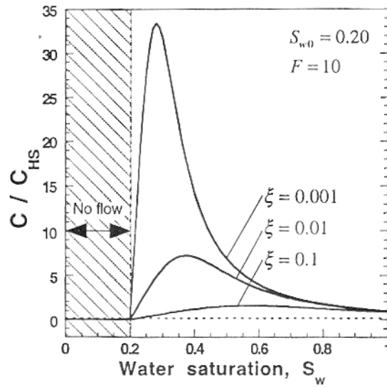
Figure 13: Evolution du coefficient de couplage normalisé par le coefficient de couplage d'Helmholtz-Smoluchowski en fonction de la saturation en eau du réseau poreux, dans le domaine des hautes salinités, prévue par le modèle de Revil et coll. (1999 b) 2
