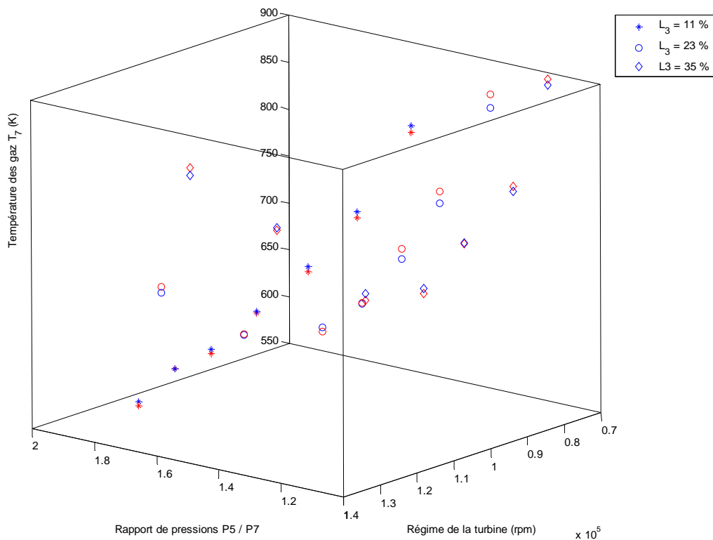
Figure 4.38 – Validation du modèle de température des gaz en sortie de la turbine, données expérimentales : motifs bleus, modèle : motifs rouges. Er_{moy} = 6.1\% , Er_{max} = 8.6\% .
