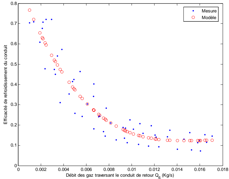
Figure 4.23 – Validation du modèle d'efficacité de refroidissement du conduit de retour d'EGR, Er_{\text{moy}} = 4.3\% , Er_{\text{max}} = 6.9\% .
