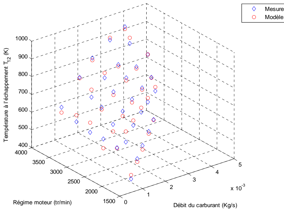
Figure 4.20 – Validation du modèle de température des gaz sortant de la chambre de combustion, Er_{moy} = 8.7\% , Er_{max} = 12.9\% .
