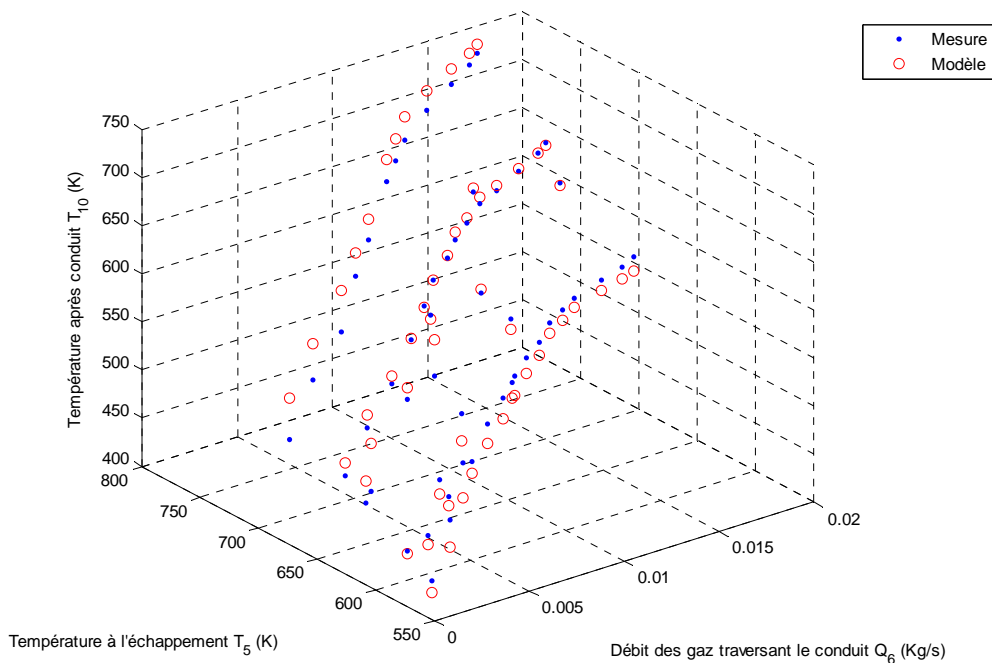
Figure 4.24 – Validation du modèle de température des gaz sortant du conduit de retour d'EGR, Er_{\text{moy}} = 5.7\% , Er_{\text{max}} = 8.6\% .
