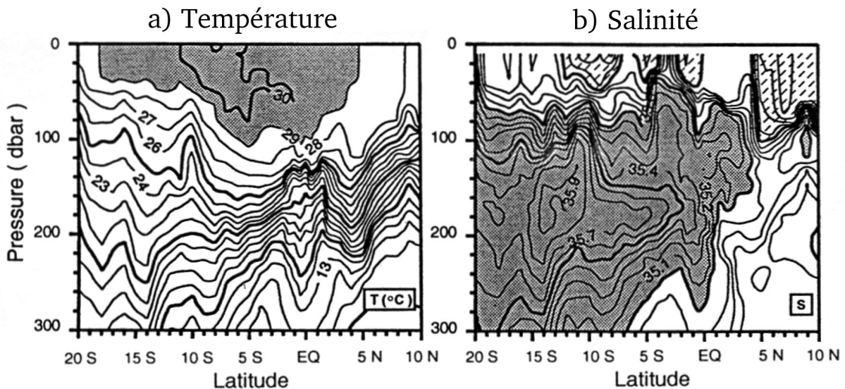
Figure 1.11 – Profils le long de 165^\circ\text{E} , en janvier 1986 (campagne SURTROPAC 05), correspondant à des conditions de référence ie. neutres : (a) température (°C, contours tous les 1^\circ\text{C} , températures supérieures à 29^\circ\text{C} grisées) et (b) salinité (psu, contours tous les 0.1 psu, salinités supérieures à 35.0 psu grisées, inférieures à 34.5 psu hachurées). D'après la figure 3 de Radenac et Rodier (1996) .
