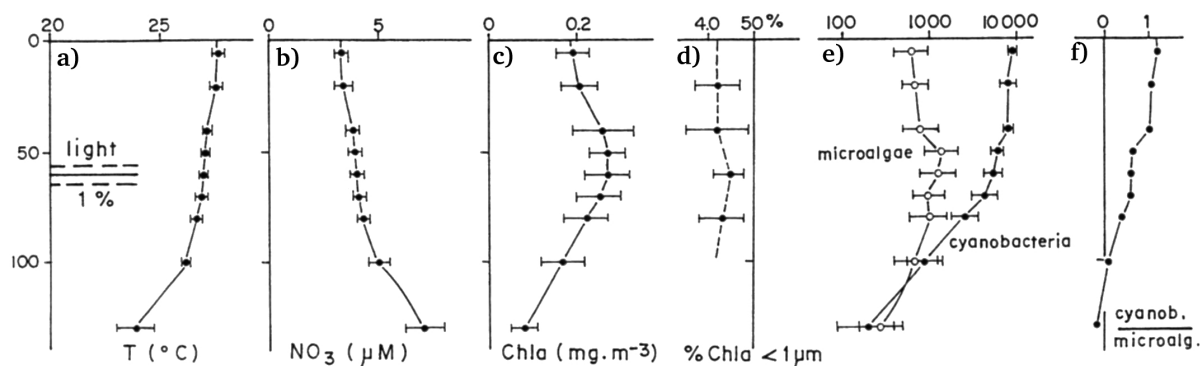
Figure 1.22 – Profils moyens de température (a), [NO_3] (b), [Chl a] (c), \%[Chl a] < 1\mu m (d), nombre de cyanobactéries et microalgues (échelle log, e), et ratio cyanobactéries/microalgues (f), obtenus à 0^\circ , 165^\circ E en avril 1988 pendant la campagne PROPPAC 2 (écosystème HNLC). La profondeur moyenne de la couche euphotique est indiquée (1% de la lumière incidente). D'après la figure 5 de Le Bouteiller et al. (1992) .
