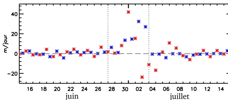
Figure 6.9 – Pompage d'Ekman calculé à partir des données journalières de rotationnel de tension de vent QuickSCAT, à 156°E-5°N, en \text{m jour}^{-1} (étoiles bleues) et variation de la profondeur de la thermocline repérée dans les données journalières TRITON par l'isotherme 24°C (étoiles rouges).
