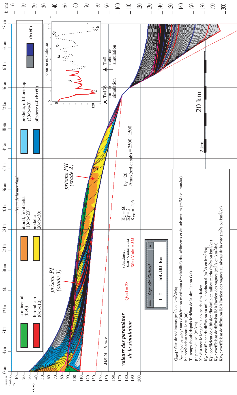
Figure VI-28 Géométrie induite par un cycle de variation eustatique sur 59 000 ans. Le flux de sédiments est constant et égal à 14 \text{ km}^3/ka . Le taux de subsidence est constant dans le temps mais différentiel dans l'espace ; il augmente vers le large de manière linéaire traduisant un basculement ou tilt de la marge. La valeur maximale à la dernière maille de simulation est de 525 \text{ m/ka} . La morphologie initiale est une droite de pente de 0,5 \text{ m/km} . La maille de simulation est de 0,5 \text{ km} . La courbe en encart correspond à la courbe de variation eustatique établie par Labeyrie, 1989 et appliquée à la simulation (sur les derniers 59^{\circ} \text{ ka} ). Les lignes temps sont représentées tous les mille ans (en noir). Les lignes rouges et bleues représentent respectivement les bas et les hauts niveaux relatifs de la courbe eustatique. Dans son ensemble, la série est progradante. Les dépôts ne s'empilent pas verticalement mais se déplacent latéralement au cours du cycle de l'amont vers l'aval. On distingue aisément sur la simulation les dépôts correspondant au stade isotopique 3 et 2.
