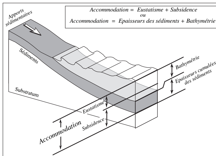
Figure VI-13 La double définition de l'accommodation (dessin de Granjeon, 1994).
