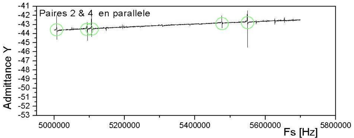
Paires 2&4 en Parallèle (fig. 3.14 . Réponse électrique. )
