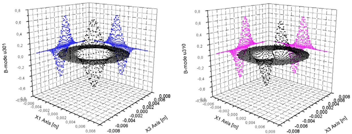
Figures 1.7, 1.8. Mode B, distribution des modes anharmoniques u_{301} et u_{310} respectivement.
