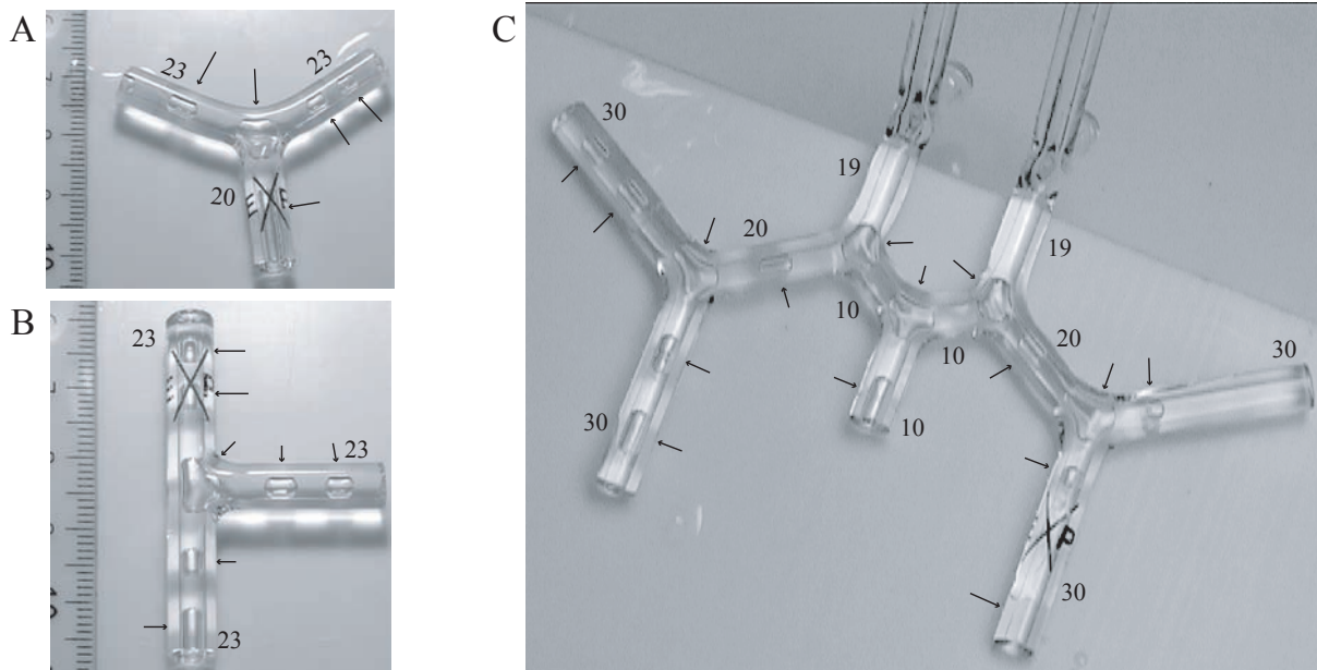
FIG. I.3.11 – Résultat de l'instabilité capillaire de l'huile silicone V1000 dans des embranchements de verre. Les nombres spécifient la longueur des tubes en millimètre, et les flèches soulignent la présence de bulles d'air. A/ Embranchement symétrique. Chaque branche 1,05 mm de rayon interne. B/ Embranchement asymétrique, avec les mêmes dimensions. C/ Embranchements multiples avec de plus faibles rapports d'aspect.
