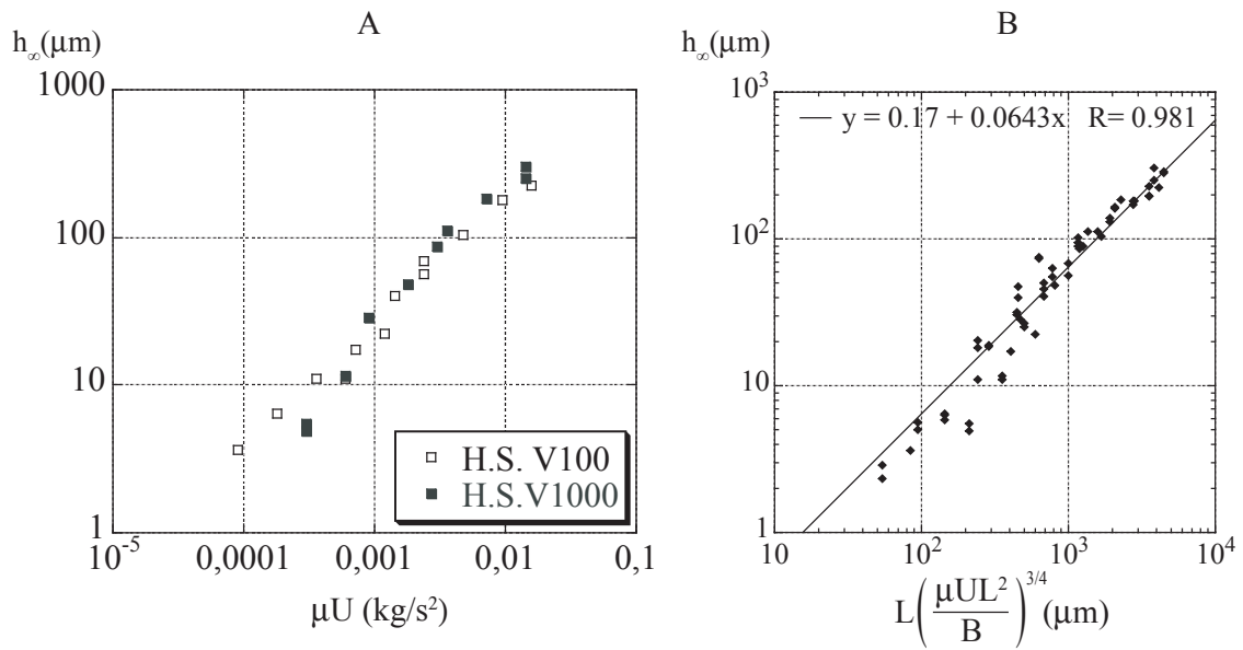
FIG. II.3.9 – Comparaison données-modèle. A / Vérification du scaling en \mu U . B / Vérification de la formule totale. La ligne représente la meilleure approximation linéaire h_\infty = 0,64 L V e^{3/4} .
