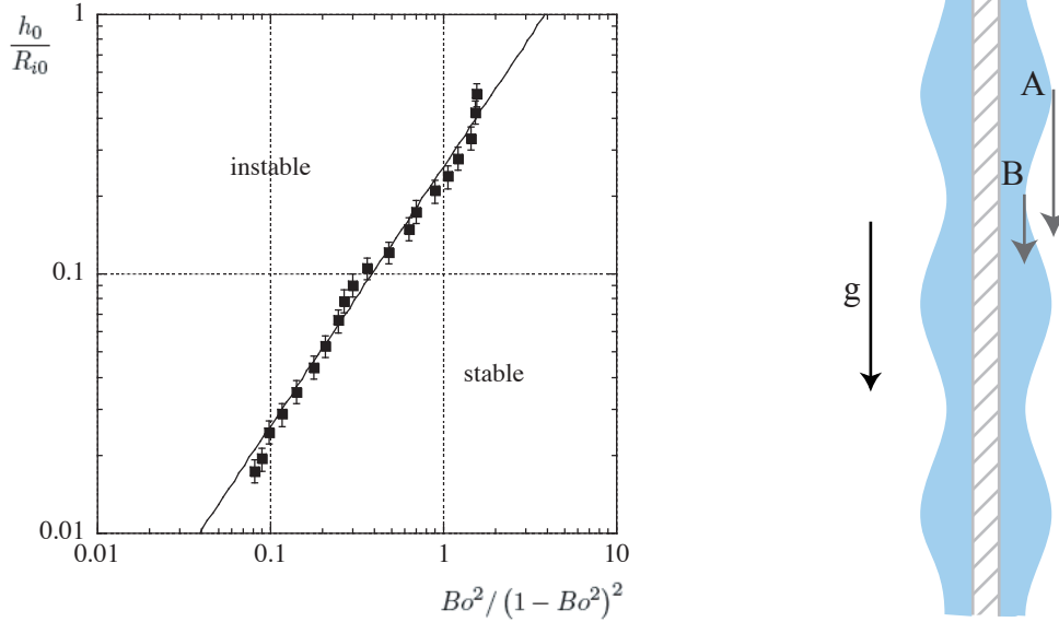
FIG. I.3.9 – (a) Transition entre une interface stable et une interface instable dans le plan \left[ \frac{h_0}{R_{i0}}; Bo^2 / (1 - Bo^2)^2 \right] : ■ données expérimentales. La ligne correspond à la meilleur approximation linéaire : \frac{h_0}{R_{i0}} = 0.26 Bo^2 / (1 - Bo^2)^2 . (b) Vue schématique pour le cas vertical. La vitesse de chute dépend de h^2 , donc le fluide placé au point A tombe plus vite que celui au point B.
