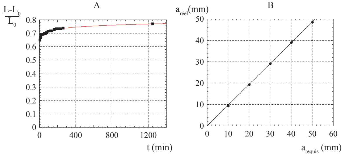
FIG. III.2.15 – A/ Vieillesse sous contrainte. La ligne représente le meilleur ajustement logarithmique y = 0,62 + 0,050 \log x ; R = 0,99201 . B/ Amplitude des mouvements du piston vus par la membrane en fonction de celle commandée au vérin. La droite représente la meilleure approximation proportionnelle y = 0,97x ; R = 0,99996 .
