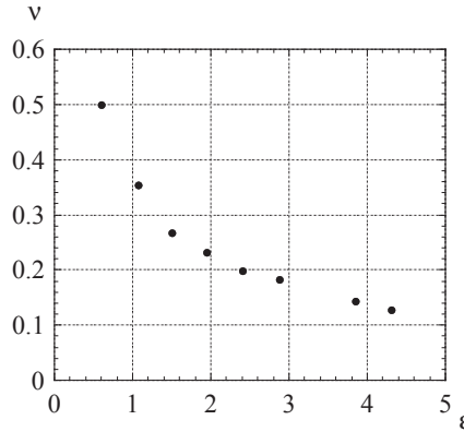
FIG. III.2.8 – Module de Poisson \nu = -\frac{L_0(b-b_0)}{b_0(L-L_0)} mesuré en fonction de l'élongation \epsilon = (L - L_0)/L_0 .
