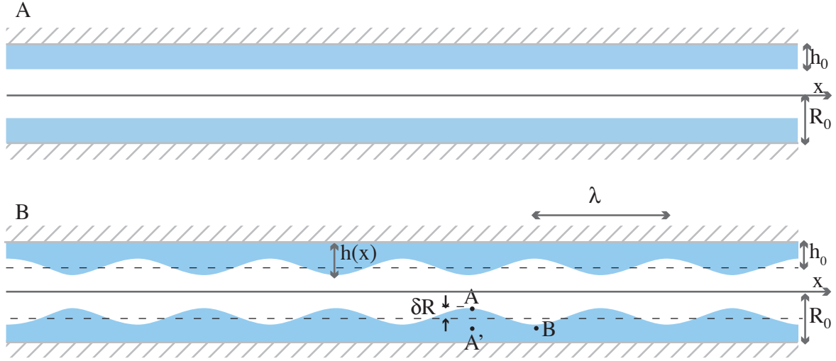
FIG. I.3.4 – Schéma de l'instabilité capillaire : A / Situation initiale pour un tube de rayon R_0 enduit d'une couche de liquide d'épaisseur h_0 . B / Situation perturbée h(x) = h_0(1 + \xi \cos(2\pi x/\lambda)) = h_0(1 + \xi \cos(kx)) .
