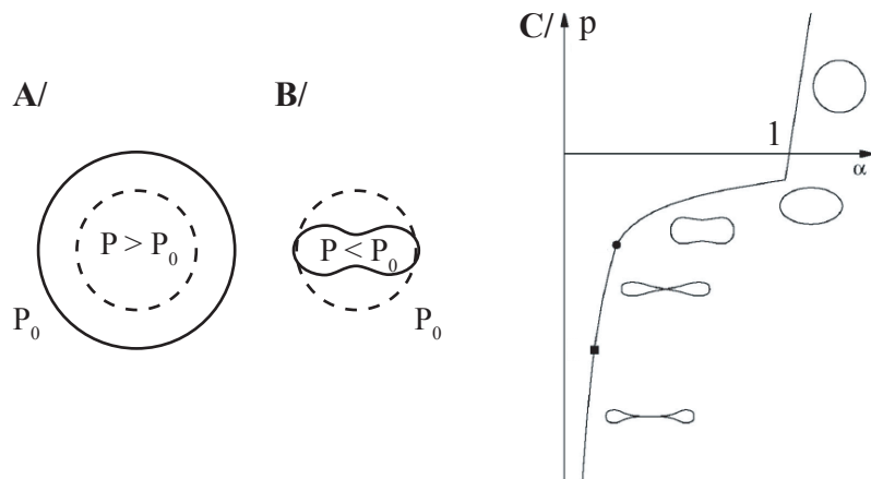
FIG. III.2.4 – Régimes de fonctionnement d'un tube élastique. A/ La pression interne est plus forte que la pression atmosphérique, et le tube est gonflé par rapport à son volume initial (en pointillés). B/ La pression transmurale P - P_0 est négative, le tube se déforme et flambe. C/ Report de la loi schématique d'évolution de la pression transmurale en fonction de \alpha = A/A_0 , tirée de [14].
