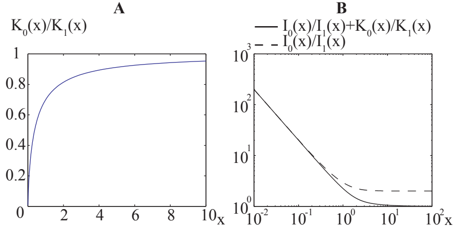
FIG. III.3.7 – Fonctions de Bessel intervenant dans la contribution du milieu extérieur. A/ K_0(x)/K_1(x) en fonction de x . B/ I_0(x)/(xI_1(x)) + K_0(x)/K_1(x)
