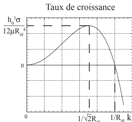
FIG. I.3.5 – Allure des variations du taux de croissance théorique \frac{h_0^3}{3\mu} k^2 \sigma \left( k^2 - \frac{1}{R_{i0}^2} \right) de \xi dans l'instabilité de Plateau-Rayleigh, en fonction du nombre d'onde k considéré.
