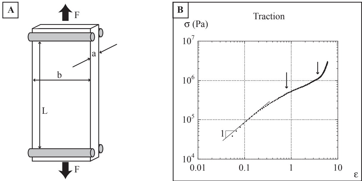
FIG. III.2.3 – Essais de traction sur le caoutchouc de la chambre à air. A/ Schéma de principe de l'expérience : on tire verticalement sur deux pinces qui enserrant les extrémités d'un morceau de caoutchouc de longueur, largeur et épaisseur initiales respectives L_0 , b_0 et a_0 . B/ Résultat pour un échantillon caractérisé par L_0 = 68 mm, a_0 = 0,7 mm et b_0 = 30 mm, étiré à une vitesse de 4 cm/min. On représente en abscisse l'élongation \epsilon = (L - L_0)/L_0 , et en ordonnée la contrainte \sigma = F/(a.b) \sim F/(a_0.b_0) . La droite a une pente 1, et les deux flèches matérialisent les bords du plateau caoutchoutique.
