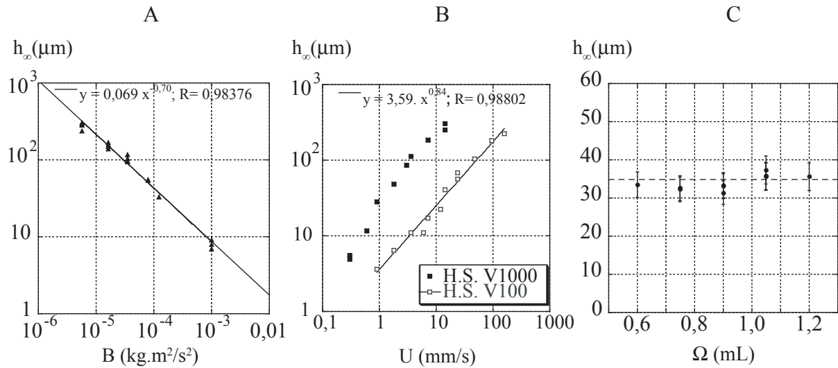
FIG. II.3.3 – A/ Effet de B sur h_\infty (huile silicone V100; U = 28,8 mm/s; b = 38 mm; L = 55,5 mm; Y_0/L = 0,42 ; \Omega = 800 \mu\text{L} ). B/ Effet de U et \mu sur h_\infty ( b = 38 mm; L = 35,5 mm; Y_0/L = 0,42 ; e = 100 \mu\text{m} ; \Omega = 800 \mu\text{L} ). C/ Effet de \Omega sur h_\infty (huile silicone V100; U = 12 mm/s; b = 38 mm; L = 45,5 mm; Y_0/L = 0,42 ; e = 100 \mu\text{m} ).
