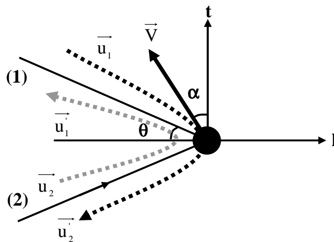
Figure II.6 : Représentation schématique de la trajectoire de la lumière lorsque les faisceaux (1) et (2) sont rétroinjectés par un dialogue optique entre les deux voies.
