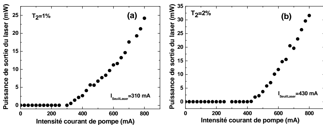
Figure I.27: Puissance émise par le laser LNA en fonction du courant d'alimentation de la diode laser de pompe (transmission du coupleur de sortie T_2 = 1\% (a) et T_2 = 2\% (b) pour une longueur de cavité de 12 mm).
