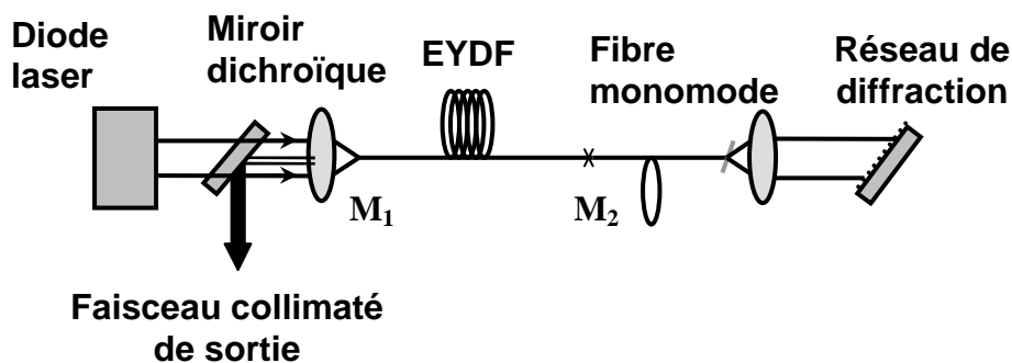
Figure I.23: Schéma de principe d'un laser à fibre double gaine codopée Er^{3+}/Yb^{3+} .
