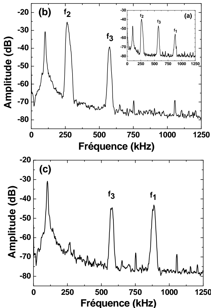
Figure II.10 : : Spectres RF du signal photodéteecté lorsque le disque est précisément placé au point de croisement des deux faisceaux de mesure : (a) sans isolateur optique sur (1) ou (2) , (b) avec isolateur sur (1) et (c) avec isolateur sur (2) .
