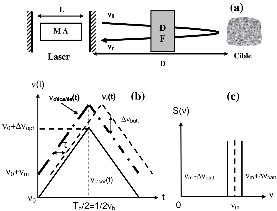
Figure III.2: a) Schéma de principe de la détection hétérodyne b) Evolution théorique de la fréquence optique en fonction du temps en détection hétérodyne: — Fréquence laser avant le dispositif de décalage; — • — Fréquence après le dispositif de décalage; ---- Fréquence réinjectée dans le laser après diffusion sur la cible et c) spectre de bruit de l'intensité émise par le laser .
