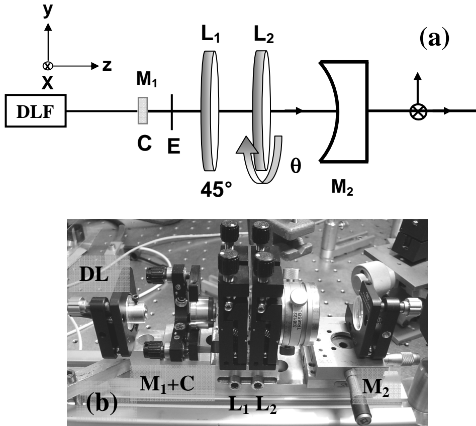
Figure IV.1. : (a) Représentation schématique du laser bi-fréquence verre phosphate dopé Yb:Er : avec DLF : Diode laser fibrée de pompage, C : Cristal, E : lame étalon, M : Miroir et L : Lames quart d'onde et (b) Photographie du dispositif réalisé.
