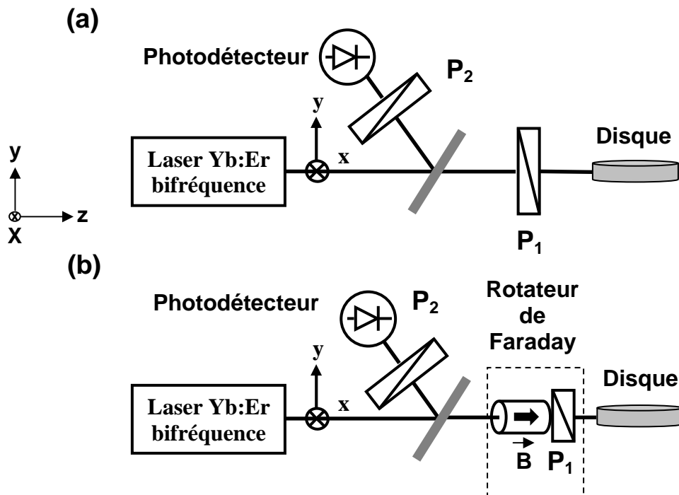
Figure IV.13 : Dispositif expérimental utilisé pour étudier le comportement d'un laser bi-fréquence soumis à un retour optique en fonction de l'état de polarisation rétroinjecté : (a) sélection de l'état de polarisation réinjecté par un simple polariseur P_1 et (b) système de rotateur à effet Faraday pour le couplage entre les deux modes propres.
