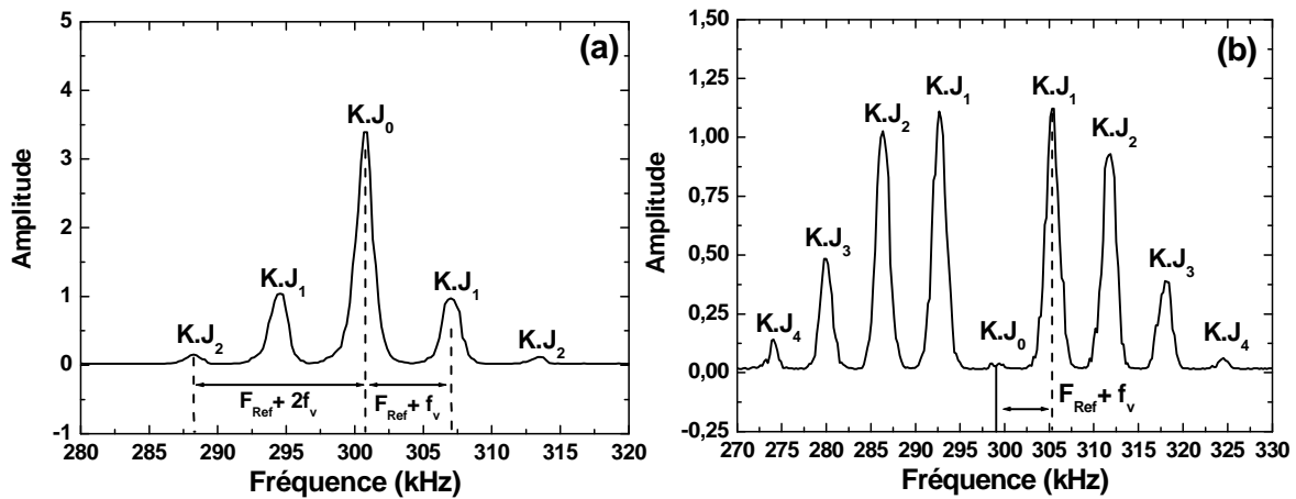
Figure II.29 : Spectres RF observés lorsque la membrane est soumise à un mouvement de vibration à la fréquence f_v=6,3 kHz : (a) Amplitude de la modulation appliquée au HP A_v=190 mV et (b) A_v=776 mV. Bande passante de l'analyseur BW=1 kHz.
