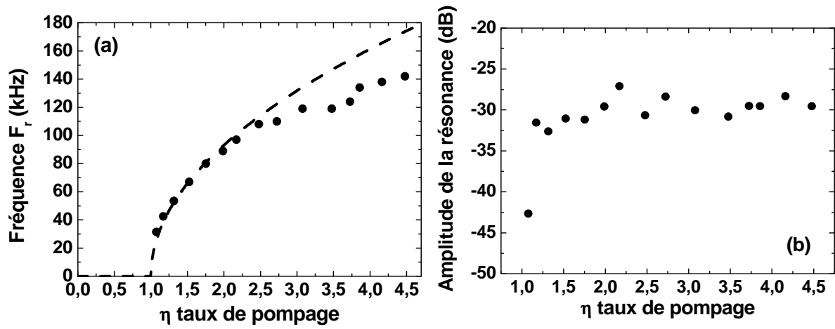
Figure 1.16: Evolution de la fréquence des oscillations de relaxations F_r (a) : ---- courbe théorique avec \gamma_c=3,8.10^8 et \beta_s=0,2 ; et de l'amplitude (b) de ces oscillations en fonction du taux de pompage \eta .
