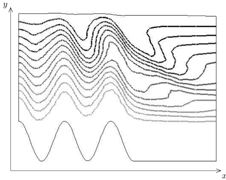
Fig. 6.24: Cas non isotherme. Douze isovalues de la plus grande valeur propre de \mathbf{a}^{(2)} , entre 1/3 et 1 du plus foncé au plus clair respectivement. L'échelle verticale est dilatée d'un facteur 30 par rapport à l'échelle horizontale.
