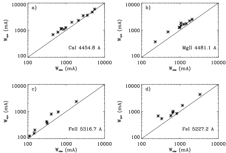
FIG. 7.15: Vérification des \log(gf) de certaines raies choisies : a) CaI 4454.8 Å ; b) MgII 4481.1 Å ; c) FeII 5316.7 Å ; d) 5227.2 Å. Pour chacune des ces raies blendées, nous avons identifié toutes les raies de la blende et nous avons tracé leur largeur équivalente mesurée sur un spectre solaire en fonction de la largeur équivalente synthétique. Le trait oblique représente la bissectrice du graphique.
