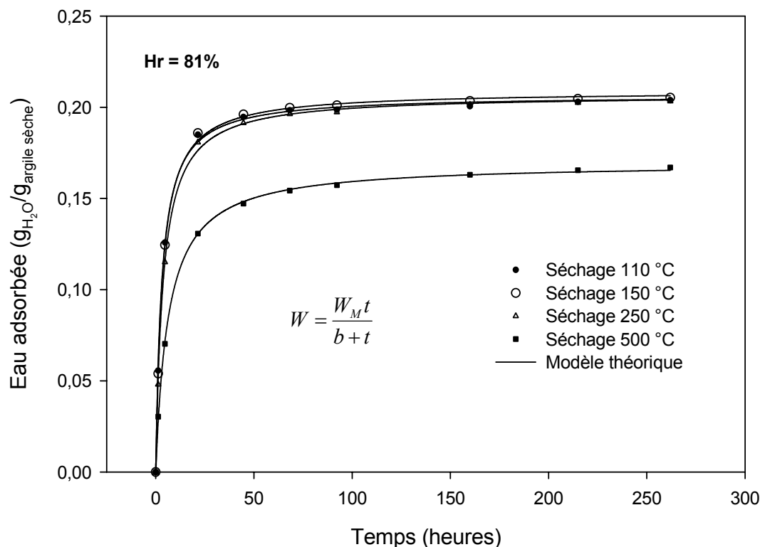
Figure 4.8 Données expérimentales et courbes de lissage. Influence de la température de séchage sur la cinétique d'adsorption d'eau de la bentonite MX80 brute (Hr : 81%). Modèle hyperbolique.
