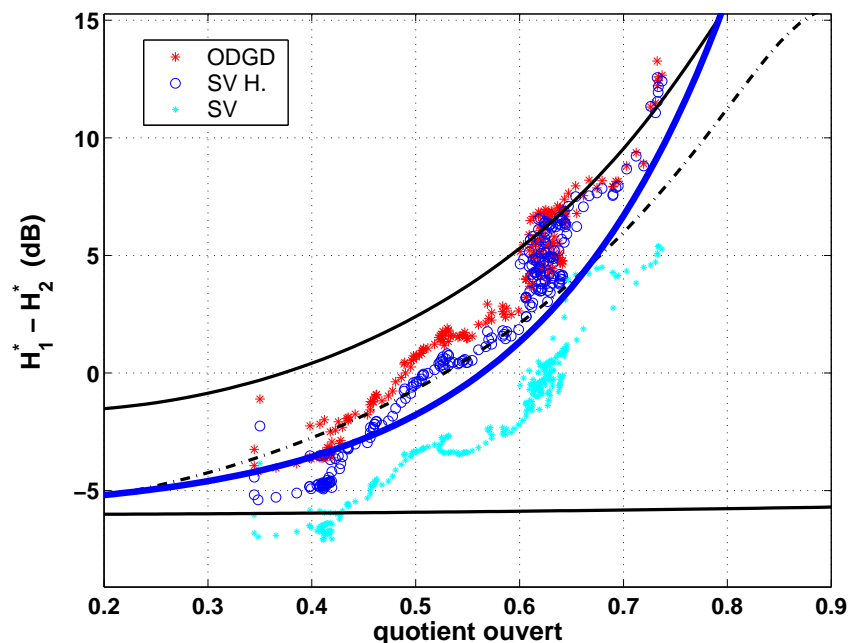
FIG. 4.15 – Mesures de (H_1 - H_2) en fonction de O_q dans le cas d'une voyelle émise de façon relâchée à pressée. Les bornes du domaine théorique de variation de (H_1 - H_2) ont été représentées en trait plein : la limite inférieure correspond à \alpha_m = 0.98 et Q_a = 0 et la limite supérieure à \alpha_m = 0.6 et Q_a = 0.2 . La courbe en pointillés correspond à la limite du domaine théorique pour Q_a = 0 ( \alpha_m = 0.6 ). La courbe en trait plein gras correspond à la relation empirique proposée par Fant [69, 70] . ODGD : mesures effectuées sur le signal ODGD obtenu par filtrage inverse, SV H. : mesures effectuées sur le signal voisé avec application d'un terme correctif (méthode de Hanson [97, 98] ), SV : mesures effectuées sur le signal voisé sans correction formantique.
