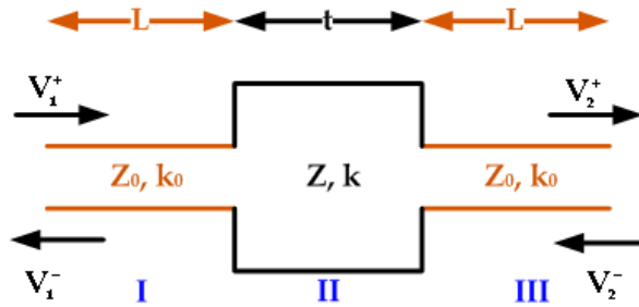
Fig. II-9: représentation des impédances et des constantes de propagation en fonction des différents milieux
