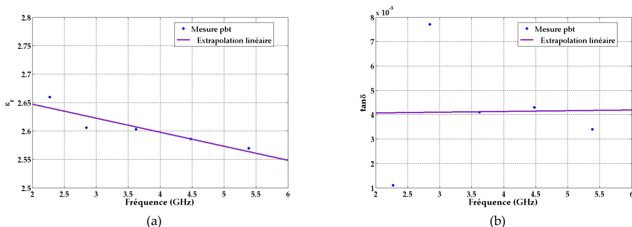
Fig. IV-3: permittivités et facteurs de pertes diélectriques, suite aux mesures et extrapolés, entre 2 et 6 GHz, pour le cas du PBT
