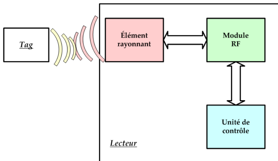
Fig. I-3: lecteur communiquant avec le tag
