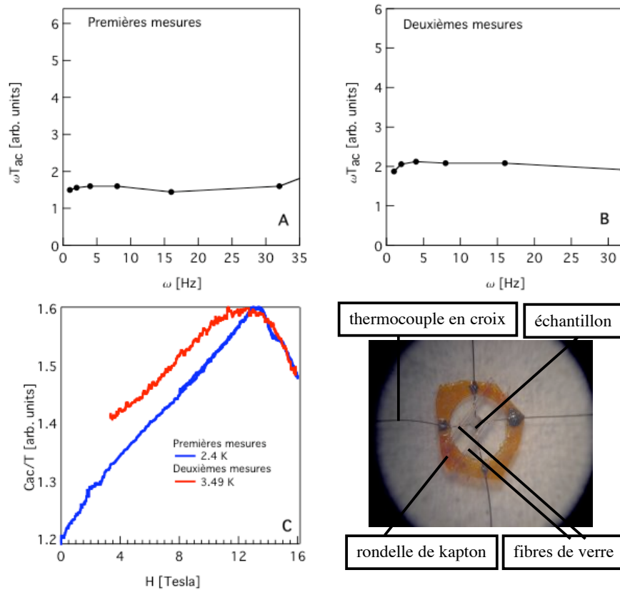
FIG. 4.10 – Comparaison des première et deuxième séries de mesures de chaleur spécifique alternative. Panel A et B Caractéristiques en fréquences du montage de l'échantillon. Cette caractéristique permet de tester la qualité du couplage thermique entre l'échantillon et le thermocouple. Le plateau de cette caractéristique indique d'une part que le couplage thermique est bon et d'autre part donne la plage de fréquences avec lesquelles on peut mesurer la chaleur spécifique (pour plus de détails sur la signification de ces caractéristiques en fréquence le lecteur pourra se reporter au chapitre techniques expérimentales). Panel C Dépendance de la chaleur spécifique divisée par la température en fonction du champ appliqué selon l'axe \vec{b} des échantillons. Une mesure de chaque série est présentée : ces mesures sont similaires. Le point d'inflexion des courbes est aux environs de 13 Tesla. Photo Photo du montage utilisé. Le thermocouple est constitué d'un fil de chromel et d'un fil de constantan. Il est collé sur une rondelle de kapton avec de la stycast noire. L'échantillon est collé au vernis General Electric sur le thermocouple. Pour la deuxième série de mesure des fibres de verre ont été ajoutées pour rigidifier le système. Ces fibres sont collées au thermocouple en quatre points et à la rondelle de kapton en quatre points.
