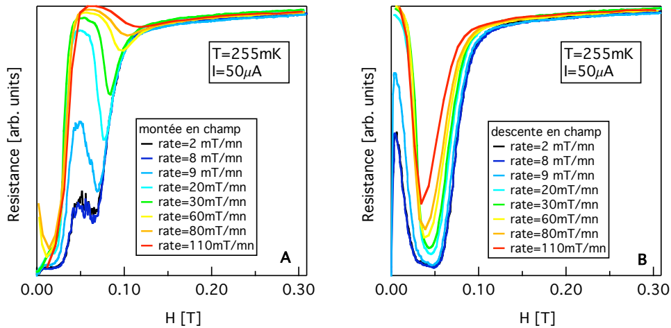
FIG. 3.9 – Dépendance de la résistance en fonction du champ appliqué selon l’axe c pour différentes vitesses de rampe en champ. A T=255 mK, pour I=50\mu A , nous avons utilisé différentes vitesses de rampe en champ. Panel A Montée en champ. Panel B Descente en champ. Le comportement singulier de la résistance en fonction du champ appliqué selon l’axe c est renforcé pour des vitesses de rampe en champ de plus en plus grandes.
