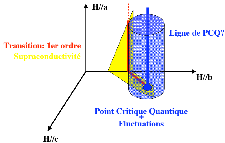
FIG. 6.9 – Diagramme de phase schématisique de la supraconductivité à hauts champs et de la transition métamagnétique. Comportements schématisiques de la supraconductivité à hauts champs et de la transition métamagnétique en fonction des champs appliqués selon les trois directions cristallographiques \vec{a} , \vec{b} et \vec{c} . La ligne rouge symbolise la transition métamagnétique du premier ordre. Cette ligne se termine par un point critique quantique : rond bleu. Comme l'augmentation du champ magnétique appliqué selon l'axe \vec{a} n'influence pas la position de la transition métamagnétique selon \vec{b} , nous pouvons supposer qu'il en est de même pour la position du point critique quantique : il y aurait une ligne de points critiques quantiques, symbolisée par une ligne bleue sur la figure. Le cylindre bleu transparent représente les fluctuations quantiques émergeant de ces points critiques quantiques. La supraconductivité induite sous champ, région en jaune sur la figure, englobe la transition du premier ordre.
