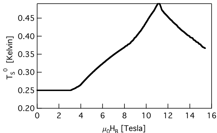
FIG. 6.13 – Dépendance de la température supraconductrice maximum en fonction du champ appliqué selon l'axe b . A champ nul on trouve une température critique de 230 mK. Les mesures donnent une température critique de 270 mK.
