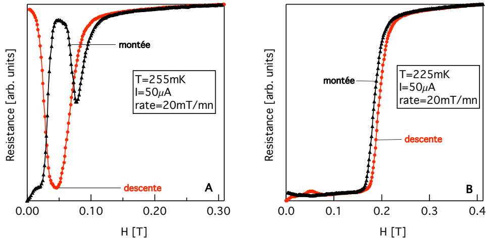
FIG. 3.7 – Dépendance de la résistance en fonction du champ appliqué selon l'axe \vec{c} . Les mesures des deux panels ont été faites pour un courant de 50 \mu\text{A} et pour une vitesse de rampe en champ de 20 \text{ mT/mn} . Panel A Mesure faite à 255 mK. La résistance a un comportement inhabituel au environ de la transition supraconductrice. A la montée on observe un pic à la transition supraconductrice pour un champ de 50 mT. A la descente la résistance augmente quand le champ diminue pour des champs inférieurs à 50 mT. Panel B Mesure faite à 225 mK. Le comportement de la résistance est redevenue classique : on observe uniquement la transition supraconductrice.
