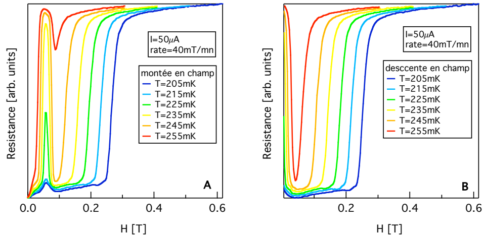
FIG. 3.10 – Dépendance de la résistance en fonction du champ appliqué selon l'axe c pour différentes températures. Pour I = 50 \mu A et une vitesse de rampe en champ de 40 \text{ mT/mn} nous avons mesuré la résistance pour différentes températures. Panel A Montée en champ. Panel B Descente en champ. Le comportement singulier de la résistance en fonction du champ appliqué selon l'axe c est renforcé pour les températures les plus élevées.
