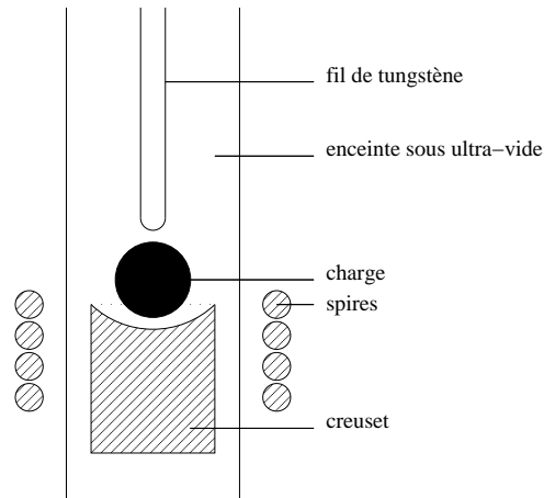
FIG. 2.1 – Principe du tirage Czochralski. La charge liquide, composée des éléments composant le cristal, est en lévitation au centre du creuset (en cuivre). Cette charge a été fondue par induction grâce au champ magnétique créé par les spires (en cuivre). Un cristal est tiré à partir de la charge liquide avec un fil de tungstène en rotation.
