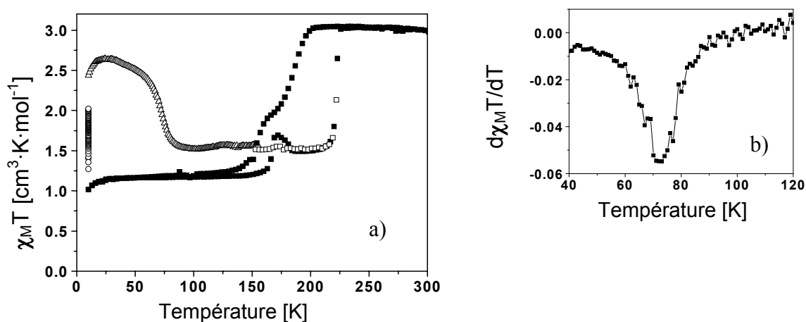
Figure IV.17 - a) T(LIESST) pour le complexe [\text{Fe}(\text{L}_{222}(\text{N}_3\text{O}_2))(\text{CN})_2]\cdot\text{D}_2\text{O} relatif à la première descente en température. b) Valeur du T(LIESST) autour de 72 K.
