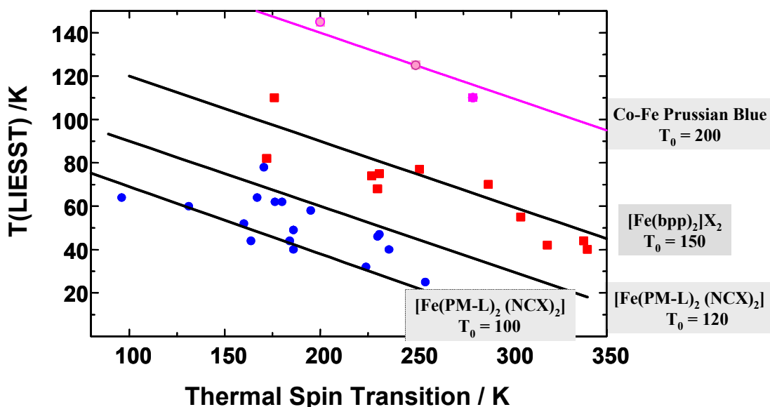
Figure I.9 - Représentation T(\text{LIESST}) vs T_{1/2} de plus de 60 composés à TS.
