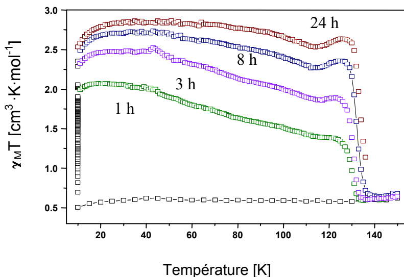
Figure III.18 Différent T(\text{LIESST}) rapportés en fonction du temps d'irradiations [\text{Fe}(\text{L}_{222}(\text{N}_3\text{O}_2))(\text{CN})_2] \cdot \text{H}_2\text{O} .
