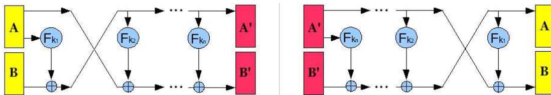
FIG. 1.5 – Cryptage et décryptage du réseaux de Feistel
