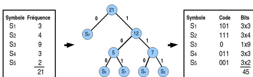
FIG. 3.1 – Algorithme d'Huffman.
