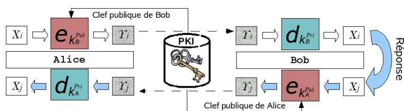
FIG. 1.1 – Principe de chiffrement asymétrique
