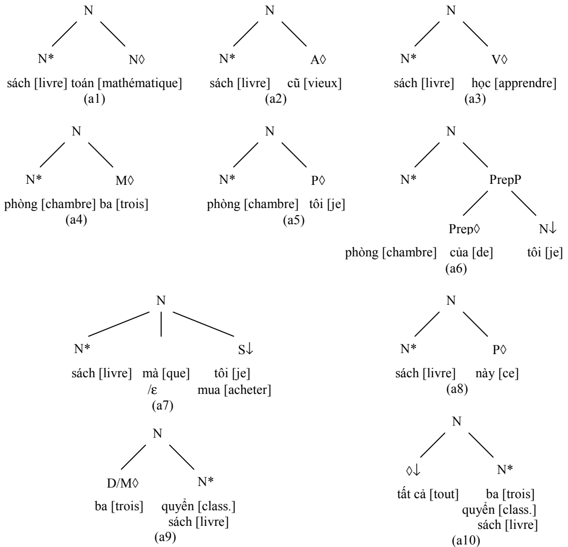
Figure 4-12 Arbres auxiliaires produisant les modifieurs du groupe nominal
