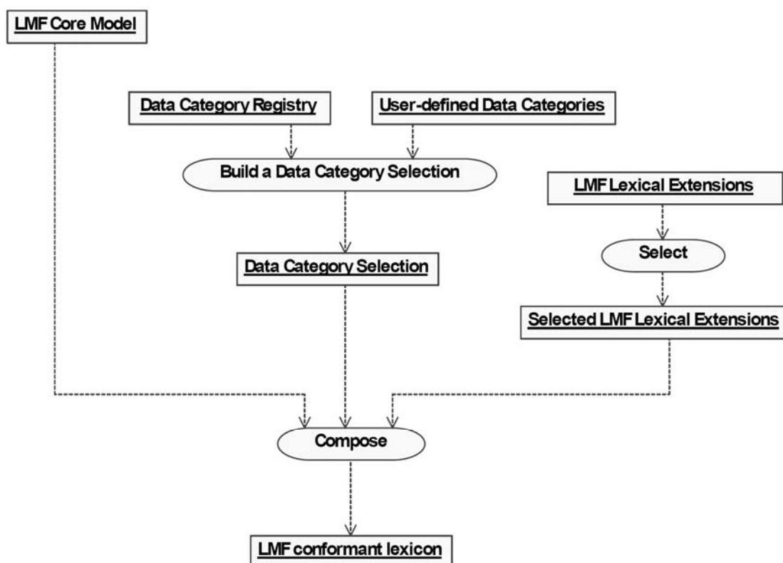
Figure 3-3 Processus d'utilisation de LMF ([ISO 05b])
