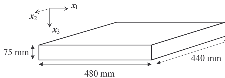
Figure 5.5. Plaque de micro-béton à propriétés continûment variables.
