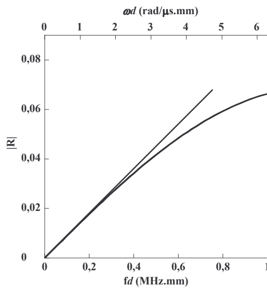
Figure 5.4. Tracé de la pente à l'origine du module du coefficient de réflexion tracé en fonction du produit fréquence-épaisseur.
