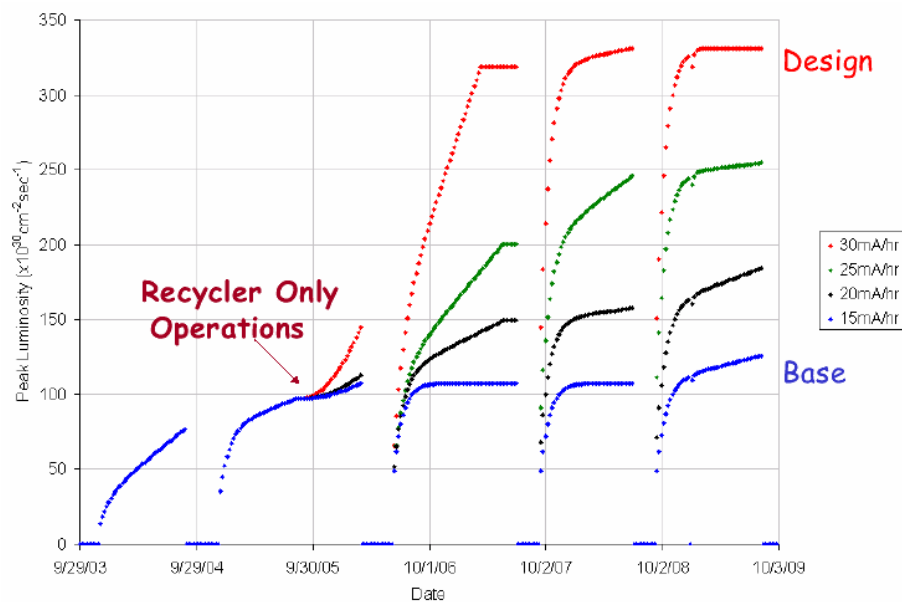
FIG. 4.28 – Projection sur l'évolution de la luminosité instantanée délivrée par le Tevatron pour diverses hypothèses de taux de stockage des antiprotons. Le mode de fonctionnement recycler only operation correspond à la mise en fonctionnement du refroidissement des antiprotons par un faisceau d'électrons.
