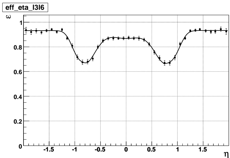
FIG. 6.5 – Efficacité de déclenchement du détecteur à muons au L3 pour un muon en fonction de sa pseudo-rapidité.
