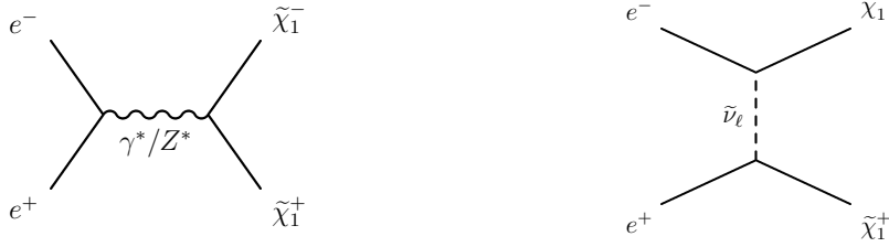
FIG. 2.1 – Diagrammes de production de paires \tilde{\chi}_1^+ \tilde{\chi}_1^- à LEP.
