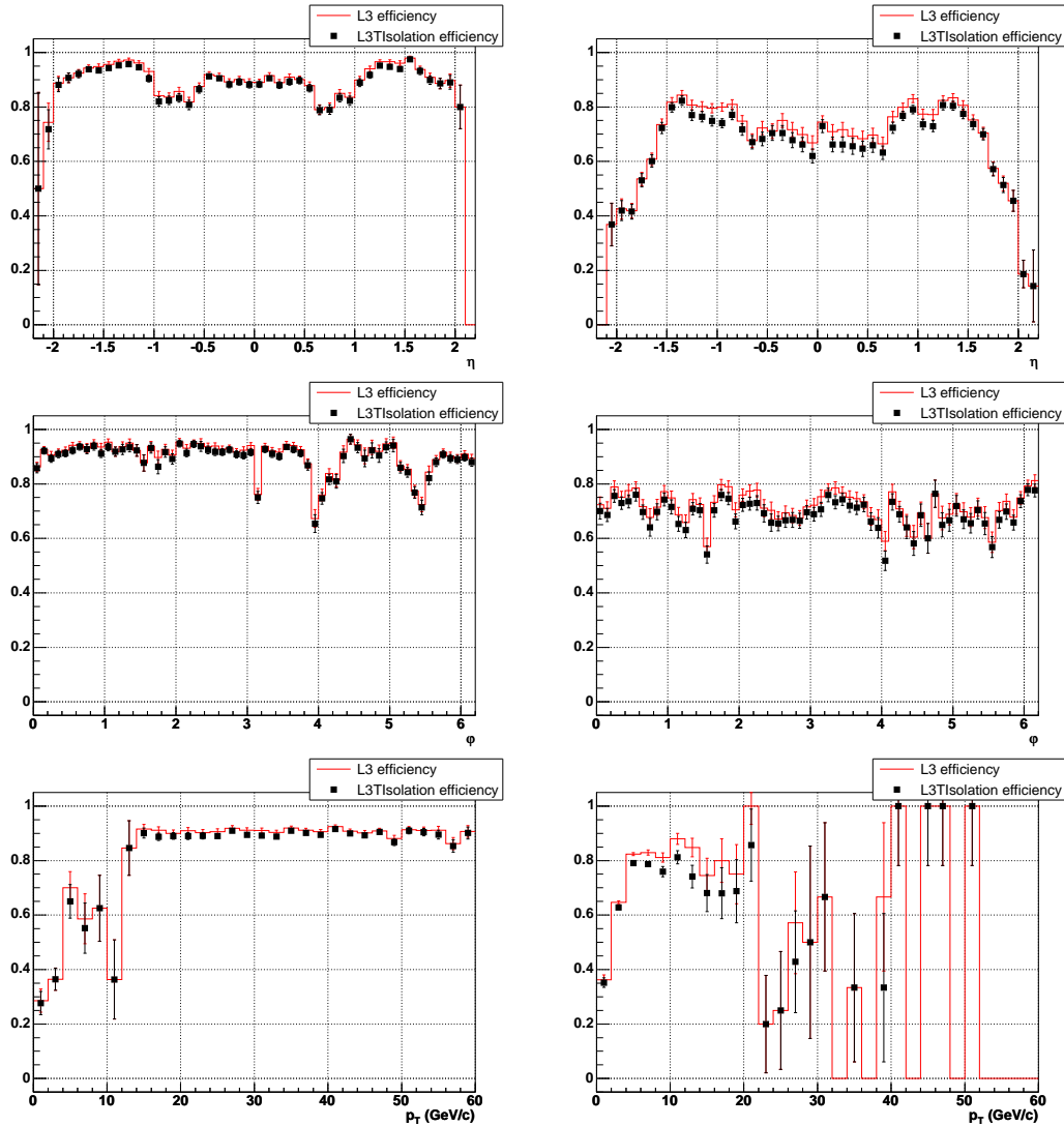
FIG. 5.7 – Efficacités en considérant les lots Z (gauche) et J/\psi (droite). De haut en bas sont présentées les efficacités en fonction de \eta , \varphi et p_T du muon reco. L'efficacité de l'outil MUON_CM est illustrée par une ligne rouge est celle correspondant à l'outil ISO_MUON par des carrés noirs. Des pertes d'efficacité de 1.3% et 3.9% sont respectivement observées pour les lots Z et J/\psi en appliquant le critère E_T^{halo} < 4 GeV.
