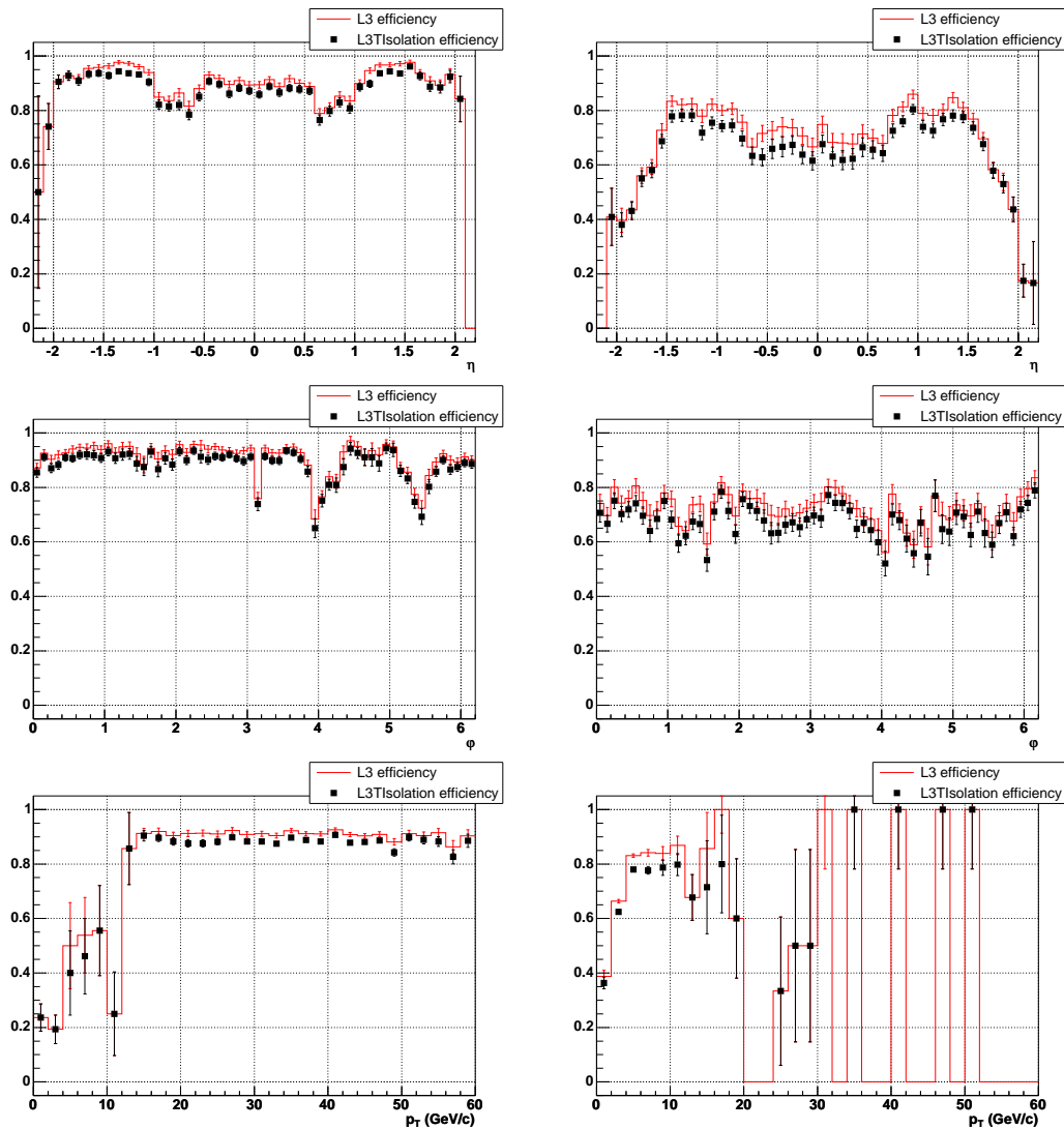
FIG. 5.10 – Efficacités en considérant les lots Z (gauche) et J/ \psi (droite). De haut en bas sont présentées les efficacités en fonction de \eta , \varphi et p_T du muon reco. L'efficacité de l'outil MUON_CM est illustrée par une ligne rouge est celle correspondant à l'outil ISO_MUON par des carrés noirs. Des pertes d'efficacité de 2.8% et 6.2% sont respectivement observées pour les lots Z et J/ \psi en appliquant les critères E_T^{halo} < 2.5 GeV et p_T^{halo} < 2.5 GeV/c.
