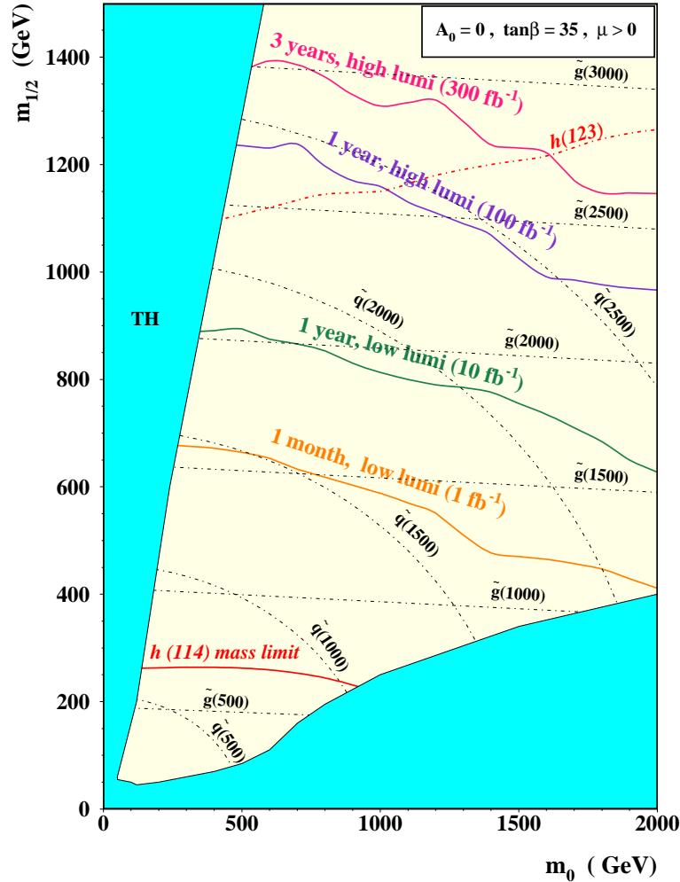
FIG. 7.18 – Potentiel de découverte à 5\sigma de l'expérience CMS dans le plan m_0 - m_{1/2} pour un scénario mSUGRA où A_0 = 0 , \mu > 0 et \tan\beta = 35 . Les lignes pleines représentent les limites obtenues pour diverses luminosités intégrées. La zone pleine est exclue théoriquement [94].
