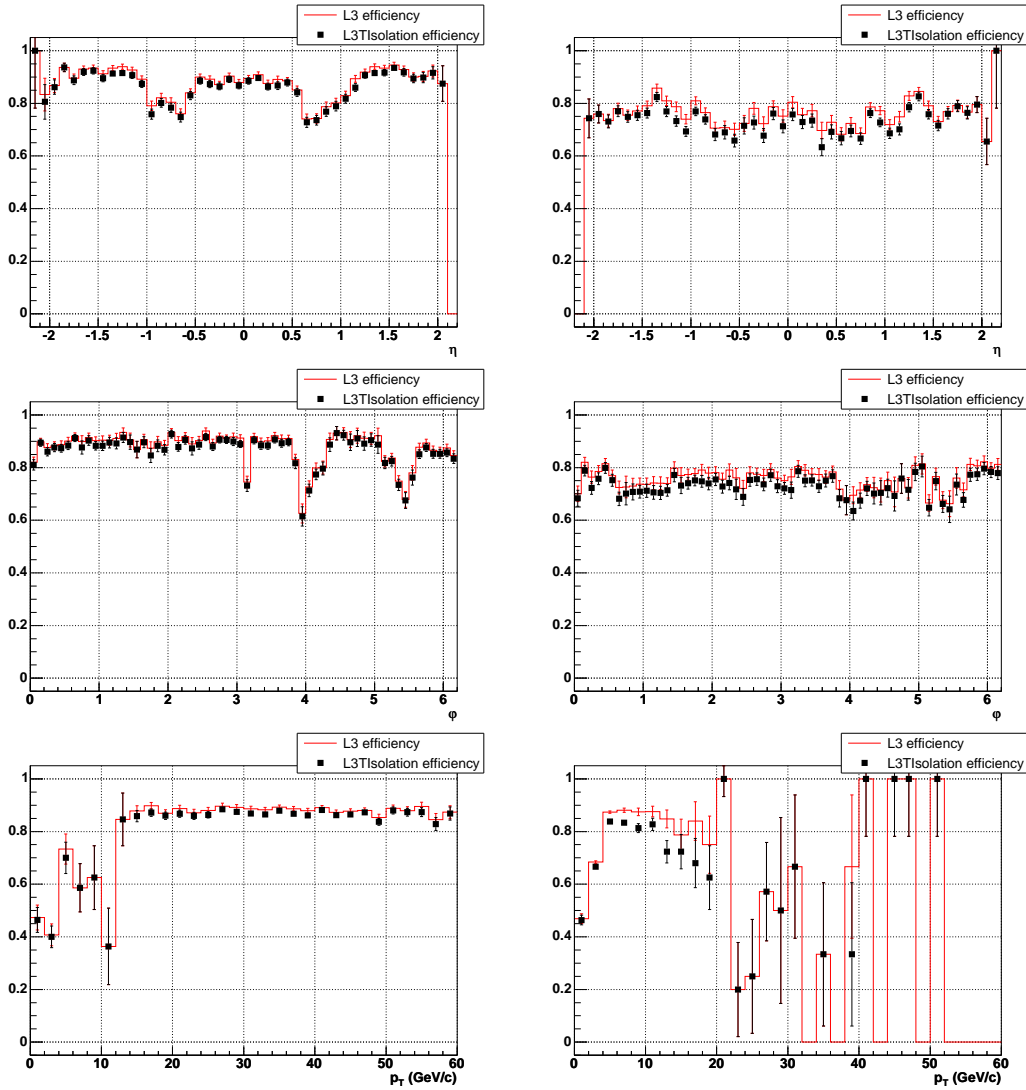
FIG. 5.12 – Efficacités en considérant les lots Z (gauche) et J/ \psi (droite). De haut en bas sont présentées les efficacités en fonction de \eta , \varphi et p_T du muon reco. L'efficacité de l'outil Muon est illustrée par une ligne rouge est celle correspondant à l'outil ISO_MUON par des carrés noirs. Des pertes d'efficacité de 1.7% et 3.8% sont respectivement observées pour les lots Z et J/ \psi en appliquant le critère E_T^{halo} < 4 GeV.
