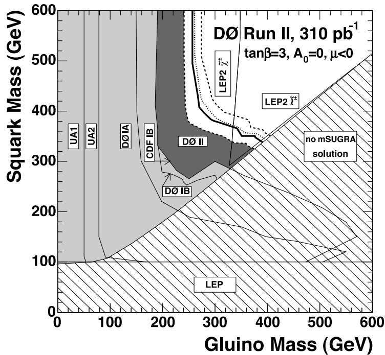
FIG. 2.5 – Exclusions dans le plan (m_{\tilde{q}}, m_{\tilde{g}}) obtenues à UA1, UA2, LEP et au Tevatron. Les traits épais plein et pointillé correspondent respectivement aux limites observée et attendue à 95% CL. La zone comprise entre les tirets correspond aux incertitudes sur les fonctions de densité partonique et à une variation d'un facteur 2 sur l'échelle de factorisation. La zone hachurée ne correspondant à aucune solution de type mSUGRA est exclue. Cette figure est extraite de la référence [34].
