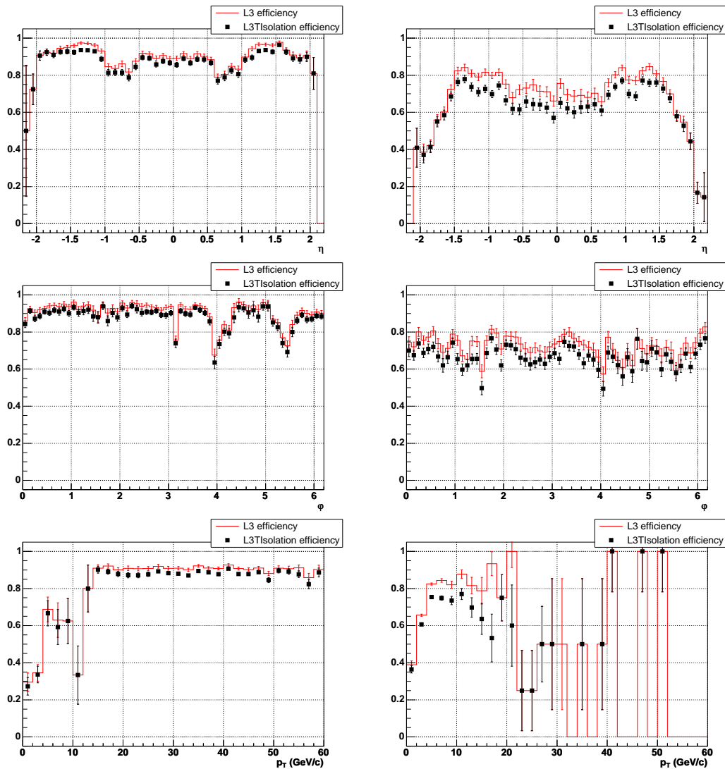
FIG. 5.8 – Efficacités en considérant les lots Z (gauche) et J/ \psi (droite). De haut en bas sont présentées les efficacités en fonction de \eta , \varphi et p_T du muon reco. L'efficacité de l'outil MUON_CM est illustrée par une ligne rouge est celle correspondant à l'outil ISO_MUON par des carrés noirs. Des pertes d'efficacité de 2.9% et 8.6% sont respectivement observées pour les lots Z et J/ \psi en appliquant le critère E_T^{halo} < 2.5 GeV.
