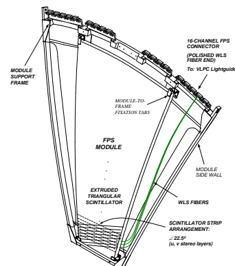
FIG. 4.10 – Module du FPS. Nous distinguons la partie centrale instrumentée de plans de fibres scintillantes formant un angle de 22.5^\circ et les parties latérales servant de support. Des fibres de décalage sont représentées dans la partie latérale.
