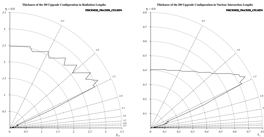
FIG. 4.12 – Épaisseur exprimée en unité de X_0 (à gauche) et \lambda_i (à droite) traversée par les particules avant d'atteindre le FPS en fonction de leur pseudo-rapacité. Les particules sont supposées produites au centre du détecteur.
