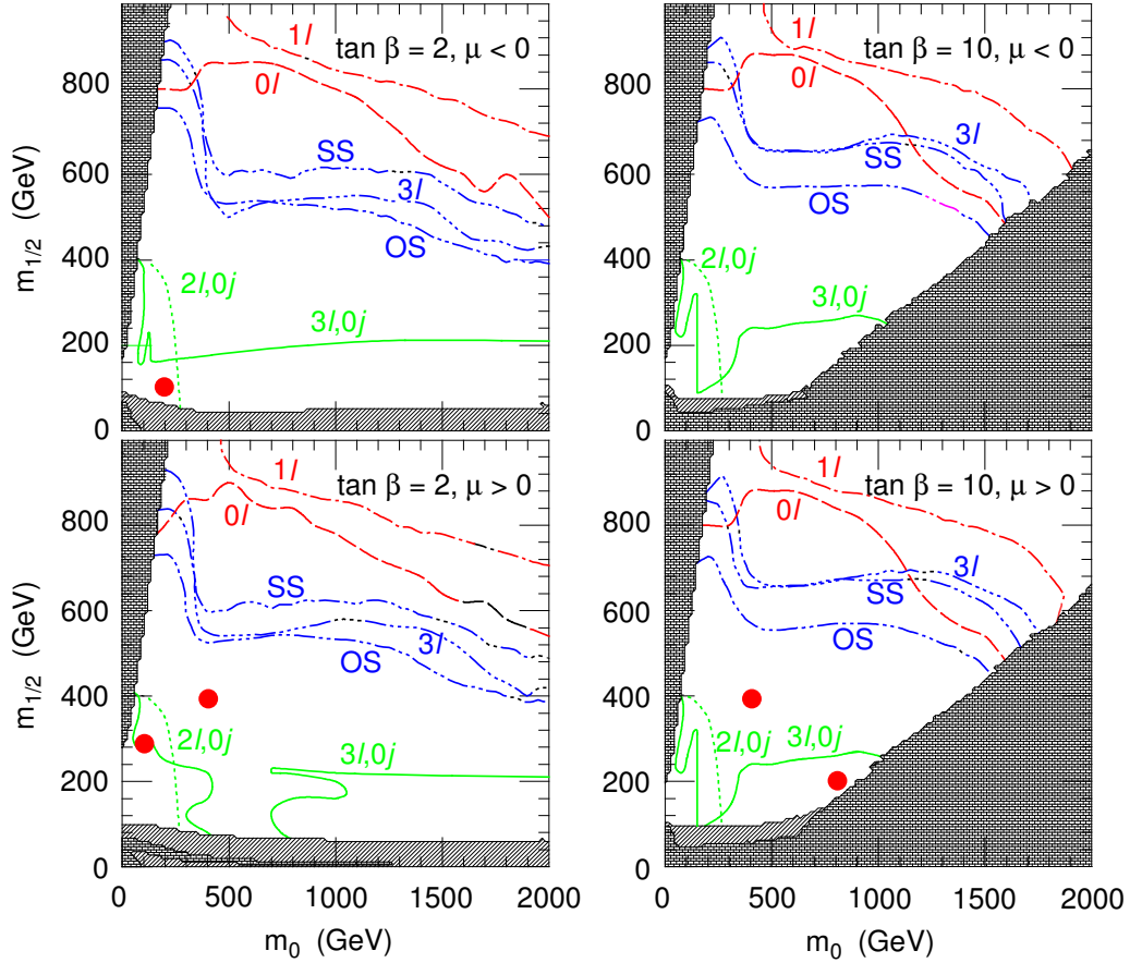
FIG. 7.17 – Potentiel de découverte de l'expérience ATLAS dans le plan m_0 - m_{1/2} pour différentes valeurs de \tan\beta et du signe de \mu , la valeur du paramètre A_0 étant fixé à 0. Chaque courbe représente la sensibilité pour un canal donné. 0l : jets + \cancel{E}_T sans lepton, 1l : jets + \cancel{E}_T + 1\ell , SS : dilepton de même signe, OS : dilepton de signes opposés, 3l : triplepton, 3l,0j : triplepton avec veto sur les jets et 2l,0j : dilepton avec veto sur les jets. La zone en briques à basses m_0 est exclue pour que la LSP soit le \tilde{\chi}_1^0 et non le \tilde{\tau}_1 . La zone en briques à grandes m_0 est elle exclue pour conserver la brisure de la symétrie électrofaible. La zone hachurée est exclue par les résultats de précédentes expériences. Les points représentent cinq points de référence mSUGRA [95].
