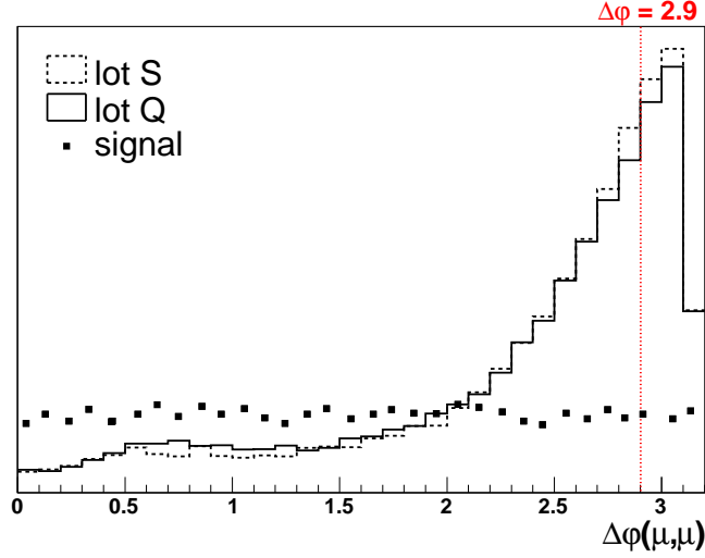
FIG. 7.1 – Distributions de l'écart angulaire en \varphi entre les deux muons de même signe pour le lot \mathcal{Q} et le signal. Le signal présente une distribution uniforme contrairement au lot \mathcal{Q} . La région \Delta\varphi(\mu,\mu) \geq 2.9 est choisie pour normaliser le lot \mathcal{Q} au lot \mathcal{S} . Seuls les événements vérifiant la présélection sont considérés.
