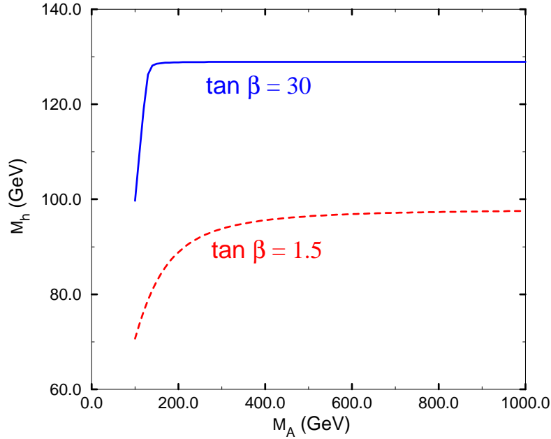
FIG. 1.7 – Masse du boson de Higgs le plus léger en fonction de la masse de A^0 et pour deux valeurs de \tan \beta . Les particules sont supposées ici avoir une masse inférieure à 1 TeV/ c^2 . Cette figure est extraite de la référence [9].
