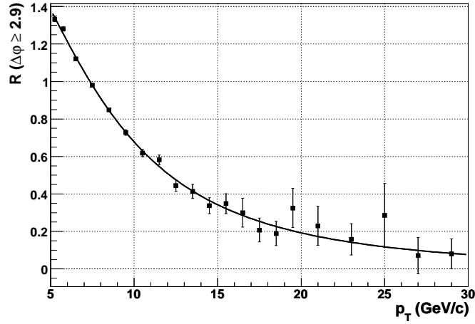
FIG. 7.2 – Fonction de pondération obtenue en normalisant la distribution en impulsion transverse du lot \mathcal{Q} à celle du lot \mathcal{S} pour les événements tels que \Delta\varphi(\mu,\mu) \geq 2.9 .
