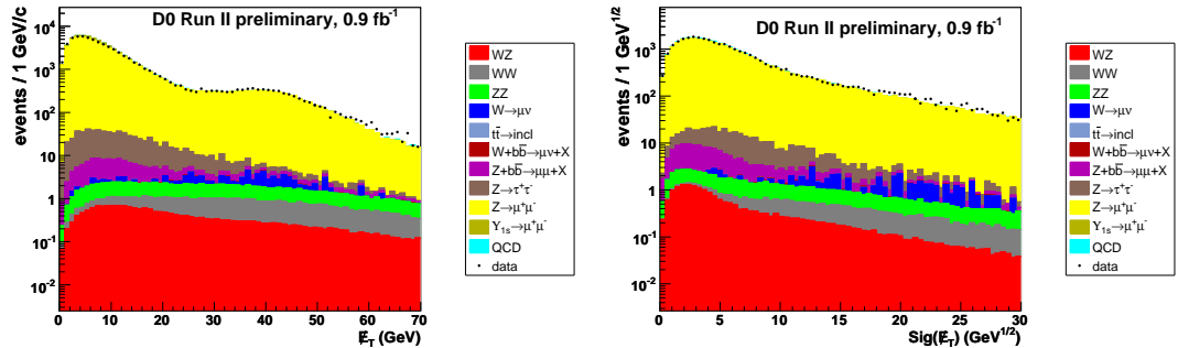
FIG. 7.6 – Distributions de l'énergie transverse manquante (à gauche) et de \text{Sig}(E_T) (à droite) pour les données et les différents bruits de fond considérés. Aucun critère n'est appliqué sur la charge des muons et la coupure sur l'impulsion transverse est renforcée à 8 GeV/c.
