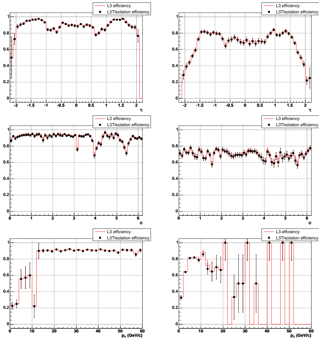
FIG. 5.9 – Efficacités en considérant les lots Z (gauche) et J/\psi (droite). De haut en bas sont présentées les efficacités en fonction de \eta , \varphi et p_T du muon reco. L'efficacité de l'outil MUON_CM est illustrée par une ligne rouge est celle correspondant à l'outil ISO_MUON par des carrés noirs. Aucune perte d'efficacité significative n'est observée pour le critère p_T^{halo} < 2.5 GeV/c.
