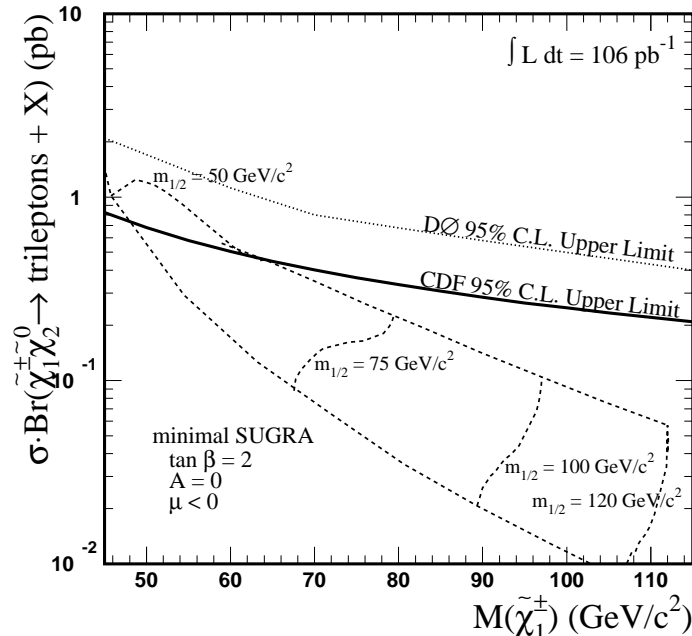
FIG. 2.9 – Limites obtenues sur \sigma(pp \rightarrow \tilde{\chi}_1^\pm \tilde{\chi}_2^0) \times BR(3\ell) par DØ et CDF durant la phase I du Tevatron. Les courbes en pointillés en bas et en haut correspondent respectivement à un choix pour m_0 de 100 et 2500 \text{GeV}/c^2 . Le paramètre m_{1/2} varie de 50 à 120 \text{GeV}/c^2 .
