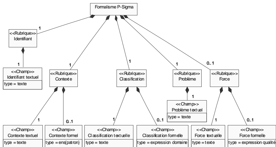
Figure 9.1. Modèle de la partie « Interface » du formalisme P-Sigma
