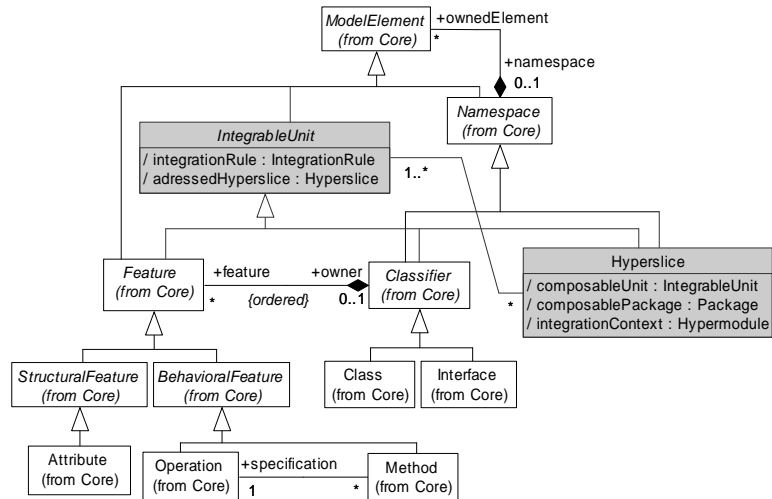
Figure 4.13. HyperJ/UML — Syntaxe abstraite des unités intégrables
