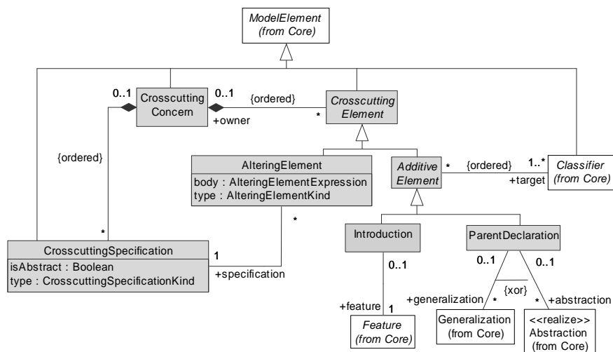
Figure 4.21. Aspect/UML — Syntaxe abstraite des éléments d'entrecroisement
