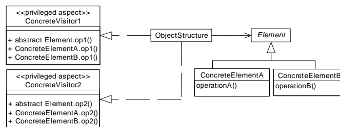
Figure 3.3. Solution en AspectJ du patron Visiteur
