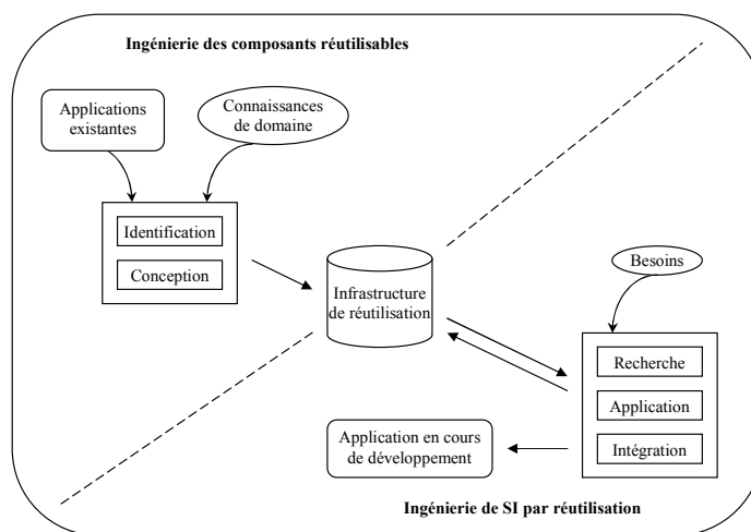
Figure 1.1. Ingénierie pour la réutilisation et ingénierie par réutilisation de composants [Cauvet et al., 01]
