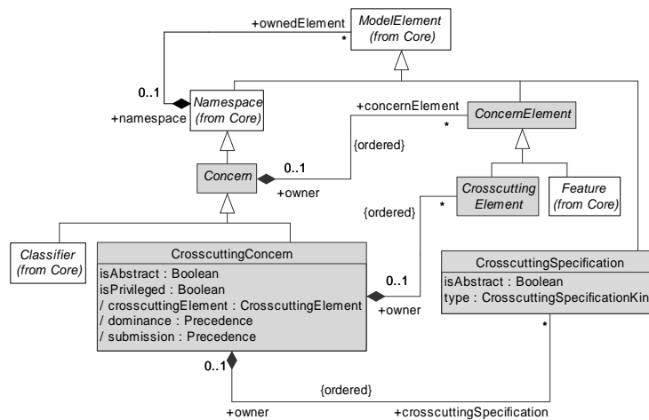
Figure 4.20. Aspect/UML — Syntaxe abstraite des préoccupations
