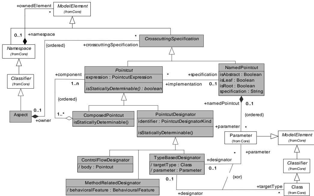
Figure 4.7. AspectJ/UML — Syntaxe abstraite des points de recouvrement
