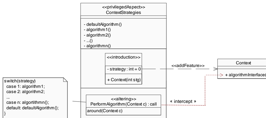
Figure 4.33. Modèle de Stratégie spécifique à AspectJ
