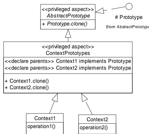
Figure 3.16. Solution en AspectJ du patron Prototype
