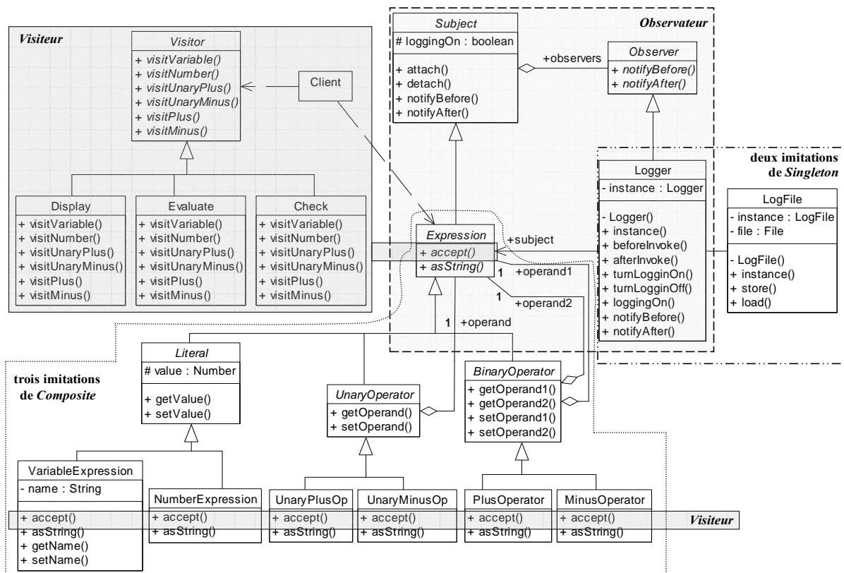
Figure 1.11. Résultat d'application des patrons Composite, Visiteur, Observateur et Singleton sur le système SEE
