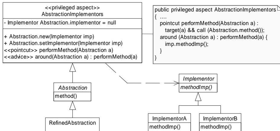
Figure 3.15. Solution en AspectJ du patron Pont
