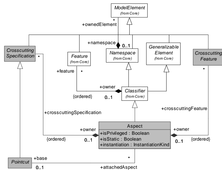
Figure 4.4. AspectJ/UML — Syntaxe abstraite d'un aspect
