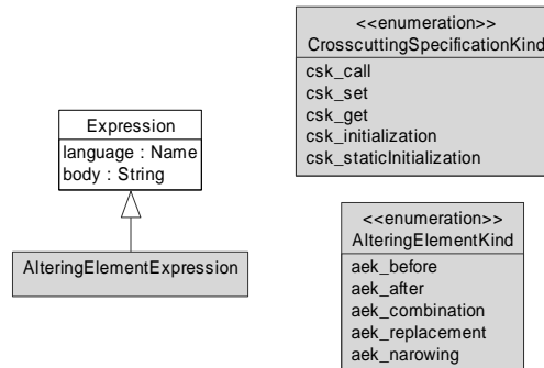
Figure 7.1. Aspect/UML — Types de données
