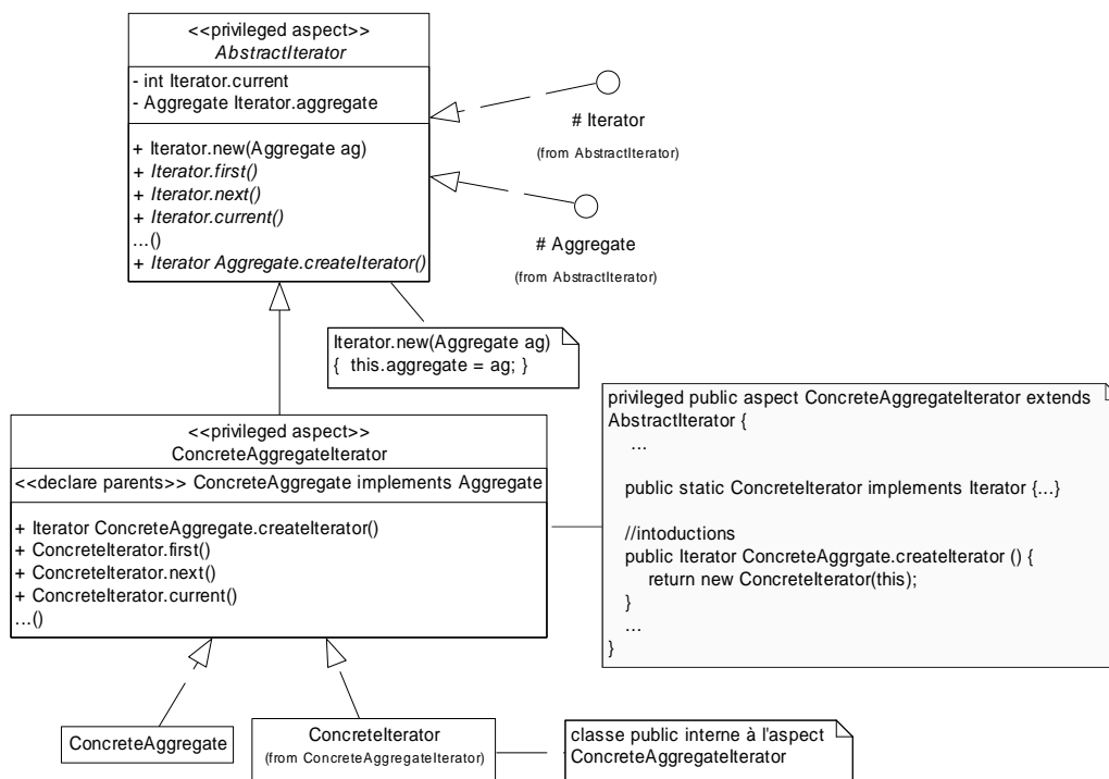
Figure 3.17. Solution en AspectJ du patron Itérateur
