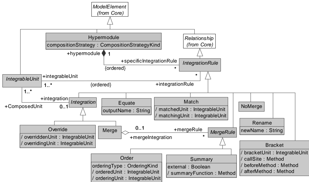
Figure 4.16. HyperJ/UML — Syntaxe abstraite des règles d'intégration spécifiques
