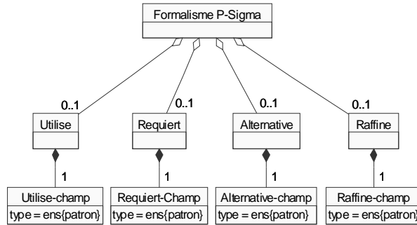
Figure 9.3. Modèle de la partie « Relations » de P-Sigma
