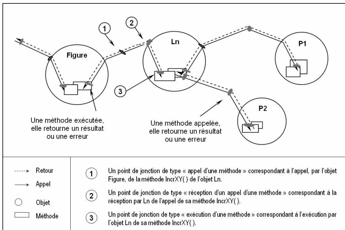
Figure 2.5. Exemples de points de jonction (issues de [Kiczales et al. , 01])
