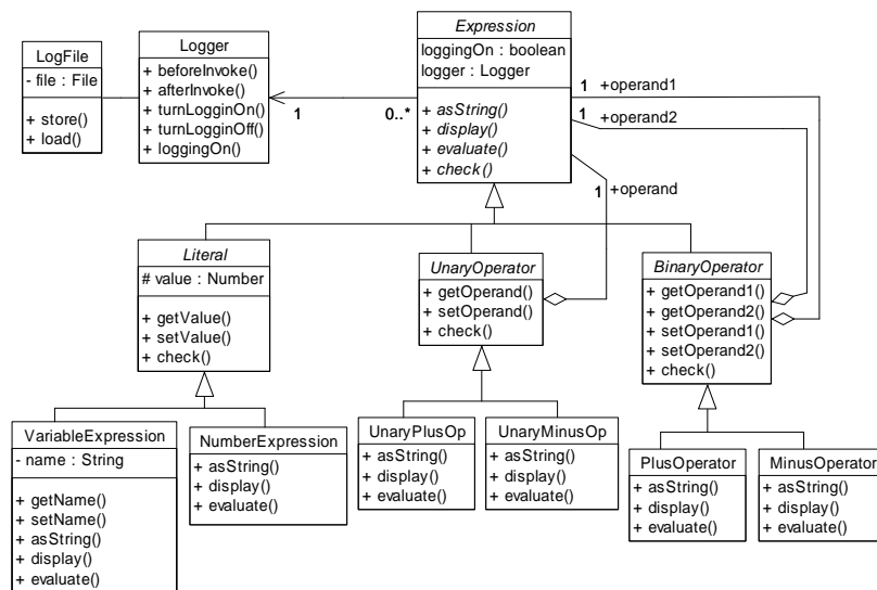
Figure 3.9. Diagramme de classes du système SEE
