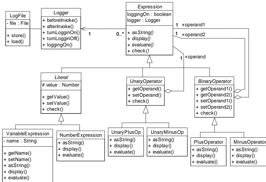
Figure 1.6. Diagramme de classes complété du système SEE
