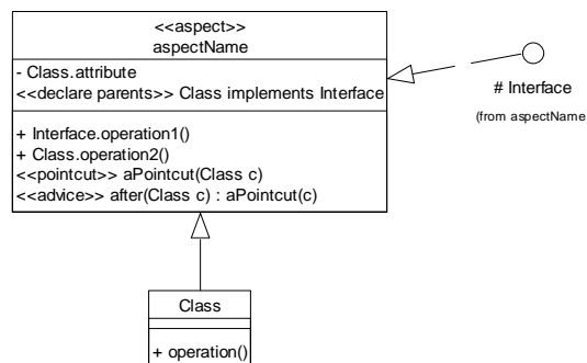
Figure 3.1. Notation pour AspectJ
