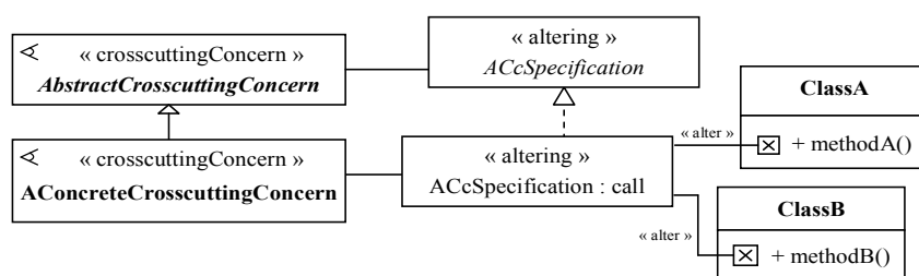
Figure 4.27. Aspect/UML — Représentation des spécifications d'entrecroisement
