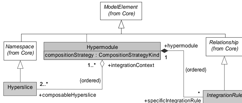
Figure 4.15. HyperJ/UML — Syntaxe abstraite des hypermodules
