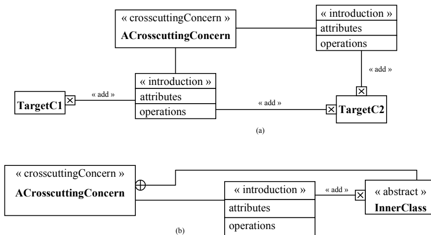
Figure 4.26. Aspect/UML — Représentation des introductions
