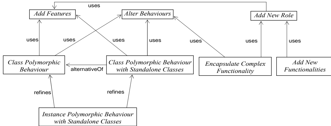
Figure 5.23. Système de patrons de conception par aspects
