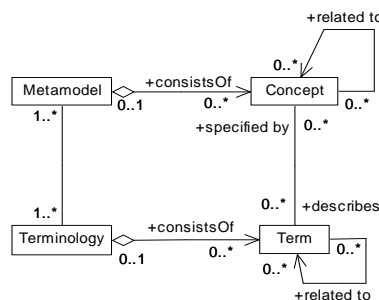
Figure 4.2. Identification et définition de la sémantique des concepts spécifiques
