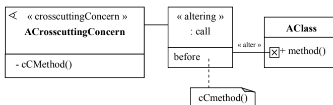
Figure 4.28. Aspect/UML — Représentation des éléments d'altération
