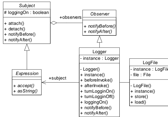
Figure 1.10. Application du patron Singleton sur le système SEE
