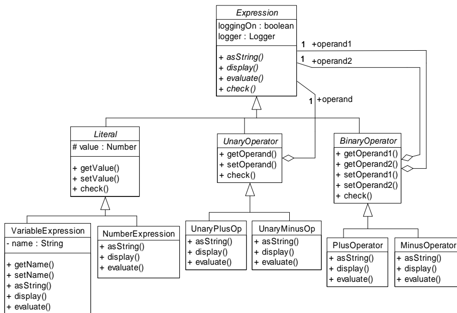
Figure 1.5. Diagramme de classes détaillé du système SEE
