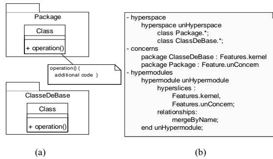
Figure 3.2. Notation pour Hyper/J
