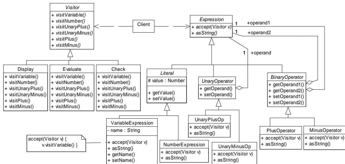
Figure 1.7. Application du patron Visiteur sur le système SEE
