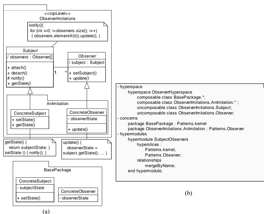
Figure 3.6. Solution en Hyper/J du patron Observateur
