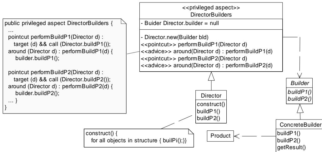
Figure 3.14. Solution en AspectJ du patron Monteur
