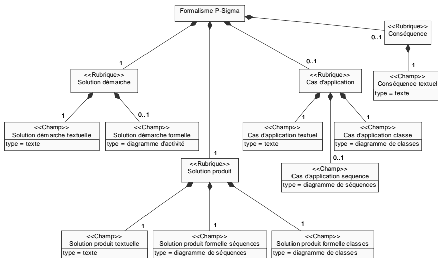
Figure 9.2. Modèle de la partie « Réalisation » du formalisme P-Sigma
