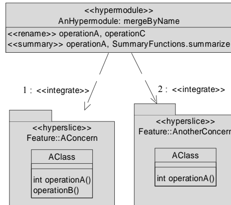
Figure 4.19. HyperJ/UML — Représentation des hypermodules et des règles d'intégration spécifiques
