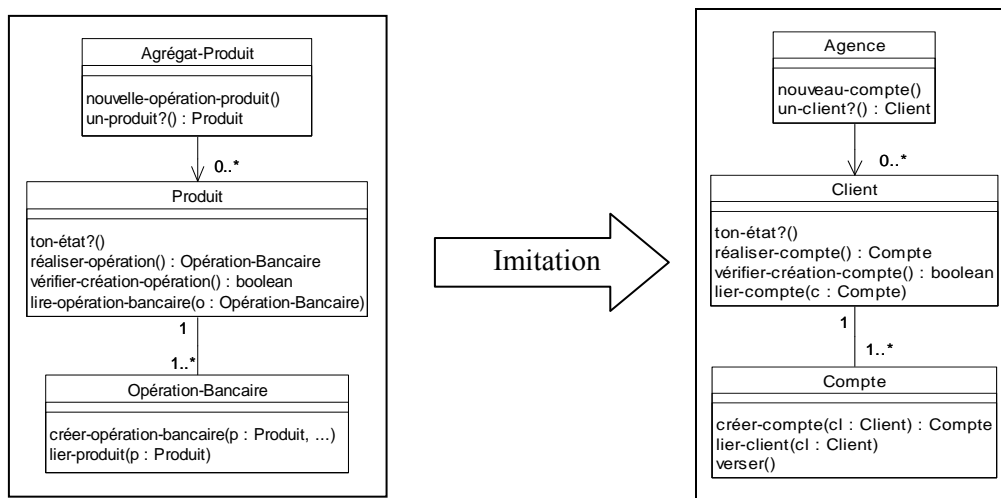
Figure 1.3. Exemple d'imitation d'un patron
