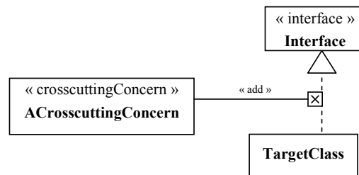
Figure 4.25. Aspect/UML — Représentation des déclarations d'héritage et de réalisation
