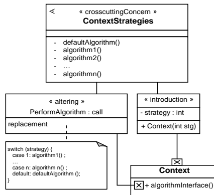
Figure 4.32. Modèle général par aspects du patron Stratégie
