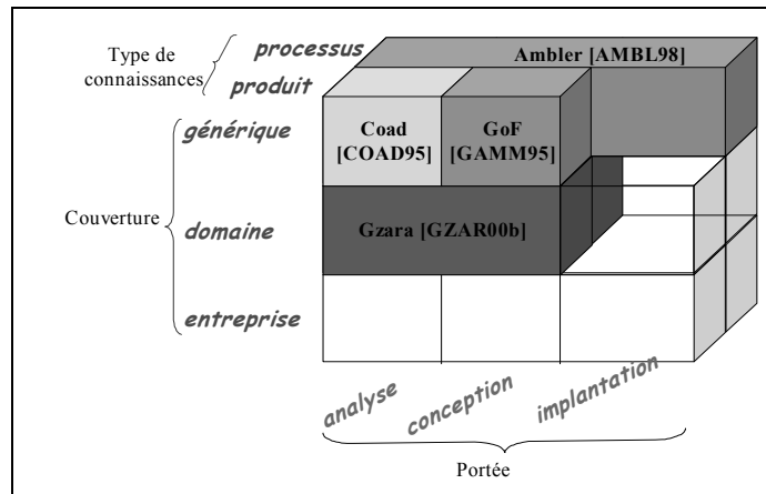
Figure 1.2. Système de patrons [Conte et al., 01c]
