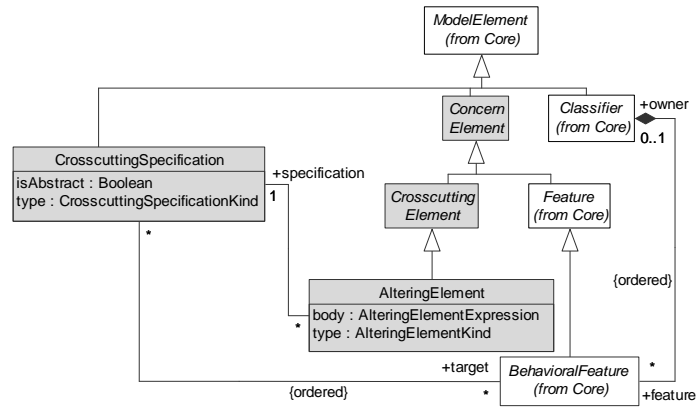
Figure 4.22. Aspect/UML — Syntaxe abstraite des spécifications d’entrecroisement
