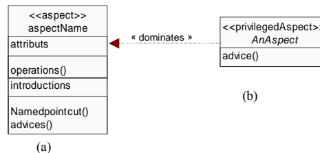
Figure 4.10. AspectJ/UML — Différentes représentations d'un aspect
