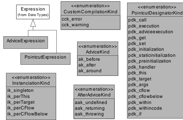
Figure 4.9. AspectJ/UML — Types de données
