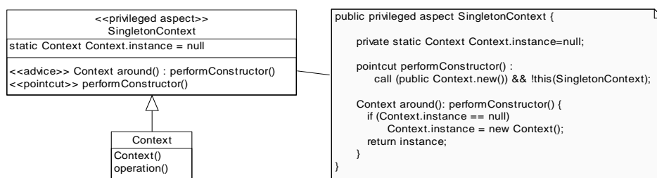
Figure 3.7. Solution en AspectJ du patron Singleton
