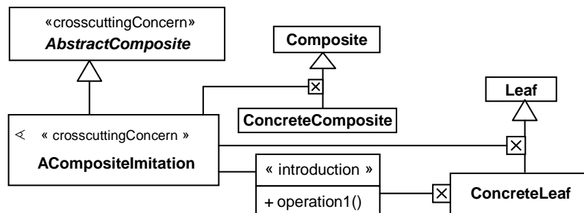
Figure 5.9. Structure par aspects de Composite
