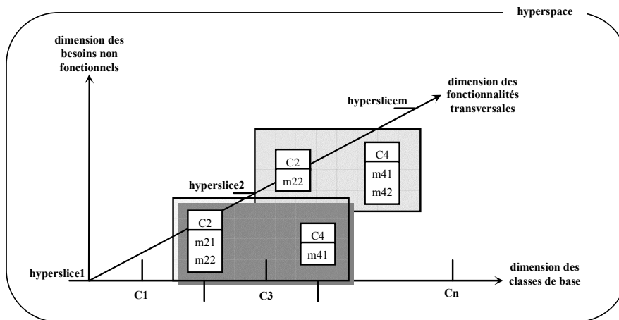
Figure 2.3. Principes de l'approche Hyperspace
