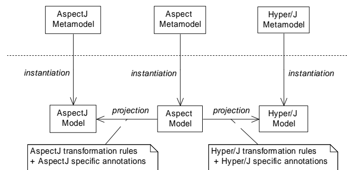
Figure 4.3. Métamodélisation des aspects et transformation de modèles
