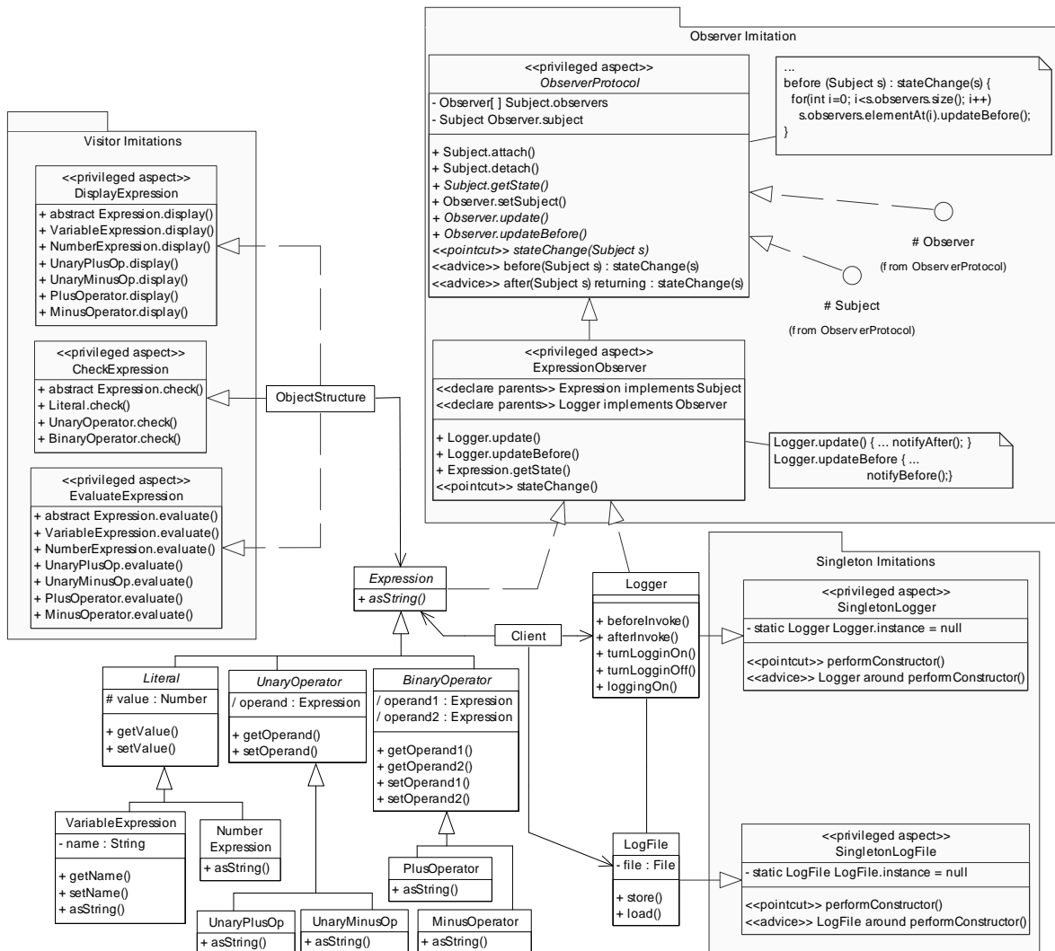
Figure 3.10. Application des solutions en AspectJ des patrons Visiteur, Observateur et Singleton sur le système SEE
