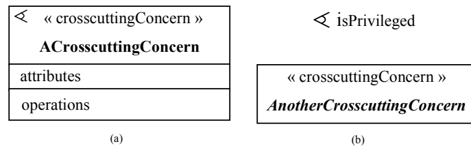
Figure 4.24. Aspect/UML — Représentation des préoccupations transversales
