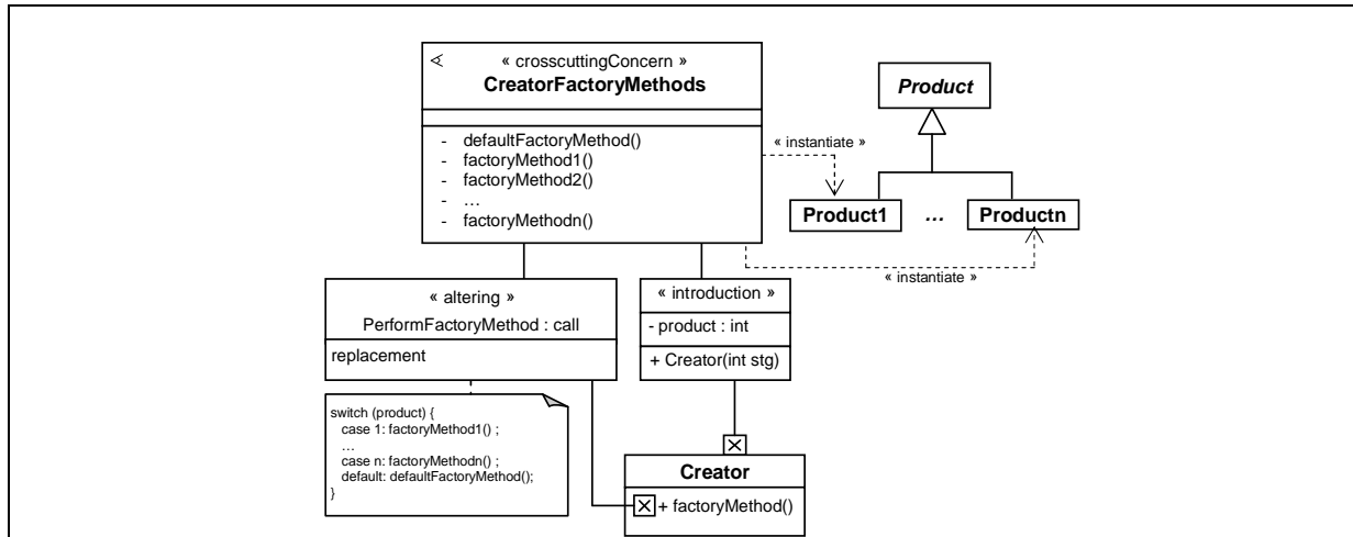
Figure 5.10. Structure par aspects de Fabrication
