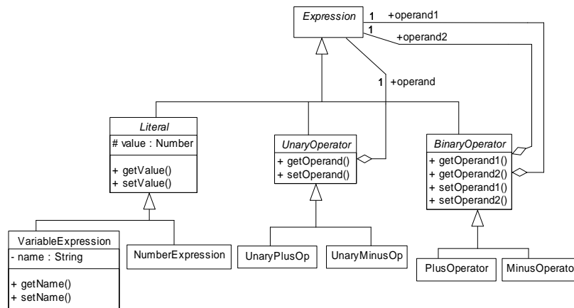
Figure 1.4. Application du patron Composite sur le système SEE
