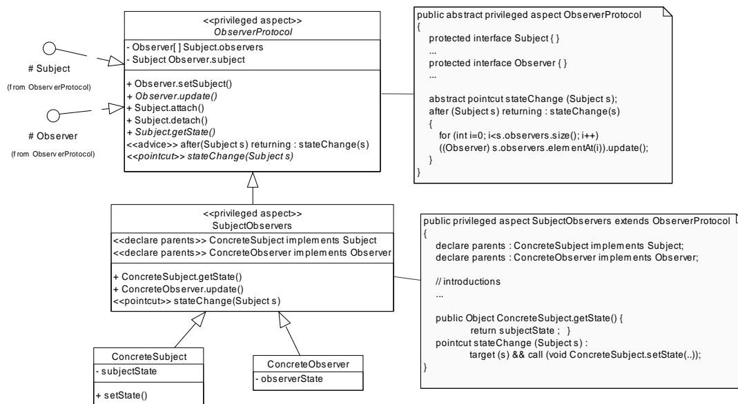
Figure 3.5. Solution en AspectJ du patron Observateur
