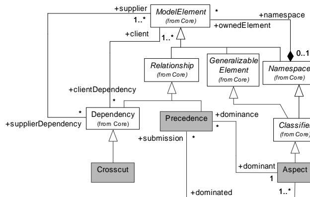
Figure 4.8. AspectJ/UML — Syntaxe abstraite des relations d'entrecroisement et de précedence
