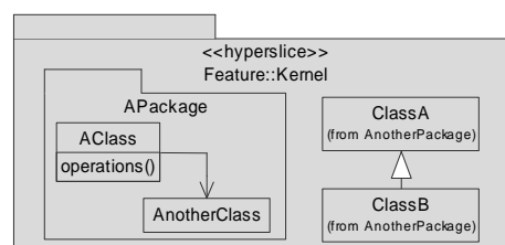
Figure 4.18. HyperJ/UML — Représentation des hyperslices
