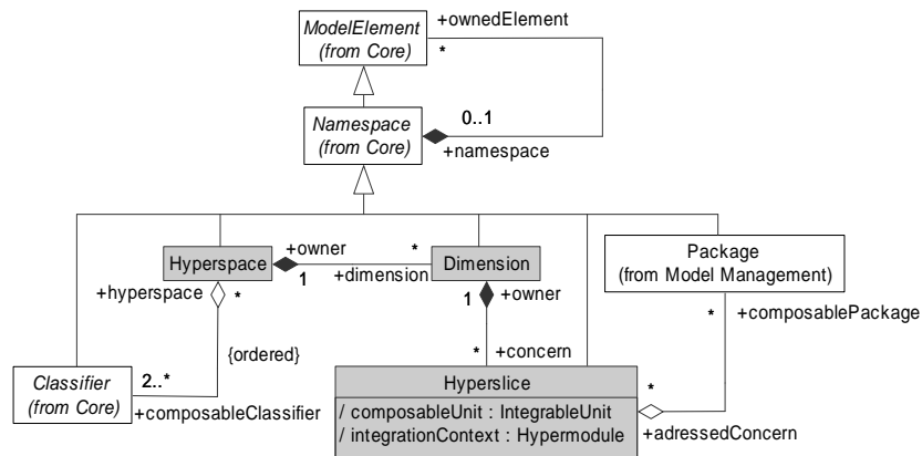
Figure 4.14. HyperJ/UML — Syntaxe abstraite d'une matrice de préoccupations
