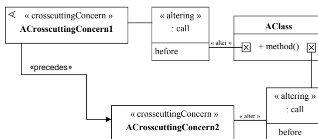
Figure 4.29. Aspect/UML — Représentation des relations de précedence
