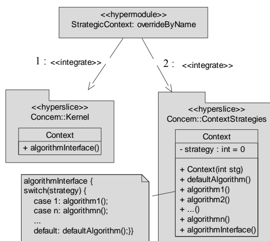
Figure 4.34. Modèle de Stratégie, spécifique à Hyper/J
