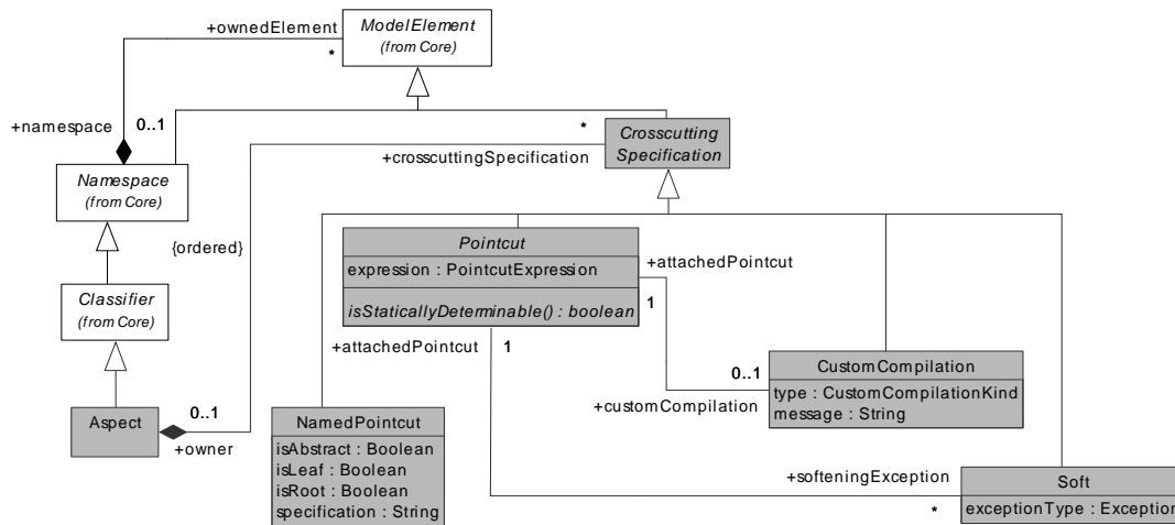
Figure 4.6. AspectJ/UML — Syntaxe abstraite des spécifications d'entrecroisement
