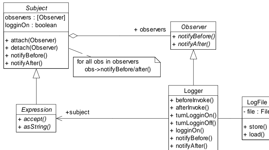
Figure 1.8. Application du patron Observateur sur le système SEE
