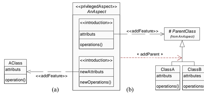
Figure 4.11. AspectJ/UML — Représentation des introductions et des déclarations d'héritage ou de réalisation
