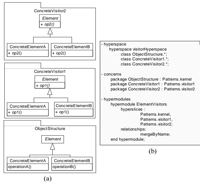
Figure 3.4. Solution en Hyper/J du patron Visiteur
