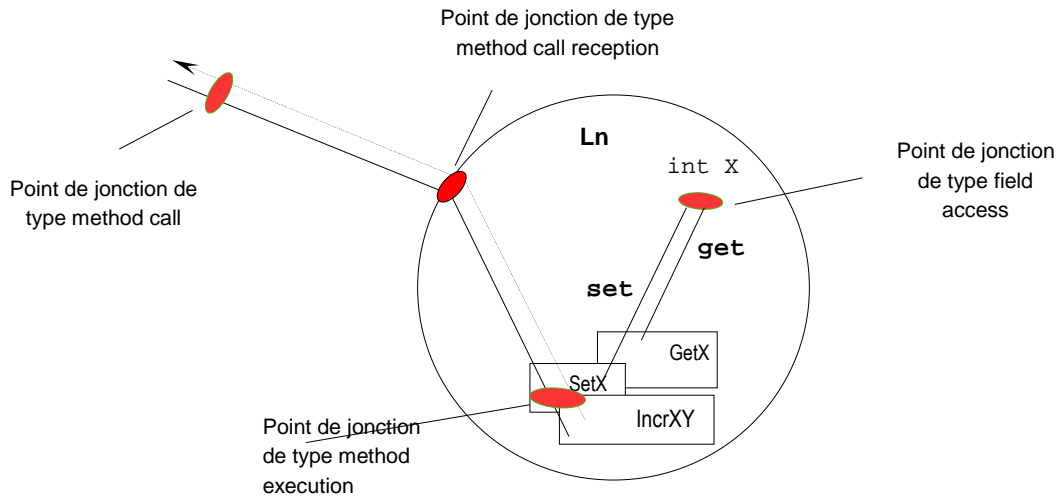
Figure 2.6. Types de points de jonction
