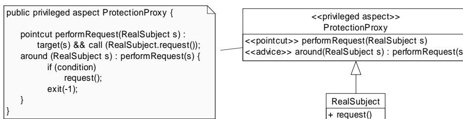
Figure 3.12. Solution en AspectJ du patron Procuration de protection
