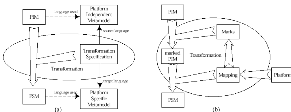
Figure 4.30. Approches MDA de transformation de modèles [OMG-MDA 03]
