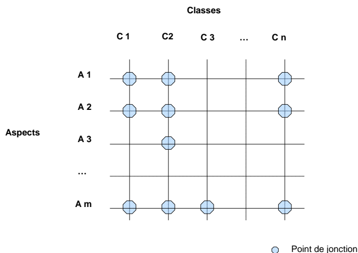
Figure 2.4. Entrecroisement entre aspects et classes en AOP [Bardou 98]
