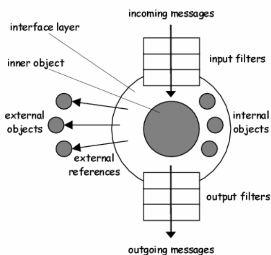
Figure 2.2. Éléments d'un objet dans le modèle Composition Filters [Aksit et al. , 96]
