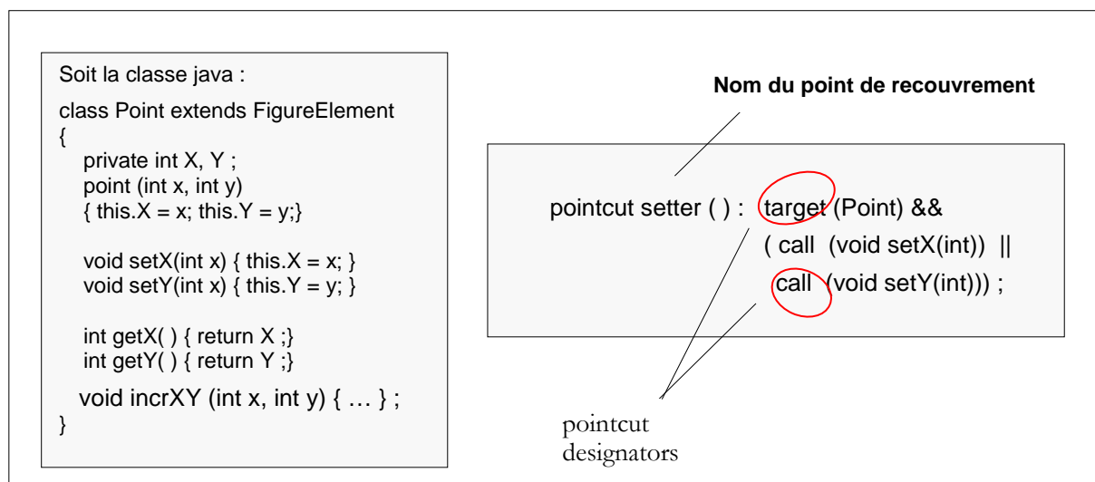
Figure 2.7. Exemple de point de recouvrement composé
