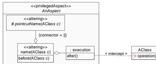
Figure 4.12. AspectJ/UML — Représentation des points de recouvrement et des perfectionnements
