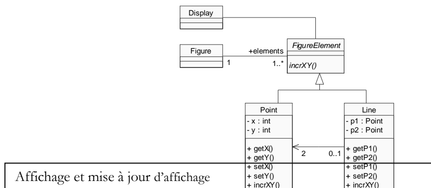
Figure 2.1. Diagramme de classes UML d'un éditeur de figures [Aspect] 02]
