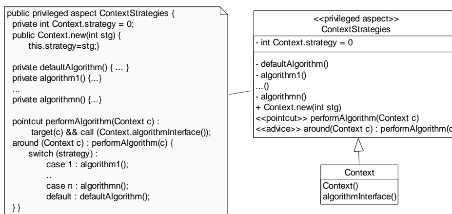
Figure 3.13. Solution en AspectJ du patron Stratégie
