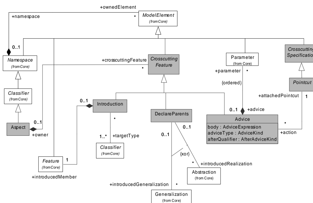
Figure 4.5. AspectJ/UML — Syntaxe abstraite des propriétés d'entrecroisement
