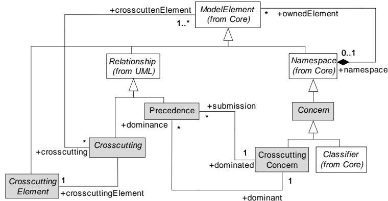
Figure 4.23. Aspect/UML — Syntaxe abstraite des relations d’entrecroisement et de précedence
