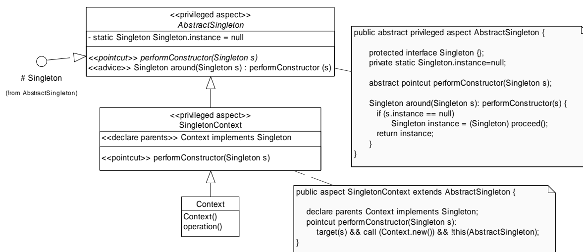
Figure 3.8. Une solution alternative à la solution en AspectJ du patron Singleton
