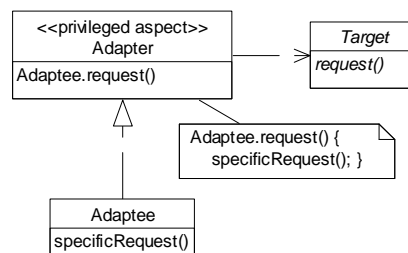
Figure 3.11. Solution en AspectJ du patron Adaptateur
