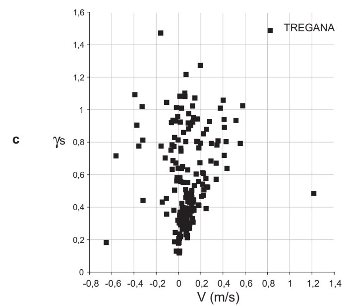
Illustration 115. Courant transversal et longitudinal, U et V , fonction de la hauteur relative des vagues \gamma_s à Porsmilin, Corssen et Tregana
