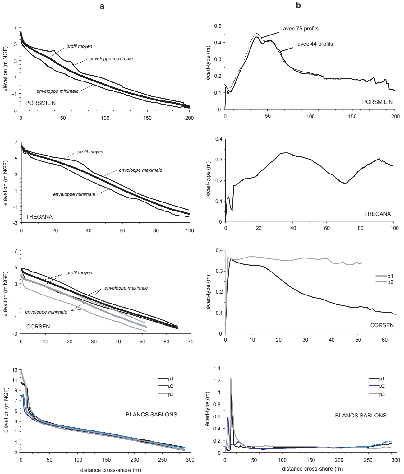
Illustration 36. (a) Profil moyen, enveloppes minimale et maximale des profils, (b) écart-type des élévations des profils des plages de Porsmilin, Corssen, Tregana et des Blancs Sablons
