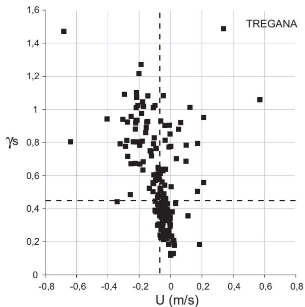
Illustration 115. Courant transversal et longitudinal, U et V , fonction de la hauteur relative des vagues \gamma_s à Porsmilin, Corssen et Tregana
