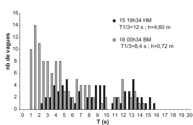
Illustration 122. Spectres d'énergie des vagues et histogrammes des périodes des vagues individuelles lors de deux situations de marées hautes (HM) et basses (BM) sur la plage de Corsen, (a) lors d'une houle bien établie, (b) lors de conditions mixtes de houle et mer du vent.
