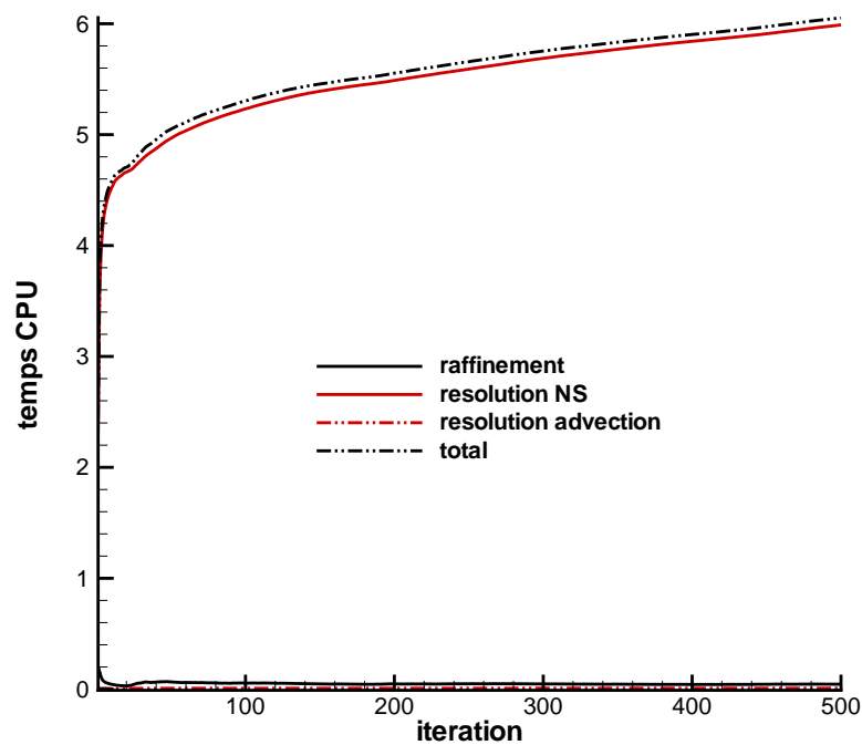
Figure 4.12 : Comparaison des temps CPU moyens avec trois niveaux fins et sans AMR.
