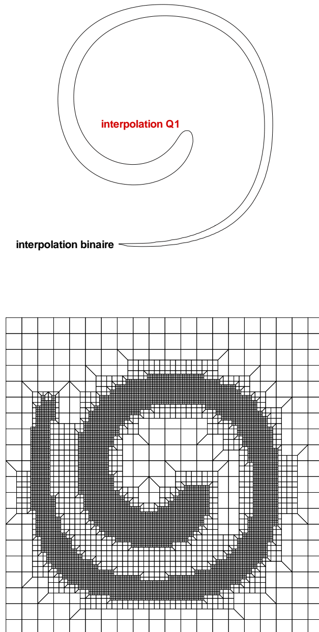
Figure 3.4 : Isovaleur S_p = 0.5g.m^{-3} obtenue par interpolation Q_1 (en rouge sur la figure du haut) et binaire (en noir sur la figure du haut) de S_p , sur G_2 . t = 8s , G_0 = 20 * 20 , vitesse analytique imposée sur tous les nœuds vitesses. Maillage AMR utilisé (bas).
