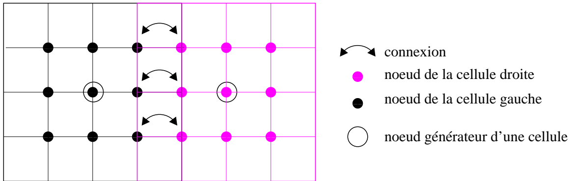
Figure 2.1 : Connexion des nœuds scalaires de deux cellules AMR .
