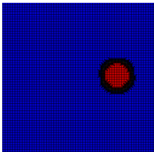
Figure 4.9 : Fluide coloré à t = 0.001s , maillage G_0 = 90 * 90 avec un niveau AMR .
