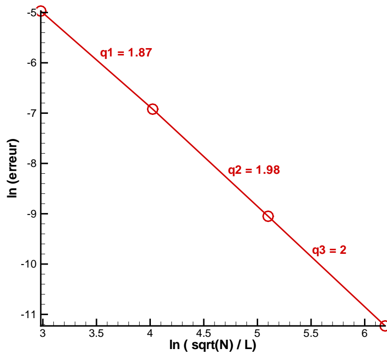
Figure 3.41 : Convergence de l'AMR en augmentant le nombre de niveaux. Les données proviennent du tableau 3.15.
