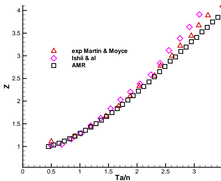
Figure 4.16 : Position adimensionnée de l'interface Z pour la rupture de barrage sur fond sec avec n^2 = 2 . G_0 = 100 * 30 avec un niveau de raffinement, \Delta t = 10^{-4}s .
