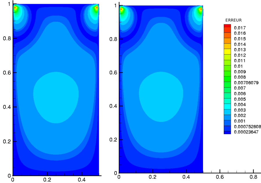
Figure 3.37 : Répartition de l'erreur e_r lorsque la température est imposée sur les bords du domaine avec 1 niveau d'AMR ( G_0 = 16 * 16 ) à droite et sans AMR ( G = 48 * 48 ) à gauche.
