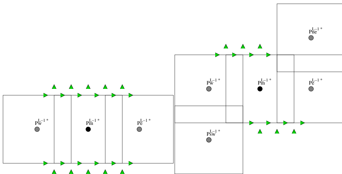
Figure 2.14 : Deux voisins ont généré une cellule AMR. Aucun voisin oblique (gauche), deux voisins obliques (droite). Nœuds interpolés représentés en vert.
