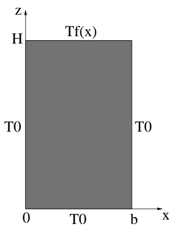
Figure 3.34 : Conduction 2D dans un rectangle dont les bords sont chauffés à des températures différentes.
