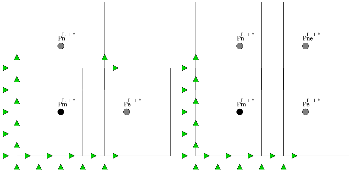
Figure 2.12 : Deux voisins ont g n r  une cellule AMR. Aucun voisin oblique (gauche), un voisin oblique (droite). N uds interpol s repr sent s en vert.
