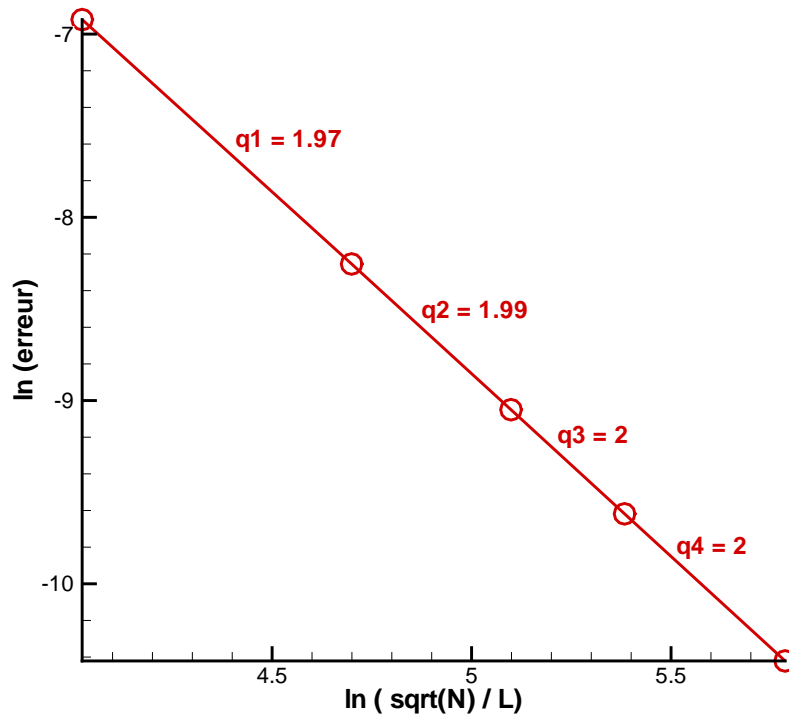
Figure 3.40 : Convergence en maillage avec deux niveaux fins. Les données proviennent du tableau 3.14.
