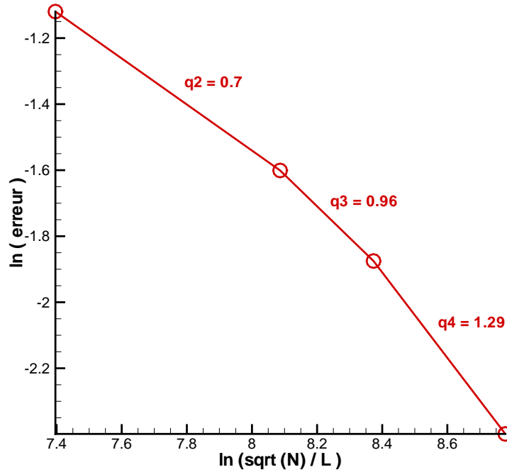
Figure 3.12 : Courbe de convergence pour un coefficient D = 10^{-9}m^2.s^{-1} sans AMR .
