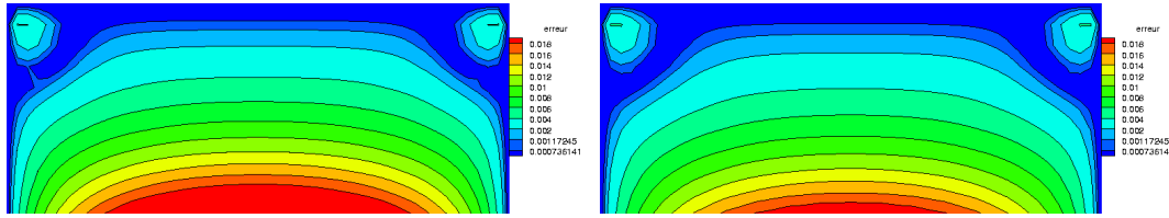
Figure 3.46 : Répartition de l'erreur sur le niveau fin avec interpolation Q_1 et injection conservative sur la gauche puis injection directe sur la droite.
