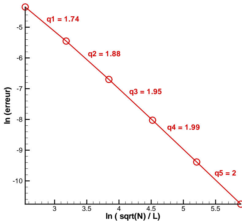
Figure 3.38 : Ordres de convergence successifs sans AMR. Les données proviennent du tableau 3.12.
