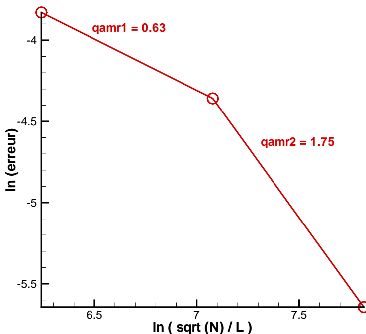
Figure 3.13 : Courbe de convergence pour un coefficient D = 10^{-8}m^2.s^{-1} avec AMR .
