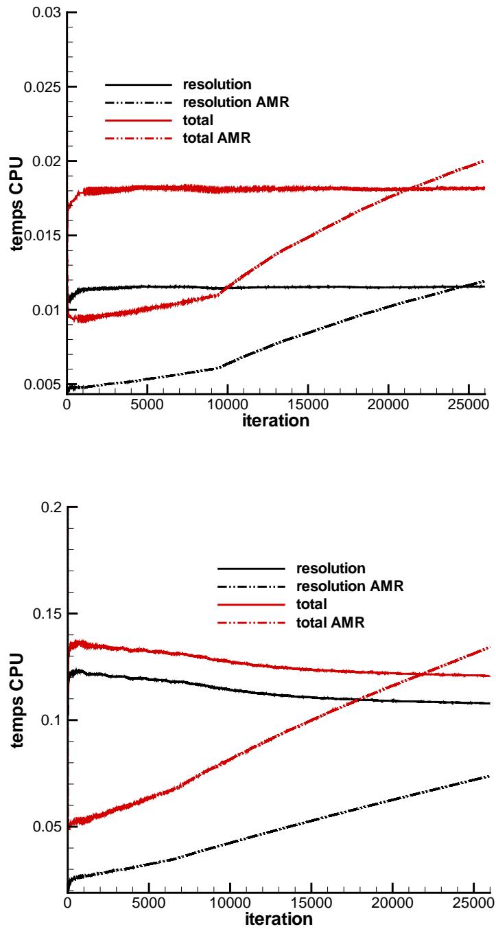
Figure 3.21 : Comparaison des temps CPU moyens avec un niveau de raffinement et sans AMR en haut. Comparaison des temps CPU moyens avec deux niveaux fins et sans AMR en bas.
