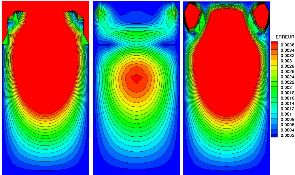
Figure 3.42 : Erreurs entre la solution analytique et numérique sur le niveau grossier G_0 = 16 * 16 avec une injection FWCV (gauche), directe (centre) sans injection (droite) lorsque l'ensemble du domaine est raffiné.
