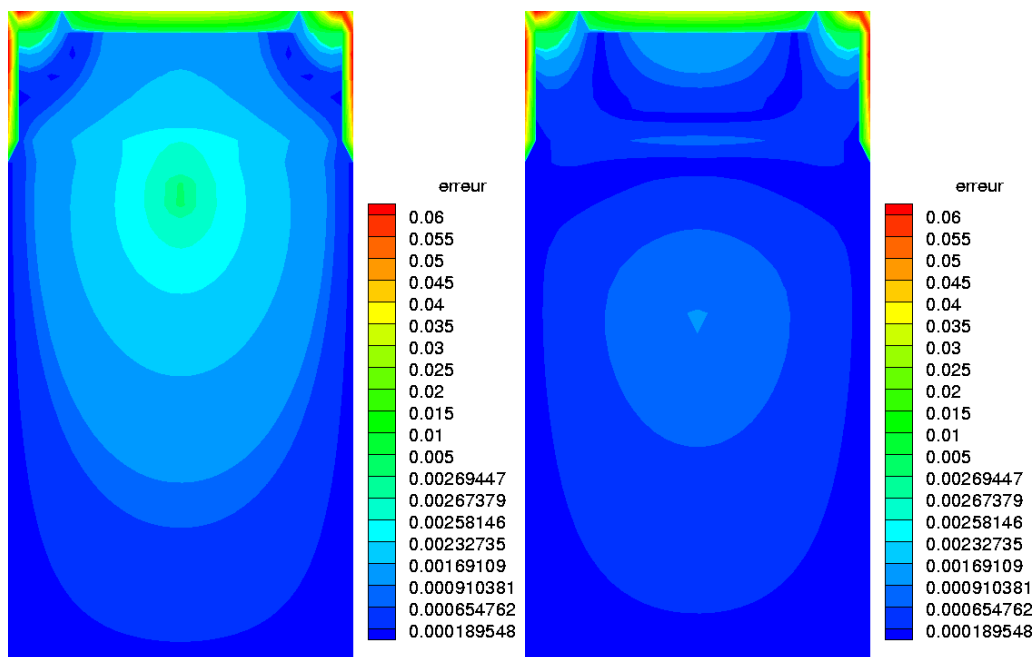
Figure 3.47 : Répartition de l'erreur sur le niveau G_0 = 32 * 32 avec interpolation Q_2 sur la gauche puis une interpolation conservatrice ( FIC ) sur la droite. Injection FWCV .
