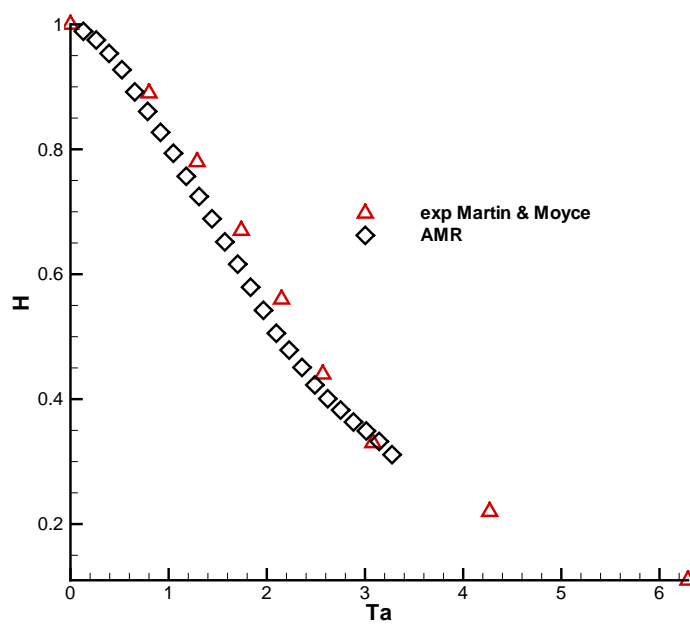
Figure 4.15 : Hauteur d'eau adimensionnée de l'interface H pour la rupture de barrage sur fond sec avec n^2 = 1 . G_0 = 100 * 30 avec un niveau de raffinement, \Delta t = 2.10^{-4}s .
