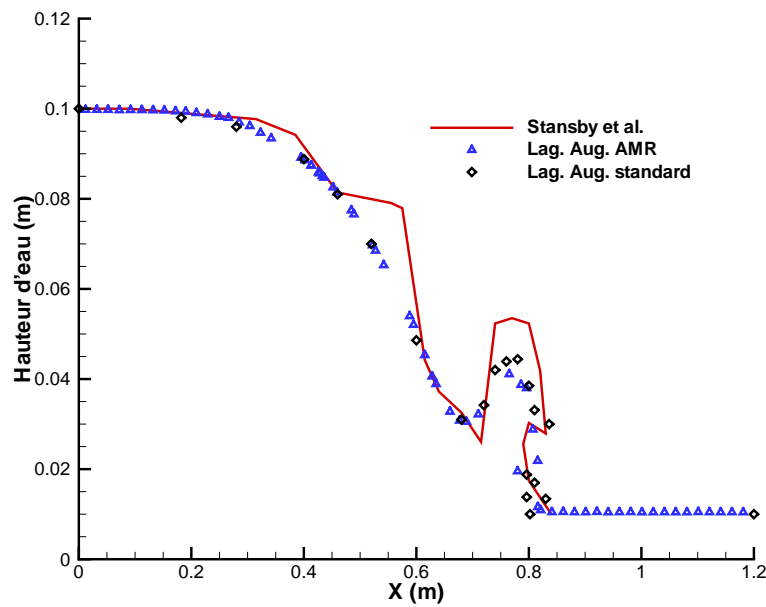
Figure 4.21 : Hauteur d'eau dans le domaine à l'instant t = 0.24s . G_0 = 400 * 47 avec un niveau de raffinement, \Delta t = 2 \cdot 10^{-4}s . Rupture sur fond mouillé, h_f = 0.01m . Rupture sur fond mouillé, h_f = 0.01m .
