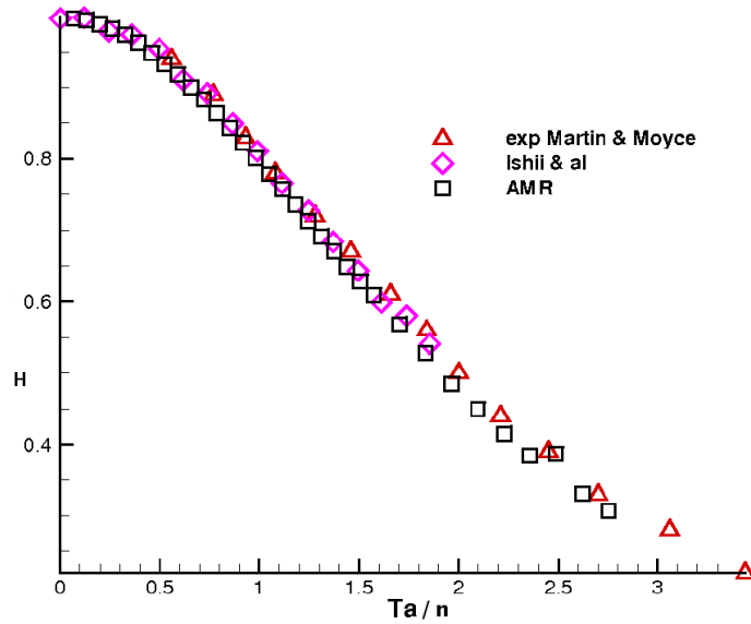
Figure 4.18 : Hauteur d'eau adimensionnée de l'interface H pour la rupture de barrage sur fond sec avec n^2 = 2 . G_0 = 100 * 30 avec un niveau de raffinement, \Delta t = 10^{-4} s .
