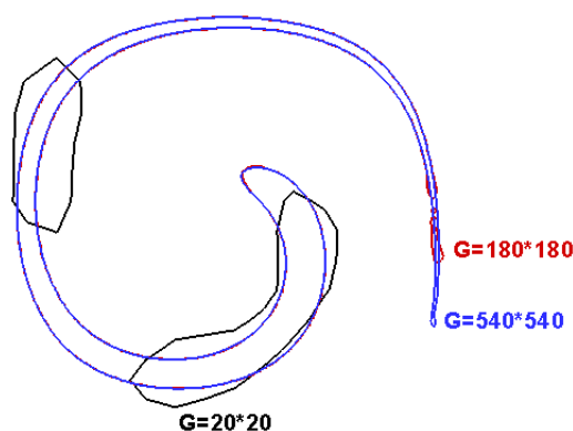
Figure 3.23 : Position de l'interface à t = 6.3s pour des maillages de pas d'espace différents. \Delta t = 0.0009s .
