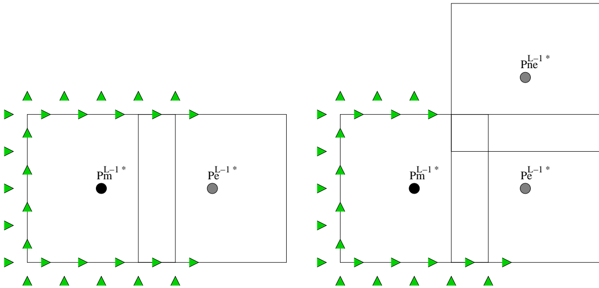
Figure 2.11 : Un seul voisin Est a g n r  une cellule AMR. Aucun voisin oblique (gauche), un voisin oblique (droite). N uds interpol s repr sent s en vert.
