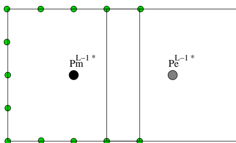
Figure 2.4 : Une seule voisine a généré une cellule AMR (Nœuds interpolés en vert).
