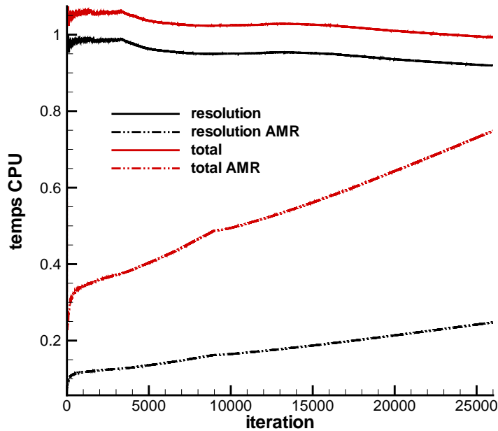
Figure 3.22 : Comparaison des temps CPU moyens avec trois niveaux fins et sans AMR.
