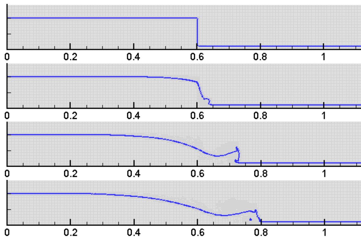
Figure 4.19 : Avancée de l'interface à t = 0.01s , t = 0.06s , t = 0.16s puis t = 0.22s (de haut en bas). G_0 = 400 * 47 avec un niveau de raffinement, \Delta t = 2 \cdot 10^{-4}s . Rupture sur fond mouillé, h_f = 0.01m .
