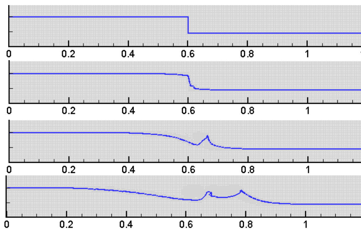
Figure 4.22 : Avancée de l'interface à t = 0.005s , t = 0.04s , t = 0.12s puis t = 0.3s (de haut en bas). G_0 = 400 * 47 avec un niveau de raffinement, \Delta t = 10^{-4}s . Rupture sur fond mouillé, h_f = 0.045m .
