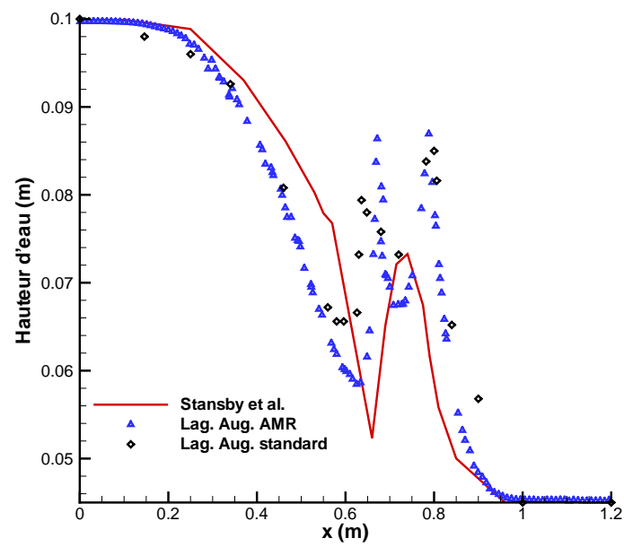
Figure 4.25 : Hauteur d'eau dans le domaine à l'instant t = 0.3s . G_0 = 400 * 47 avec un niveau de raffinement, \Delta t = 10^{-4}s . Rupture sur fond mouillé, h_f = 0.045m .
