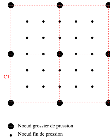
Figure 2.29 : Interpolation Q_2 sur les nœuds de pression
