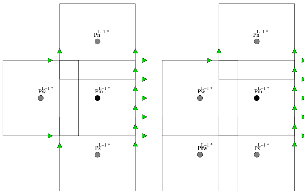
Figure 2.13 : Trois voisins ont généré une cellule AMR. Aucun voisin oblique (gauche), un voisin oblique (droite). Nœuds interpolés représentés en vert.
