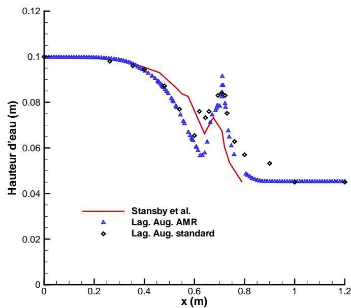
Figure 4.24 : Hauteur d'eau dans le domaine à l'instant t = 0.2s . G_0 = 400 * 47 avec un niveau de raffinement, \Delta t = 10^{-4}s . Rupture sur fond mouillé, h_f = 0.045m .
