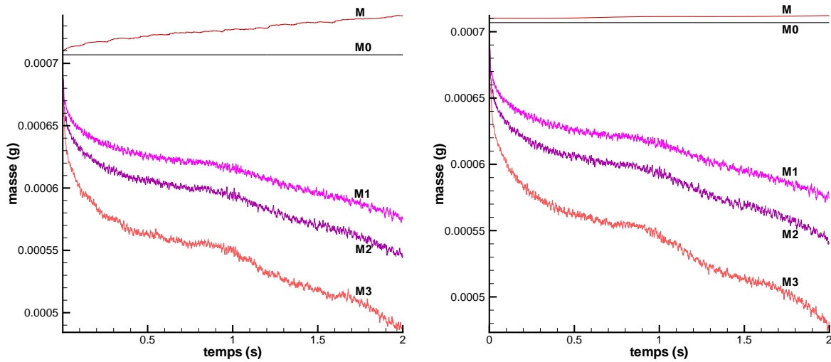
Figure 3.7 : Evolution de la masse, avec G_0 = 16 * 16 et deux niveaux de raffinement pour la figure de gauche et avec G = 144 * 144 sans AMR pour la figure de droite. Vitesse interpolée sur les niveaux fins avec du Q_1 et analytique ailleurs. Interpolation binaire de S_p pour les nœuds de limites des niveaux de raffinement.
