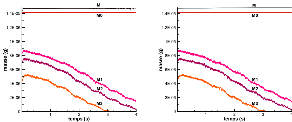
Figure 3.56 : Evolution des masses pour la tache cisillée autour de l'axe x avec un niveau de raffinement (gauche) et sans AMR (droite) pendant 4s. D = 10^{-8}m^2.s^{-1} .
