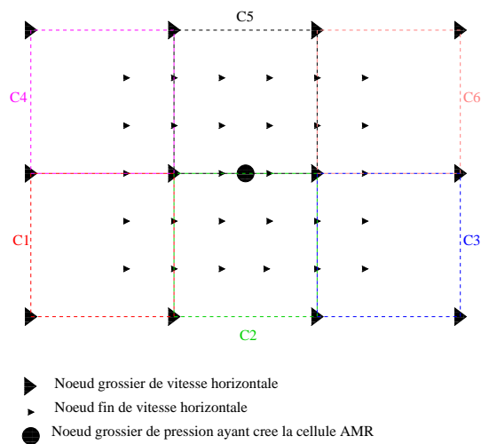
Figure 2.28 : Interpolation Q_1 sur les nœuds de vitesse horizontale
