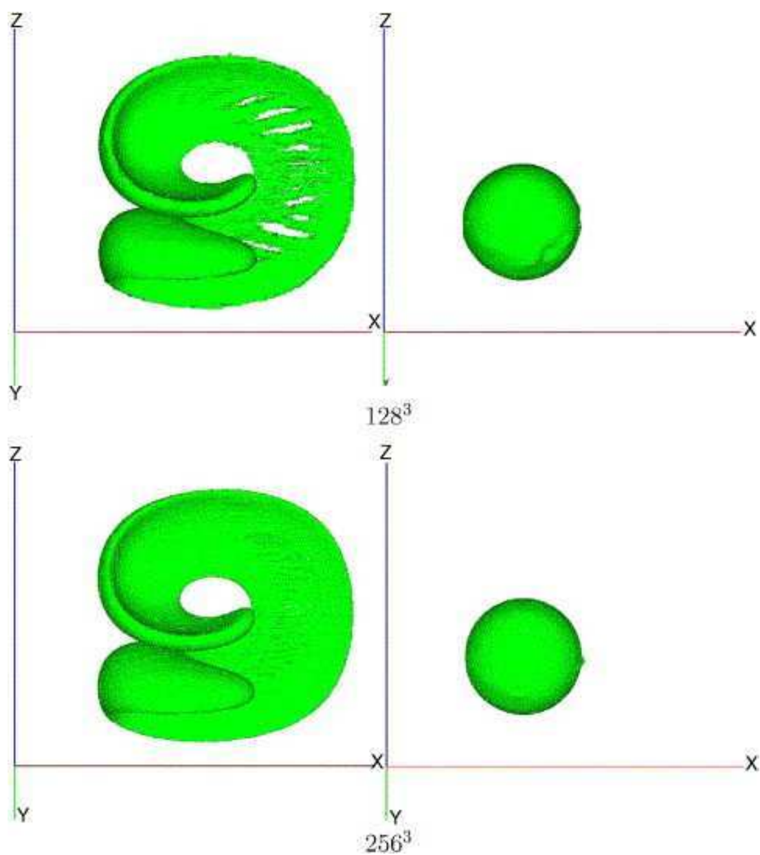
Figure 3.57 : Représentation de l'interface à son maximum de déformation ( t = 1.5s ) et à son minimum ( t = 3s ) pour un maillage G = 128 * 128 * 128 (haut) et G = 256 * 256 * 256 (bas) ([LIOVIC 06]).
