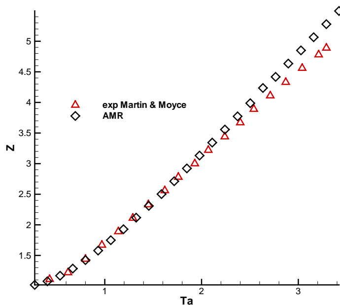
Figure 4.14 : Position adimensionnée de l'interface Z pour la rupture de barrage sur fond sec avec n^2 = 1 . G_0 = 100 * 30 avec un niveau de raffinement, \Delta t = 2.10^{-4}s .
