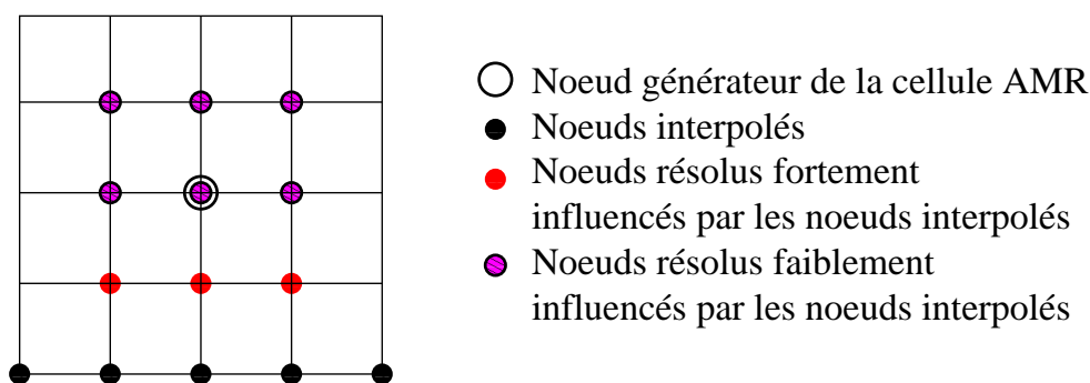
Figure 3.44 : Influence de l'interpolation Q_2 sur les nœuds résolus par discrétisation.
