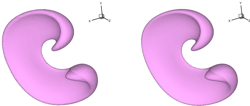
Figure 3.58 : Représentation de l'interface à t = 0.75s , pour un maillage G_0 = 12 * 12 * 12 (gauche) et G = 22 * 22 * 22 (droite), avec deux niveaux fins et un schéma TVD.
