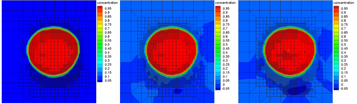
Figure 3.3 : Concentration massique interpolée sur les limites des niveaux de raffinement par une interpolation Q_1 (gauche), Q_2 (centre) et Q_3 (droite) à t = 0.1s . Vitesse analytique imposée sur tous les nœuds vitesses.
