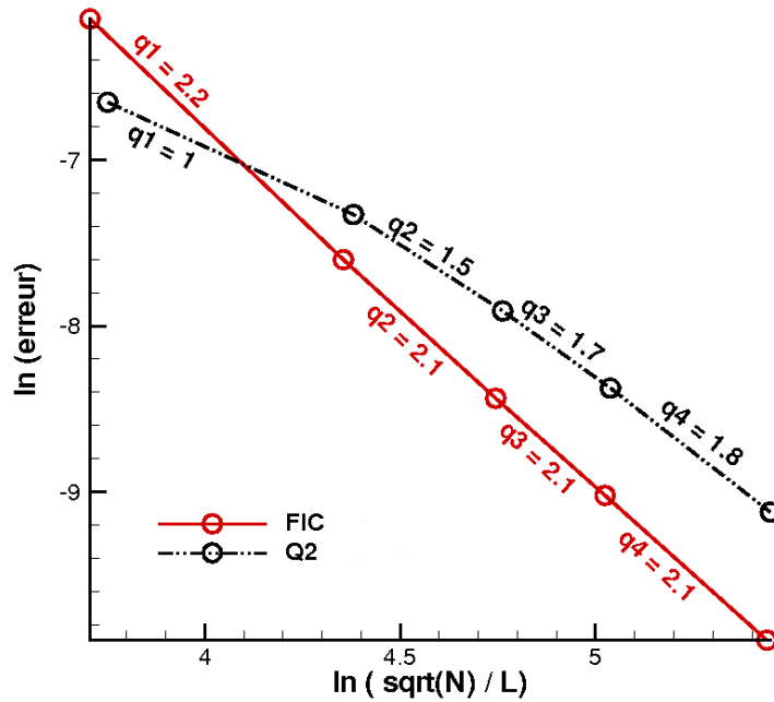
Figure 3.48 : Comparaison des ordres de convergence obtenus avec une interpolation Q_2 à ceux obtenus avec une interpolation conservative (FIC). Injection FWCV.
