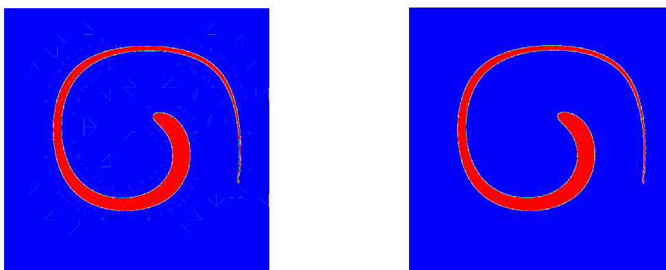
Figure 3.24 : Comparaison de la position de l'interface avec trois niveaux de raffinement (gauche) et sans AMR sur un maillage fin équivalent (droite) à t = 6.3s .
