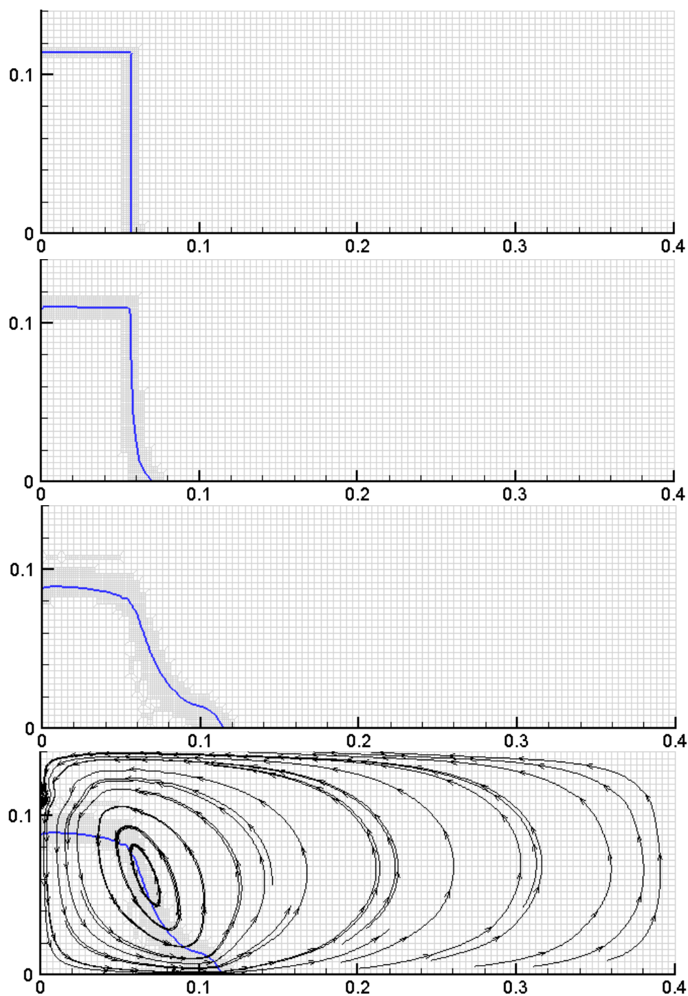
Figure 4.17 : Avancée de l'interface à t = 0.005s , t = 0.03s puis t = 0.08s (de haut en bas) pour la rupture de barrage sur fond sec avec n^2 = 2 . Lignes de courant pour t = 0.08s . G_0 = 100 * 30 avec un niveau de raffinement, \Delta t = 10^{-4}s .
