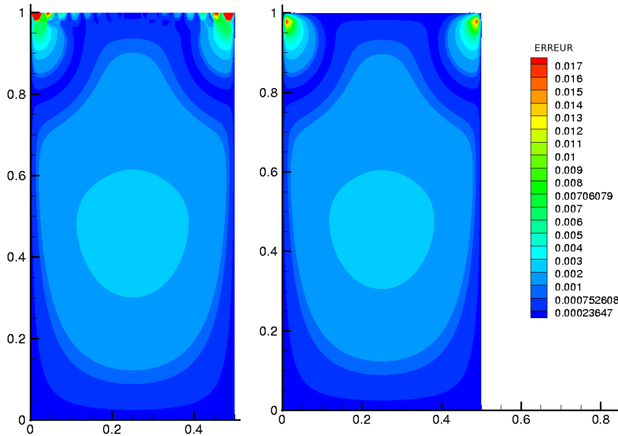
Figure 3.36 : Répartition de l'erreur e_r lorsque la température est imposée sur les bords du domaine à droite et interpolée à gauche. Maillage G_0 = 16 * 16 avec un niveau fin.
