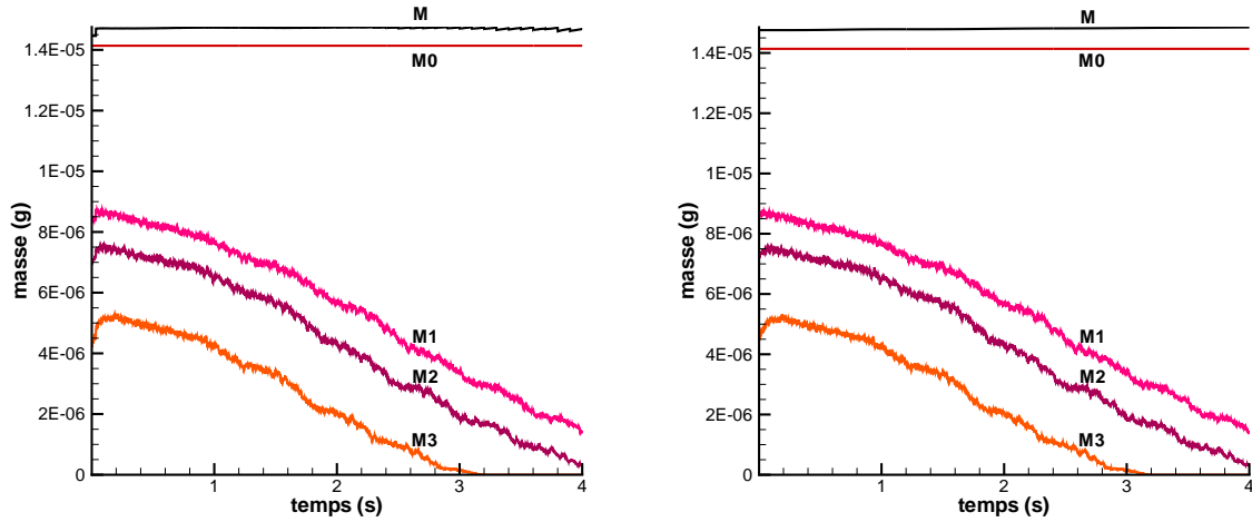
Figure 3.54 : Evolution des masses pour la tache cisailée autour de l'axe z avec un niveau de raffinement (gauche) et sans AMR (droite) pendant 4s. D = 10^{-8}m^2.s^{-1} .
