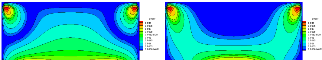
Figure 3.45 : Répartition de l'erreur sur le niveau fin avec interpolation Q_2 et injection conservative sur la gauche puis injection directe sur la droite.
