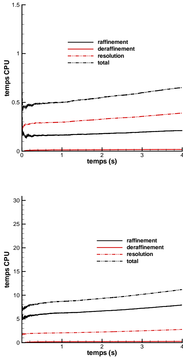
Figure 3.52 : Comparaison des différents temps moyens avec AMR pendant t = 4s . G_0 = 16 * 16 * 16 avec un niveau à gauche. G_0 = 12 * 12 * 12 avec deux niveaux à droite.
