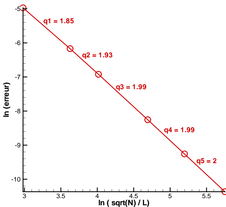
Figure 3.39 : Convergence en maillage avec un niveau d'AMR. Les données proviennent du tableau 3.13.
