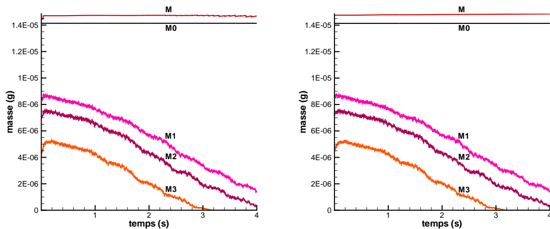
Figure 3.49 : Evolution des masses pour la tache cisailée autour de l'axe y avec un niveau de raffinement (gauche) et sans AMR (droite) pendant 4s. D = 10^{-8}m^2.s^{-1} .
