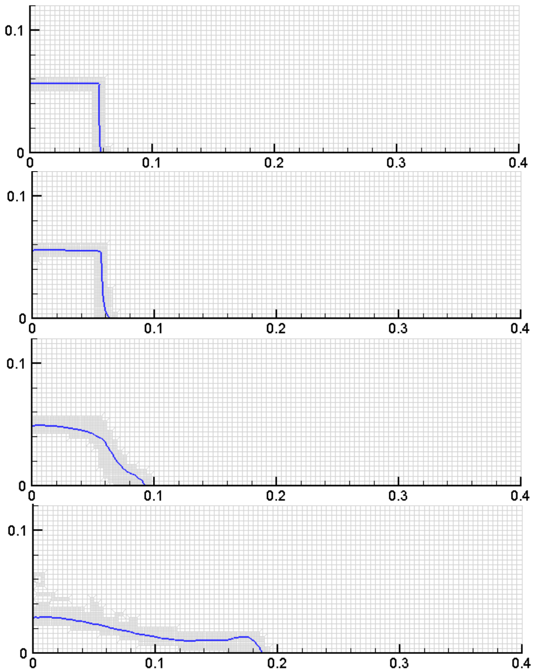
Figure 4.13 : Avancée de l'interface à t = 0.01s , t = 0.02s , t = 0.06s puis t = 0.16s (de haut en bas) pour la rupture de barrage sur fond sec avec n^2 = 1 . G_0 = 100 * 30 avec un niveau de raffinement, \Delta t = 2.10^{-4}s .
