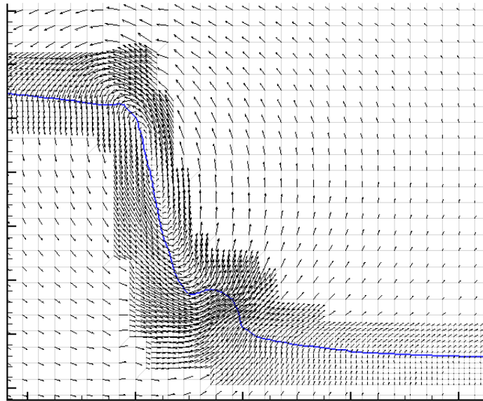
Figure 4.23 : Champ de vitesses à t = 0.04s . G_0 = 400 * 47 avec un niveau de raffinement, \Delta t = 10^{-4}s . Rupture sur fond mouillé, h_f = 0.045m .
