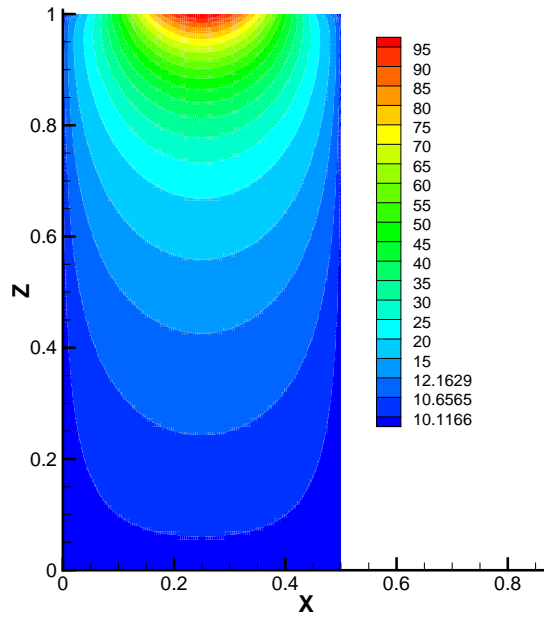
Figure 3.35 : Répartition analytique de la température sur un maillage G = 48 * 48 .
