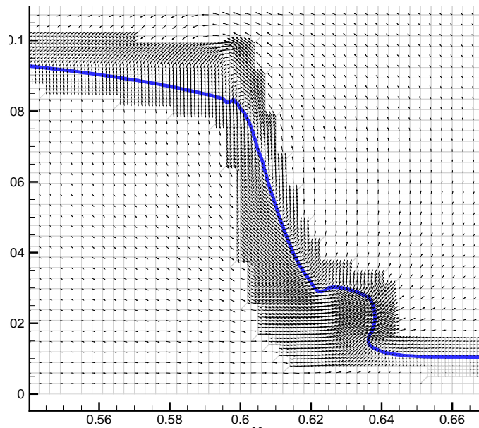
Figure 4.20 : Champ de vitesses à t = 0.06s . G_0 = 400 * 47 avec un niveau de raffinement, \Delta t = 2 \cdot 10^{-4}s . Rupture sur fond mouillé, h_f = 0.01m .
