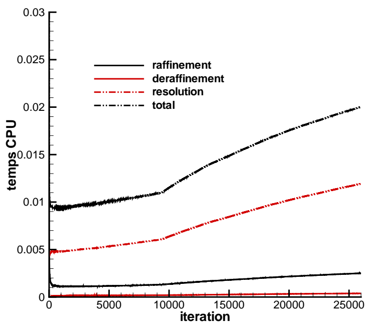
Figure 3.18 : Temps CPU moyens avec un niveau de raffinement.
