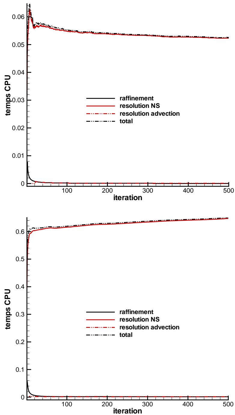
Figure 4.11 : Comparaison des temps CPU moyens avec un niveau d'AMR (resp deux niveaux) et sans AMR en haut (resp en bas).
