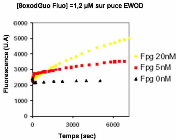
Figure 112: Détection minimale de Fluorescence sur EWOD
