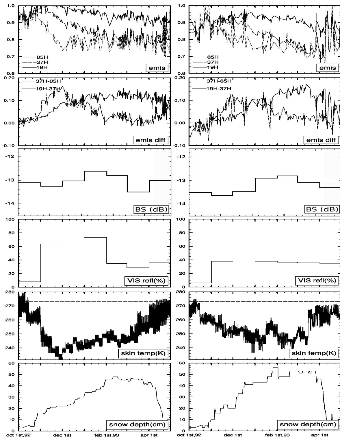
FIG. 4.11: Les séries temporelles entre octobre 1992 et avril 1993 en deux points du globe. À gauche en Russie ( 134,7^{\circ}\text{E};60,4^{\circ}\text{N} ) (a) et à droite au Canada ( 293,3^{\circ}\text{E};54,9^{\circ}\text{N} ) (b). De haut en bas : les émissivités à 19 GHz, 37 GHz et 85 GHz en polarisation horizontale (SSM/I F-10 et F-11), les différences d'émissivité 19H-37H et 37H-85H, les réflectances visibles mensuelles (AVHRR), les températures de surface (ISCCP) et les mesures in situ des épaisseurs de neige. Les émissivités ne sont présentées que si elles ont été calculées en ciel dégagé.
