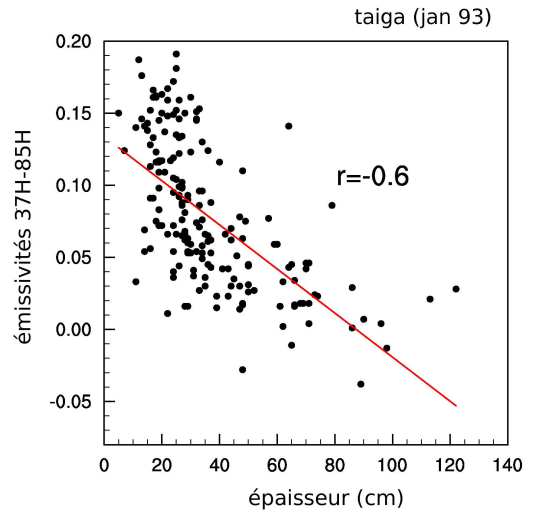
FIG. 5.6: Le comportement de la différence d'émissivités à 37 GHz-H et à 85 GHz-H avec l'épaisseur. Les données sont limitées au mois de janvier 93 sur les zones de taïga.
