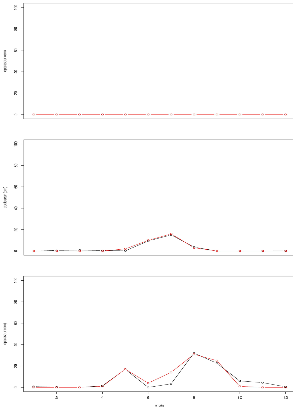
FIG. 5.33: Exemples de séries temporelles en trois points pour lesquels l'inversion par RNA (en noir) est satisfaisante par rapport aux mesures in situ (en rouge). Ces points sont respectivement, de haut en bas, localisés en (53,5^{\circ}E : 40,5^{\circ}N) , (45,5^{\circ}E : 43,5^{\circ}N) , (30,5^{\circ}E : 61,5^{\circ}N) .
