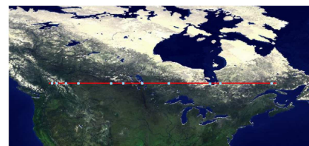
FIG. 4.3: La position de la coupe et des stations canadiennes où ont été relevées les épaisseurs du manteau.(image MODIS/Terra)
