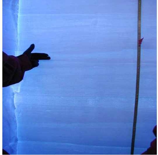
FIG. 1.5: Structure en couches du manteau neigeux observé par transparence. Leur luminosité dépend de leur surface spécifique, i.e. la surface totale d'adsorption ( Cabanes et al. (2003); Hoff et al. (1998) ). (image www.stolaf.edu/other/cegsic/itase )
