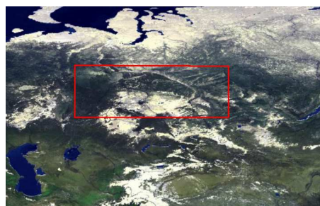
FIG. 4.6: La localisation de la zone utilisée pour les histogrammes de la figure 4.7. (image MODIS/Terra)
