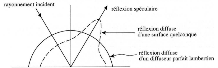
FIG. 2.4: Indicatrice de réflexion illustrant les notions de surfaces spéculaire et lambertienne. ( Bonn and Rochon (1992))
