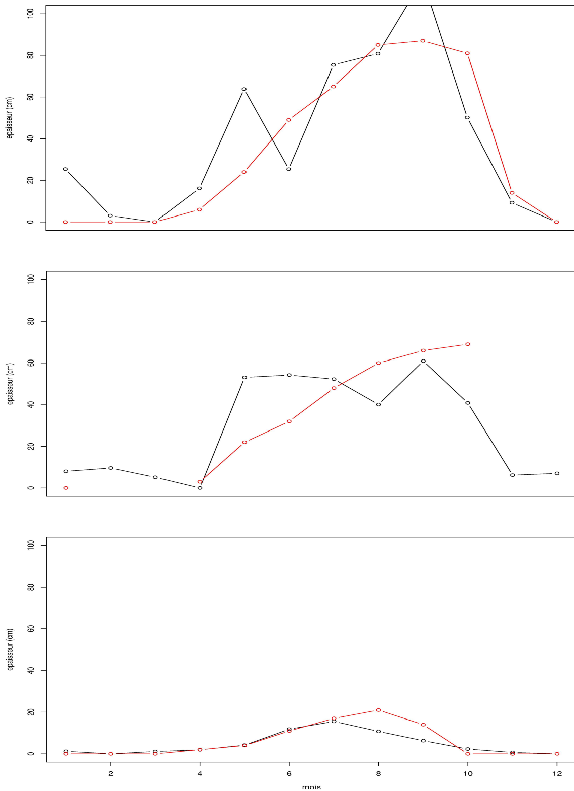
FIG. 5.32: Exemples de séries temporelles en trois points pour lesquels l'inversion par RNA (en noir) n'est pas satisfaisante par rapport aux mesures in situ (en rouge). Ces points sont respectivement, de haut en bas, localisés en (47,5^\circ E : 64,5^\circ N) , (32,5^\circ E : 67,5^\circ N) , (129,5^\circ E : 52,5^\circ N) .
