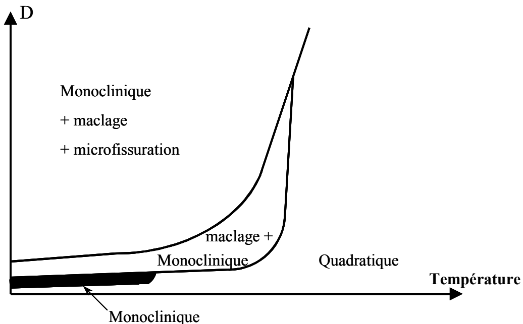
Figure II.8. Domaines de transformation des particules de zirconite en fonction de leur diamètre D [FAN88]
