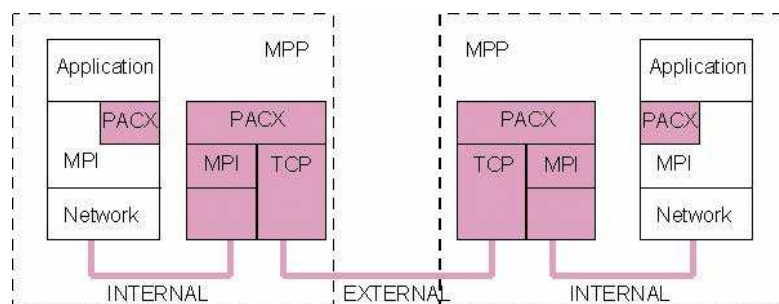
FIG. 2.7 – PACX-MPI [45].
