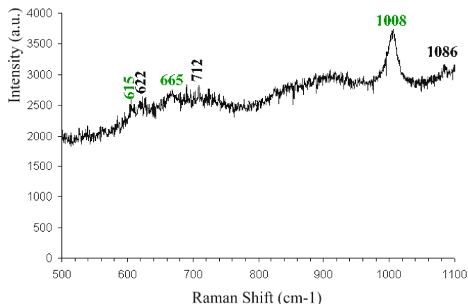
Figure IV-9: Spectre de diffusion Raman obtenu dans la couche incolore superficielle de l'échantillon 21LCF, montrant les pics principaux du gypse (en vert) et de la calcite (en noir). \lambda=647,1 nm ; G=200 ; P=2 mW ; t=60 sec., 4 acq.
