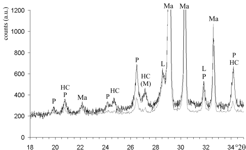
Figure III-7: Diffractogramme sur poudre de l'échantillon de Litharge (Laverdure) avant (en gris) et après le test T2 (en noir) dans l'intervalle [18-34]^{\circ}2\theta , mettant en évidence l'augmentation de la proportion en plumbonacrite (P) et en hydrocérusite (HC). Pics du massicot (Ma) et de la litharge (L).
