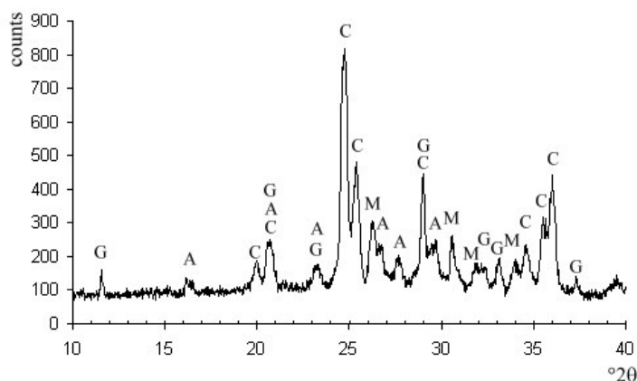
Figure IV-46: Diffractogramme obtenu en surface de l'échantillon 13LCF010, montrant la présence de gypse CaSO_4 \cdot 2H_2O (G), de cérusite PbCO_3 (C), d'anglésite PbSO_4 (A) et de minium Pb_3O_4 (M).
