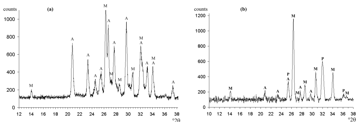
Figure IV-69: (a) Diffractogramme obtenu en surface de l'échantillon 13LCS013, montrant la présence majoritaire de l'anglésite PbSO_4 (A) et du minium Pb_3O_4 (M). (b) Diffractogramme de la coupe transversale de 13LCS013. Pics de la plattnélite \beta - PbO_2 (P), du minium Pb_3O_4 (M) et de l'anglésite PbSO_4 (A).
