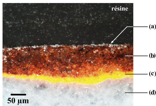
Figure IV-7: Observation en microscopie optique de la stratigraphie de l'échantillon 21LCF (x 200).
