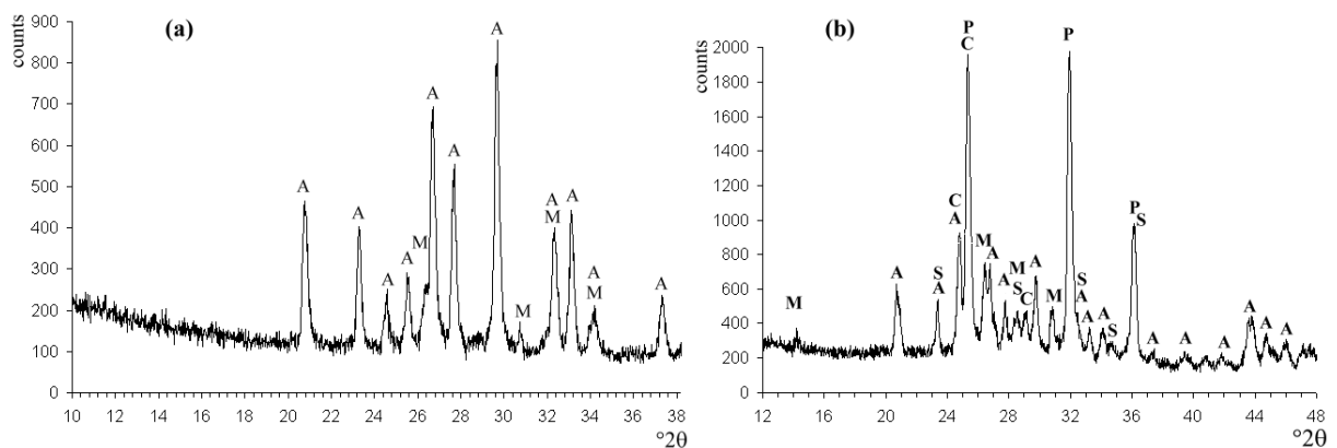
Figure IV-55: (a) Diffractogramme obtenu en surface de l'échantillon 11DF06 montrant la présence majoritaire d'anglésite PbSO_4 (A) et de minium Pb_3O_4 (M). (b) Diffractogramme obtenu en mode « focalisé » sur la coupe transversale, montrant les pics de la plattnérite \beta-PbO_2 (P) et de la calcite CaCO_3 (C). Position des pics les plus intenses de la scrutinyite \alpha-PbO_2 (S).
