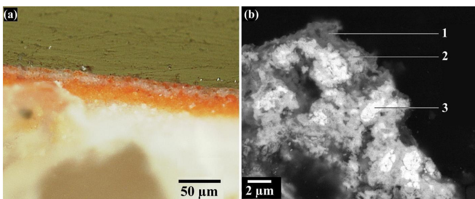
Figure IV-29: (a) Vue en microscopie photonique de la coupe transversale de 13F08 (x200). (b) Vue en microscopie électronique à balayage (électrons rétrodiffusés) de la couche supérieure, constituée de trois phases caractéristiques (1 : gypse ; 2 : anglésite/cérusite ; 3 : minium).
