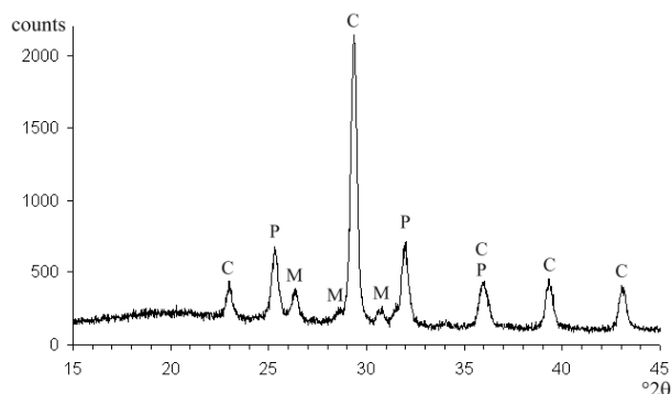
Figure IV-42: Diffractogramme de la couche picturale de l'échantillon 13LCF09 obtenu en mode "focalisé", montrant la présence de calcite \text{CaCO}_3 (C), de plattnérite \beta\text{-PbO}_2 (P) et de minium \text{Pb}_3\text{O}_4 (M).
