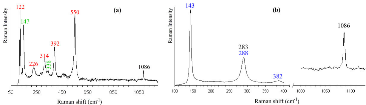
Figure III-28: Spectres de diffusion Raman obtenus ponctuellement en surface de la couche d'altération de l'éprouvette E1. (a) zones de couleur rouge-orangé, présentant les pics de Pb_3O_4 (en rouge), de la litharge \alpha - PbO (en vert) et de la calcite CaCO_3 (en noir); (b) zones de couleur vert-jaune: pics du massicot \beta - PbO (en bleu) et de la calcite (en noir). Conditions d'acquisition: \lambda=785nm , P=0,25mW , 40sec \times 4acc .
