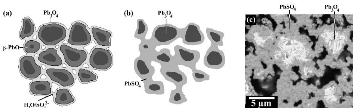
Figure IV-81: Représentation schématique de l'altération de grains de Minium en milieu humide sulfaté. (a) Mouillage des grains de pigment synthétisés à température excessive par une solution diluée d'acide sulfurique. (b) Structure des grains après sulfatation du massicot présent en périphérie. (c) Image d'électrons rétrodiffusés (échantillon 11DF06, couche supérieure).
