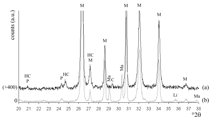
Figure III-2: Diffractogramme sur poudre de l'échantillon T1-2 dans l'intervalle [20-38]^\circ 2\theta (a), comparé au diffractogramme de référence du Minium de marque Laverdure (b). Pics de la plumbonacrite (P), de l'hydrocérusite (HC), du minium Pb_3O_4 (M), de la litharge (L), du massicot (Ma) et de la calcite (C).
