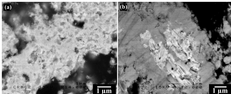
Figure IV-60: Vue en microscopie électronique à balayage (électrons rétrodiffusés) des constituants des couches d'altération de l'échantillon 11DF011. (a) Couche noire, x14000. (b) Couche incolore, x12000.
