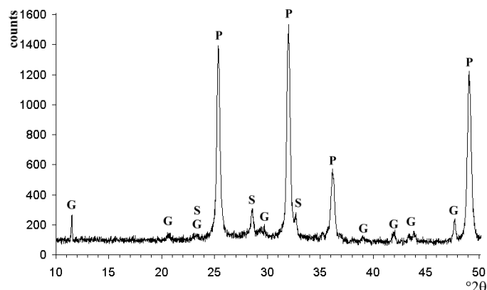
Figure IV-32: Diffractogramme obtenu en surface de l'échantillon 11LCF03 dans l'intervalle angulaire [10-50]^\circ 2\theta . Pics de la plattnérite \beta\text{-PbO}_2 , (P) du gypse \text{CaSO}_4 \cdot 2\text{H}_2\text{O} (G) et de la scrutinyte \alpha\text{-PbO}_2 (S).
