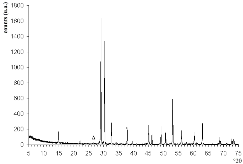
Figure VI-3: Diffractogramme sur poudre du Massicot de marque Laverdure. Pics de Pb 3 O 4 (Δ)
