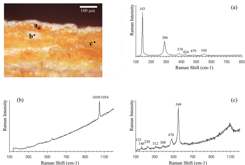
Figure IV-95: Spectres de diffusion Raman de certaines zones caractéristiques de la coupe transversale M2. (a) Grain orange, composé de massicot \beta -PbO et de minium Pb_3O_4 . (b) Grain incolore d'hydrocérusite 2PbCO_3 \cdot Pb(OH)_2 (c) Grain de couleur jaune-orangé, composé de minium Pb_3O_4 et de litharge \alpha -PbO. \lambda=514 \text{ nm} , P=0,2 \text{ mW} , 10 \text{ sec.} , 4 \text{ acc.} , \times 500 .
