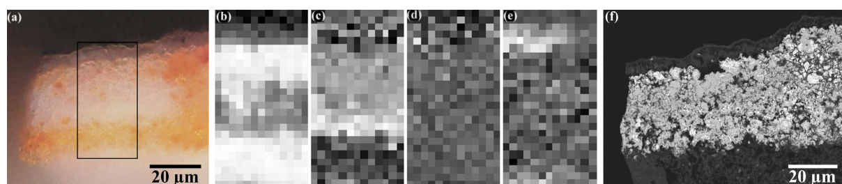
Figure IV-37: (a) Vue en microscopie photonique de la zone de 11LCF04 cartographiée par spectrométrie Raman. Cartographies (12 x 24 points) de la zone caractéristique. (b) minium \text{Pb}_3\text{O}_4 ; (c) cérusite \text{PbCO}_3 ; (d) anglésite \text{PbSO}_4 ; (e) calcite \text{CaCO}_3 . (f) Vue en microscopie électronique à balayage de la même zone (électrons rétrodiffusés, x 950).
