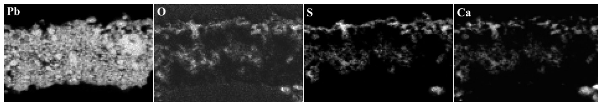
Figure IV-34: Cartographies élémentaires du plomb, de l'oxygène, du soufre et du calcium obtenues par microsonde électronique au sein de la coupe transversale de l'échantillon 11LCF03 (120 \mu m x 80 \mu m). Pas latéral: 1 \mu m.
