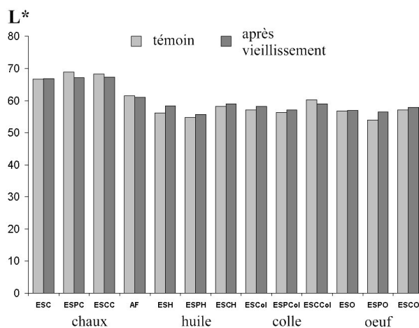
Figure III-31: Eprouvettes au Minium : Valeurs de la clarté L* mesurée par spectrophotométrie en réflectance diffuse à la surface des éprouvettes témoin (en gris clair) et après vieillissement artificiel (en gris foncé).
