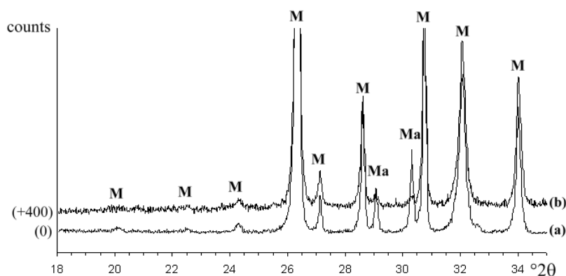
Figure III-8: Diffractogramme sur poudre de l'échantillon de Minium avant (a) et après (b) le test T2, montrant la forte diminution de la proportion de massicot (Ma). M: pics du minium Pb_3O_4 .
