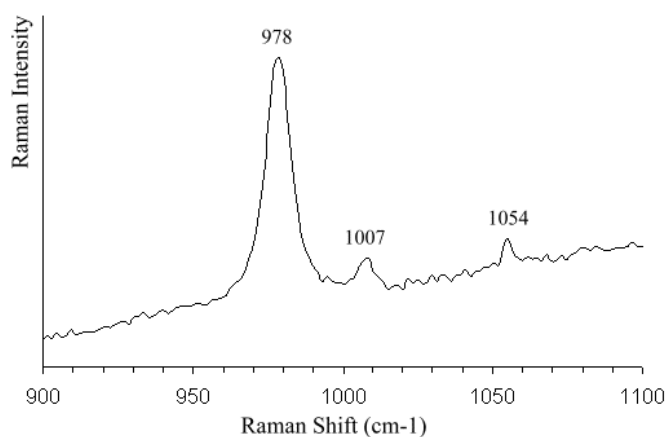
Figure IV-26: Spectre Raman obtenu en surface de l'échantillon 13F07 (couche superficielle blanche), comportant les pics de l'anglésite \text{PbSO}_4 ( 978\text{ cm}^{-1} ), du gypse \text{CaSO}_4 \cdot 2\text{H}_2\text{O} ( 1007\text{ cm}^{-1} ) et de la cérusite \text{PbCO}_3 ( 1054\text{ cm}^{-1} ). \lambda=514\text{ cm}^{-1} , P=2\text{ mW} , 20\text{ sec} . \times 4\text{ acc.} , G=\times 500 .
