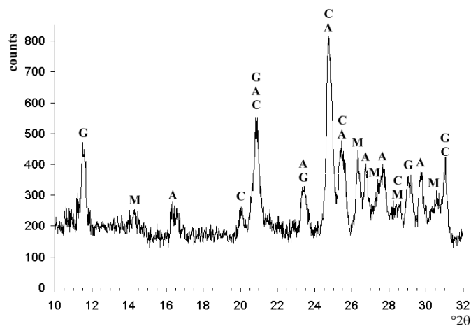
Figure IV-36 : Diffractogramme obtenu en surface de l'échantillon 11LCF04 dans l'intervalle angulaire [18-32]^\circ 2\theta , montrant la présence de gypse CaSO_4 \cdot 2H_2O (G), de cérusite PbCO_3 (C), d'anglésite PbSO_4 (A) et de minium Pb_3O_4 (M).
