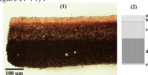
Figure IV-74: (1) Vue en microscopie photonique de la coupe transversale de l'échantillon 13LCS014 (x200). (2) Succession stratigraphique.
