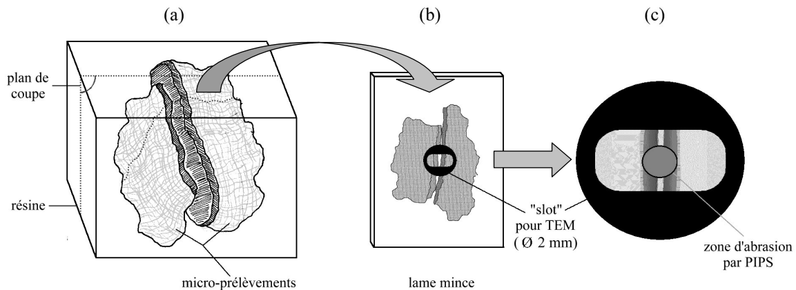
Figure II-13: Préparation d'un échantillon avant l'amincissement ionique par PIPS. (a) Enrobage des micro-prélèvements et coupe transversale. (b) Transfert de la coupe sur un support de verre et fabrication d'une lame mince (30 \mu\text{m} ). (c) Transfert sur un porte échantillon de type "slot" pour TEM.
