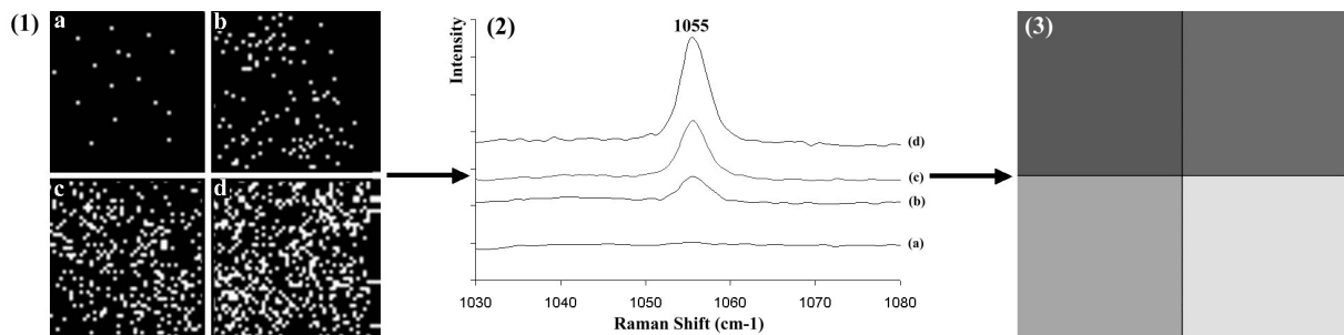
Figure II-7: Principe de la cartographie Raman (2 x 2 points) d'un échantillon hétérogène basé sur le calcul de l'aire d'un pic de référence. (1) Représentation schématique de la répartition du composé de référence (représenté en blanc). (2) Spectres obtenus dans les quatre cellules (pic principal à 1055 \text{cm}^{-1} ). (3) Carte de répartition semi-quantitative obtenue après calcul des intensités intégrées dans l'intervalle [1030-1080] \text{cm}^{-1} .
