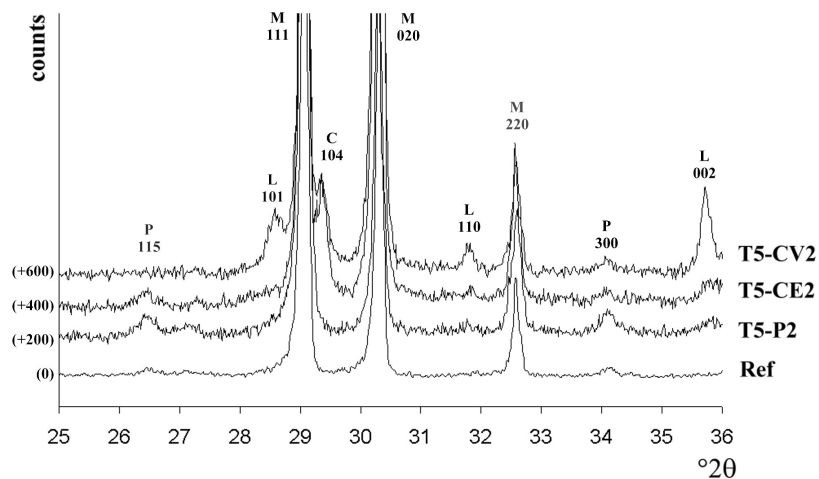
Figure III-18: Diffractogrammes sur poudre des échantillons T5-P2, T5-CE2 et T5-CV2 comparés au diffractogramme de référence de la massicot (Laverdure) dans l'intervalle [25-36]^{\circ}2\theta . Pics de la plumbonacrite (P), de la litharge (L), du massicot (M) et de la calcite (C).
