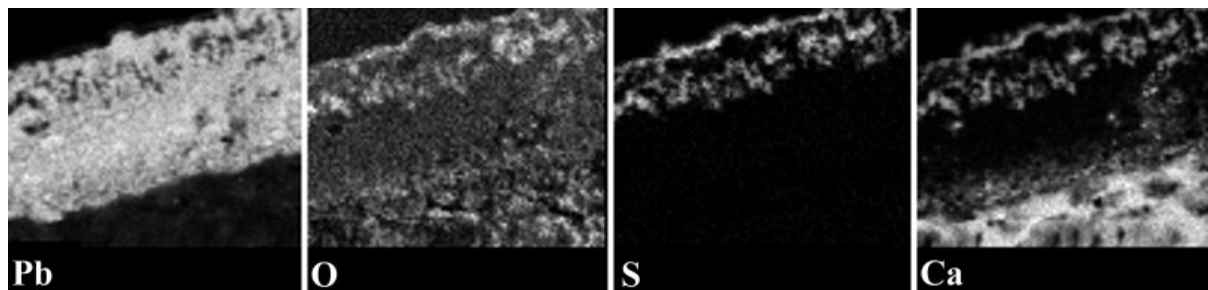
Figure IV-43: Cartographies élémentaires du plomb, de l'oxygène, du soufre et du calcium obtenues par microsonde électronique au sein de la coupe transversale de l'échantillon 13LCF09 ( 100\mu\text{m} \times 80\mu\text{m} ). Pas latéral : 1\mu\text{m} .
