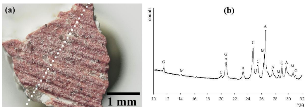
Figure IV-28: (a) Vue à la loupe binoculaire (x25) de la surface de l'échantillon 13F08 et lieu de la coupe transversale (ligne pointillée). (b) Diffractogramme obtenu en surface de l'échantillon dans l'intervalle [10\text{-}32]^\circ 2\theta , montrant la présence de gypse (G), de minium \text{Pb}_3\text{O}_4 (M), d'anglésite \text{PbSO}_4 (A) et de cérusite \text{PbCO}_3 (C).
