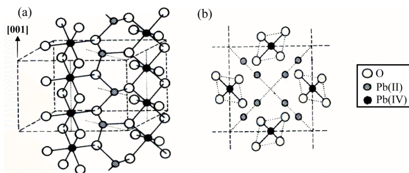
Figure I-3: Représentation de la maille élémentaire de l'orthoplombate de plomb Pb_3O_4 , (a) dans l'espace ; (b) en projection sur le plan (001).
