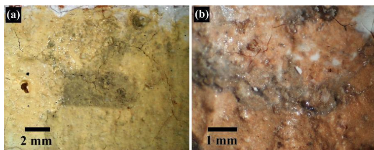
Figure III-41: Vue à la loupe binoculaire de la couche picturale de l'éprouvette E2. (a) Massicot, obscurcissement de la zone irradiée (au centre). (b) Litharge, obscurcissement localisé dans les dépressions de la couche picturale. Grandissements \times 20 et \times 47 respectivement.
