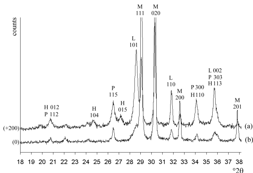
Figure III-5: Diffractogramme de l'échantillon T1-5 dans l'intervalle [18-38]^\circ 2\theta (a), comparé au diffractogramme de référence de l'oxyde PbO Merck pur (b). Pics de l'hydrocérusite (H), de la plumbonacrite (P), du massicot (M) et de la litharge (L).
