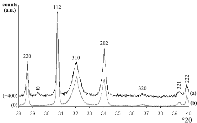
Figure III-1: Diffractogramme sur poudre de l'échantillon T1-1 dans l'intervalle [20-38]^\circ 2\theta (a), comparé au diffractogramme de référence de Pb_3O_4 (b). hkl: réflexions sur les plans réticulaires de Pb_3O_4 . *Réflexion sur la famille de plans (104) de la calcite CaCO_3 .
