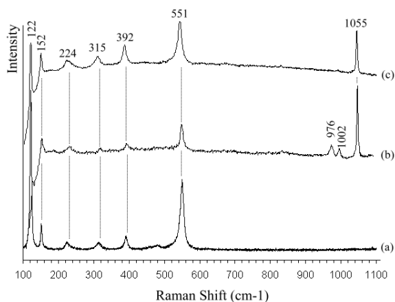
Figure IV-64: Spectres Raman obtenus dans la coupe transversale de l'échantillon 13DF012. (a) Couche inférieure rouge ( \lambda=514\text{ nm} , P=2\text{mW} , 10 sec., 4 acc., x500) (b) Spectre obtenu à l'interface entre la couche supérieure blanche et la résine d'enrobage ( \lambda=514\text{ nm} , P=1\text{mW} , 20 sec., 4 acc., x500). (c) Spectre caractéristique de la couche supérieure blanche (514 nm, P=2\text{mW} , 10 sec., 4 acc., x500). Echelle verticale arbitraire.
