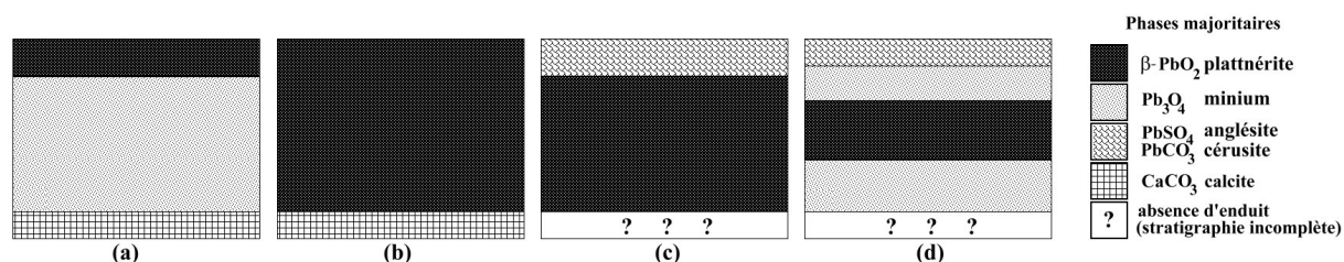
Figure IV-83: Représentation schématique des différentes stratigraphies caractéristiques observées dans les échantillons contenant de la plattnérite \beta-PbO_2 . (a) 13LCF09, 13DF011; (b) 11LCF03, 11DF05; (c) 11F01, 11F07; (d) 11DF06, 13LCS013, 13LCS014.
