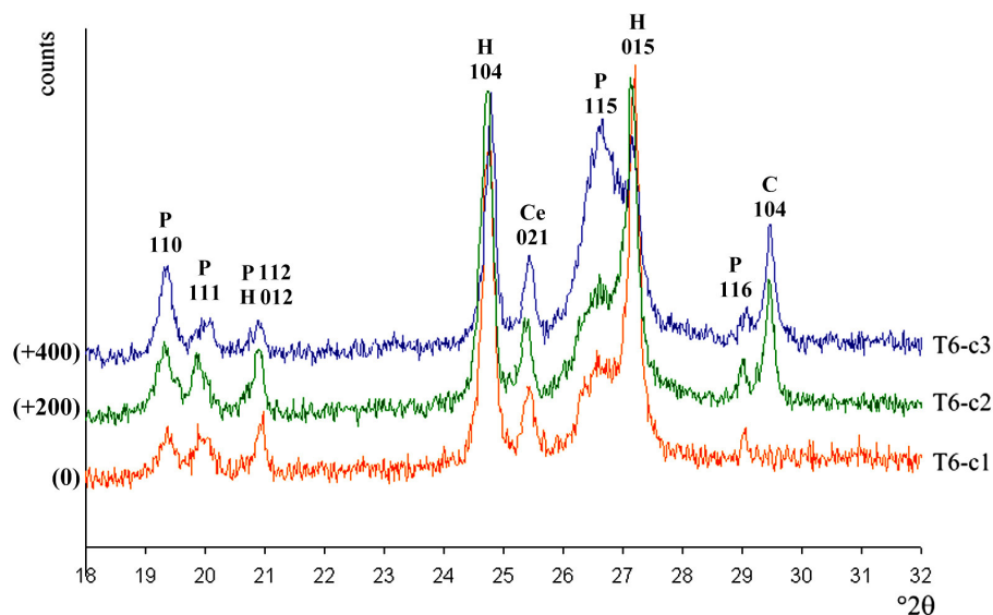
Figure III-23: Diffractogrammes sur poudre dans l'intervalle [18-32]^\circ 2\theta des échantillons T6-c1 (en orange), T6-c2 (en vert) et T6-c3 (en bleu) après le test. Pics de la plumbonacrite (P), de l'hydrocérusite (H), de la cérusite (Ce) et de la calcite (C).
