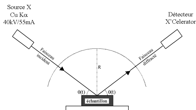
Figure II-3: Schéma du principe de l'analyse d'un échantillon massif en Diffraction de Rayons X en configuration "Bragg-Brentano" \theta-\theta .
