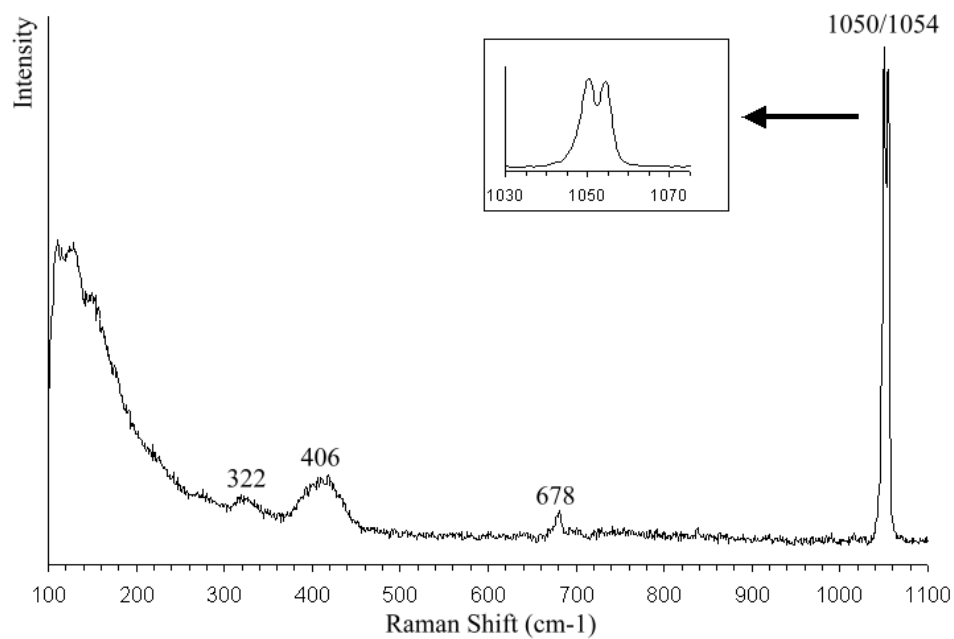
Figure VI-8: Spectre Raman du Blanc de Plomb de marque Laverdure. \lambda=514 nm, P=10 mW, T=5 sec., 4 acc., x200.
