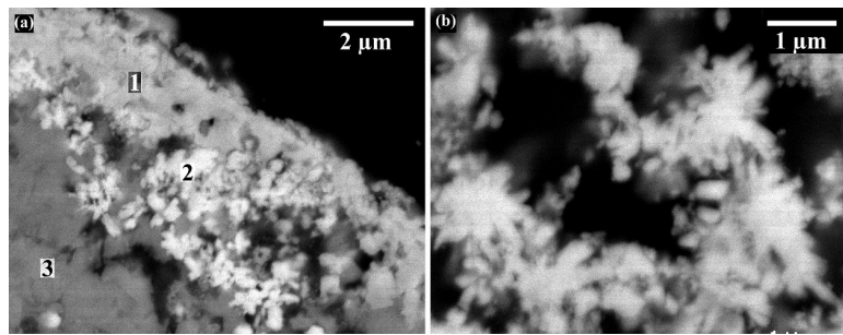
Figure IV-53: Vues au MEB de la coupe 11DF05. (a) Zone supérieure (x10000): couche superficielle d'anglésite PbSO_4 et/ou de cérusite PbCO_3 (1), des grains de plattnérite \beta-PbO_2 (2) et des cristaux de gypse CaSO_4 \cdot 2H_2O (3). (b) Détail des grains de plattnérite (x15000).
