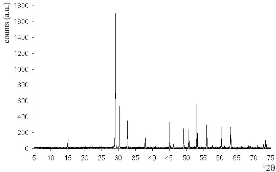
Figure VI-19: Diffractogramme sur poudre de la plattn rite cuite   616 C pendant 10 heures, montrant l'ensemble des pics du massicot ( \beta -PbO).
