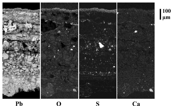
Figure IV-93: Cartographies élémentaires (plomb, soufre, calcium et oxygène) obtenues par microsonde électronique dans la section transversale de l'échantillon M2 (350μm x 900μm). Pas latéral: 1 μm.
