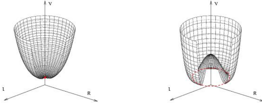
FIG. I.2.1 – Représentation simplifiée du potentiel de Higgs, pour \Phi = \varphi_3 + i\varphi_4 : à gauche, si \mu^2 > 0 , le minimum est atteint en un point ; à droite, si \mu^2 < 0 , le minimum définit un cercle dans le plan complexe
