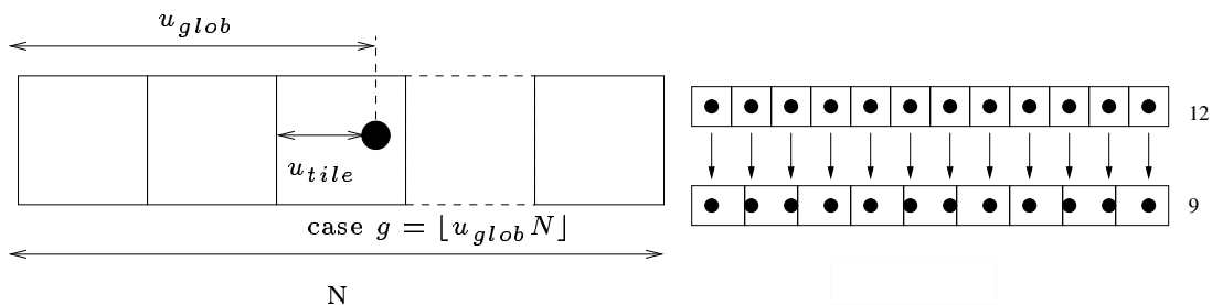
(a) Le composant Pavage virtuel calcule la position du point aux coordonnées u_{glob} dans la grille virtuelle de taille N .
