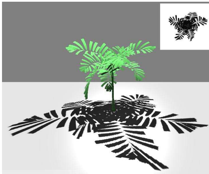
FIG. 5.3 – Carte d'ombre.
