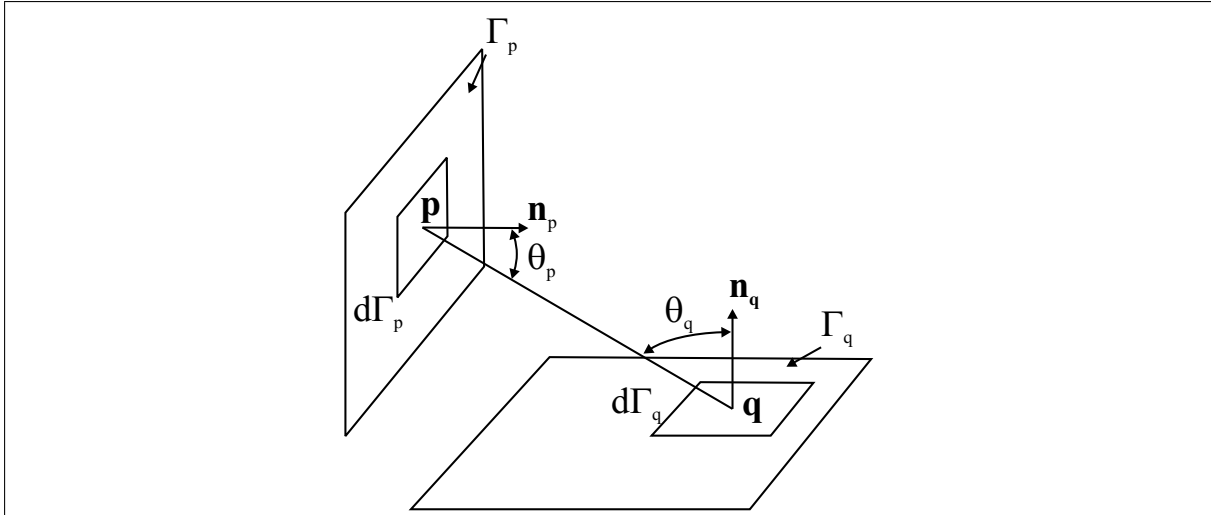
Fig. III.3 – Le facteur d'angle entre les surfaces d\Gamma_p et d\Gamma_q est une quantité purement géométrique qui dépend des formes et des positions respectives des deux surfaces.
