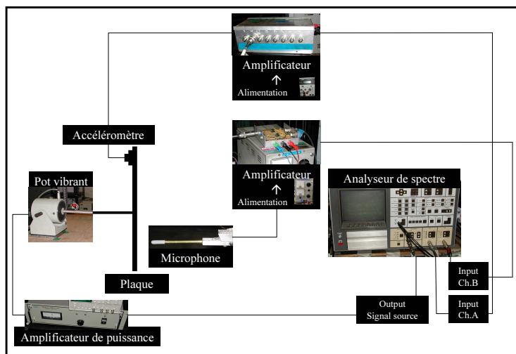
Fig. V.14 – Schéma du dispositif expérimental.
