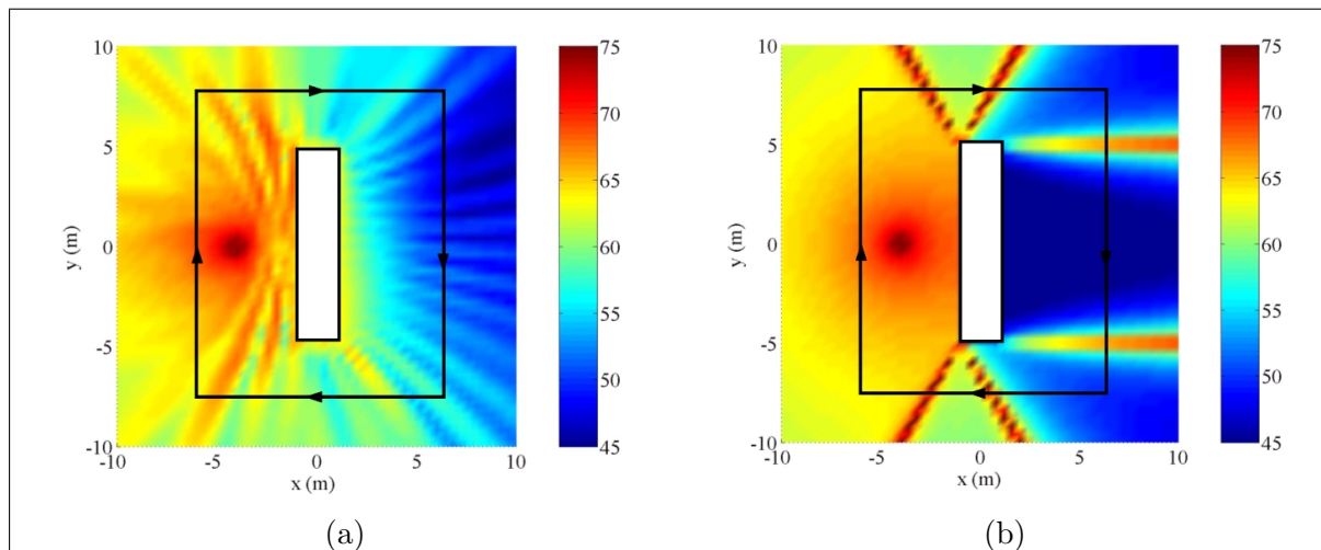
Fig. IV.18 – Diffraction d'une source cylindrique par une barrière rectangulaire de dimensions 10\text{ m} \times 2\text{ m} . L_p (dB - ref : 2.10^{-5}\text{ Pa} ) autour de la barrière calculé par (a) la BEM et (b) la méthode du transfert radiatif. L'étude est menée sur le tiers d'octave centré sur 250 Hz.
