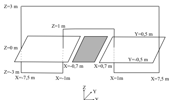
Fig. VI.21 – Plans de calcul acoustique du bruit rayonné par la transmission : les calculs sont menés sur un plan double parallèle et situé de part et d'autre de la face supérieure du carter, et sur un plan perpendiculaire à la face.
