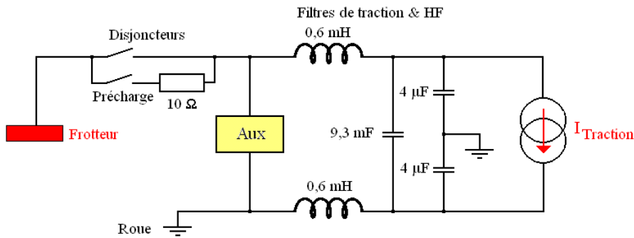
Figure 4-21 : Schéma équivalent du tramway CITADIS 302
