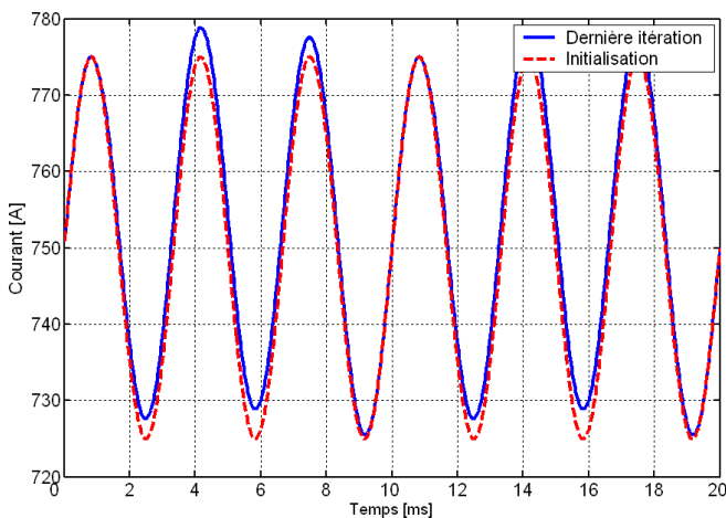
Figure 5-18 : Allure temporelle de I_{dc}
