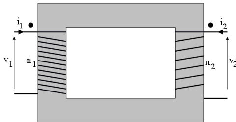
Figure III-1 : Transformateur à deux enroulements
