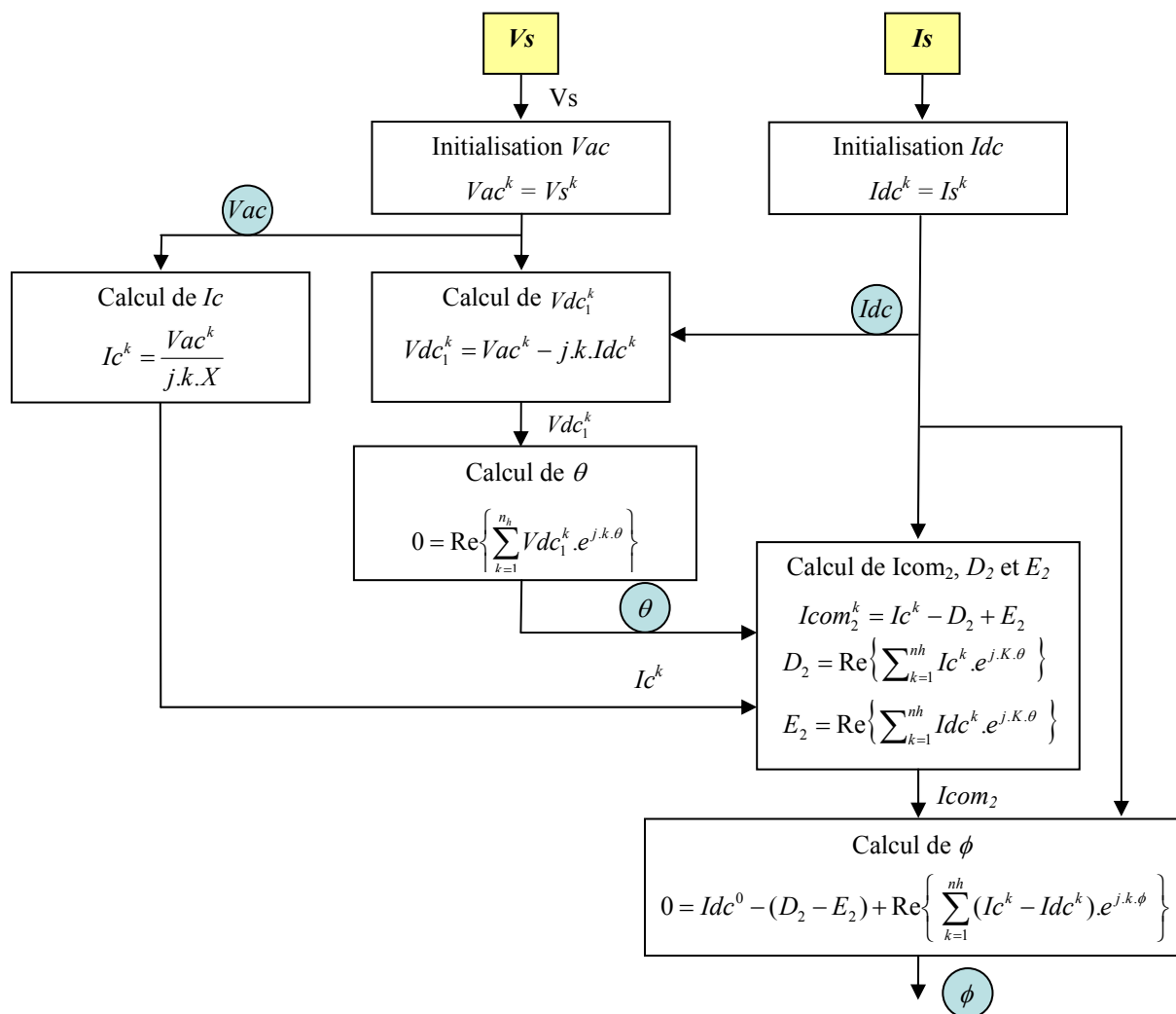
Figure 5-10 : Principe d'initialisation des inconnues V_{ac} , I_{dc} , \theta et \phi
