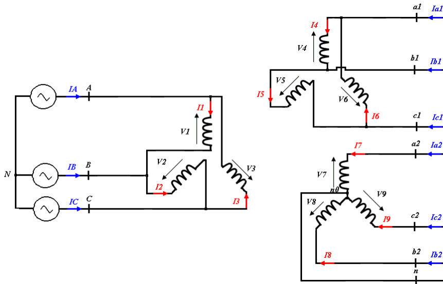
Figure 3-19 : Couplage Ddy_n d'un transformateur
