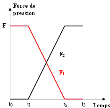
Figure 4-6 : Evolution des efforts de pression lors de la transition
