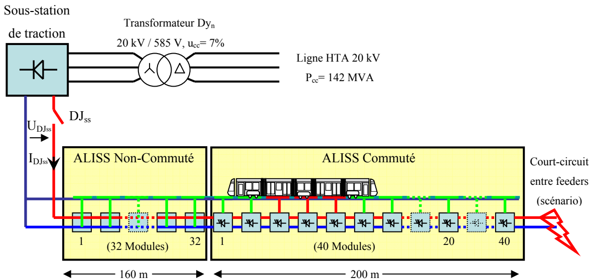
Figure 4-23 : Schéma de référence pour l'ensemble des simulations dynamiques sur la ligne de la Rochelle
