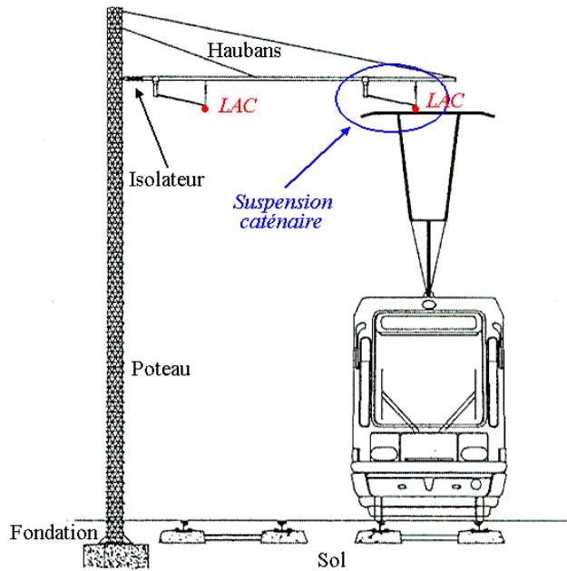
Figure 1-7 : Support latéral d'une ligne aérienne de contact
