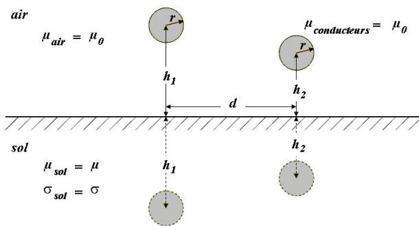
Figure 2-17 : Deux conducteurs cylindriques au dessus d'un sol conducteur
