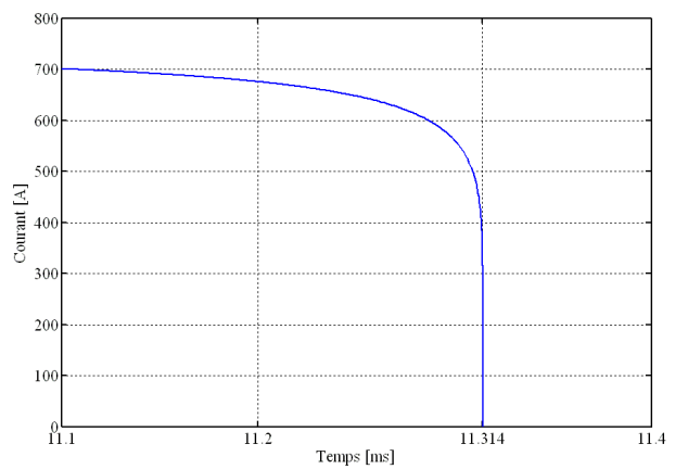
Figure 4-11 : Zoom sur l'évolution du courant i_1(t) durant les derniers instants de transition
