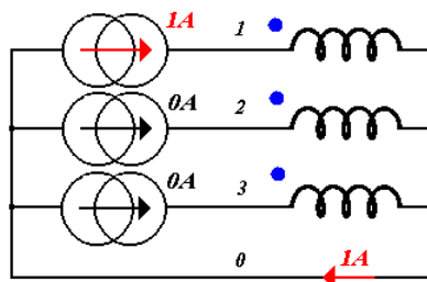
Figure 3-3 : Boucle de courant entre les conducteurs 1 et 0
