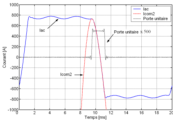
Figure 5-12 : Illustration de I_{ac} et de I_{com2} avec le bon angle \phi
