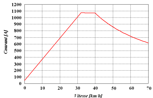
Figure 1-5 : Courant de traction d'un CITADIS 302 en fonction de sa vitesse
