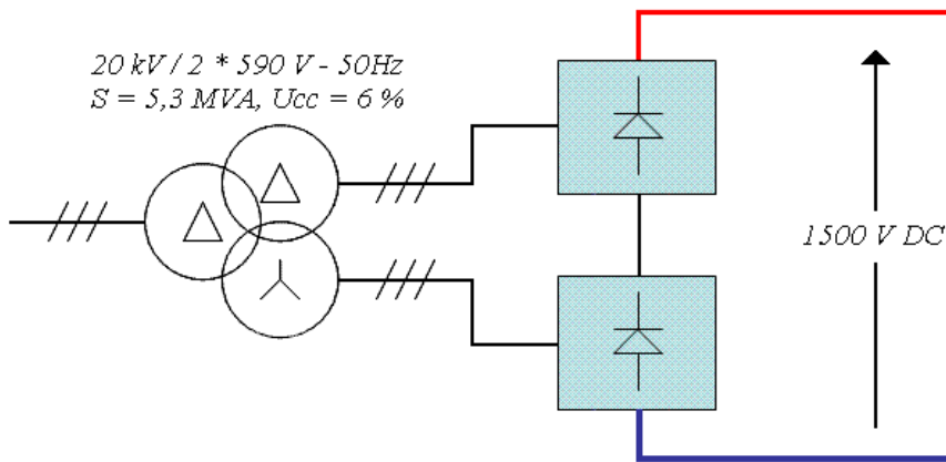
Figure 3-20 : Association série de deux ponts redresseurs, site de Valenciennes
