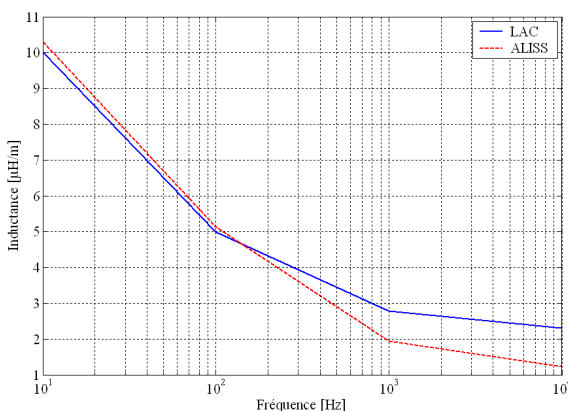
Figure 3-15 : Evolution des inductances Feeder positif / Rail avec la fréquence, sur les structures LAC et ALISS
