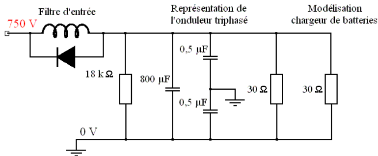
Figure 4-22 : Schéma équivalent des auxiliaires du tramway CITADIS 302
