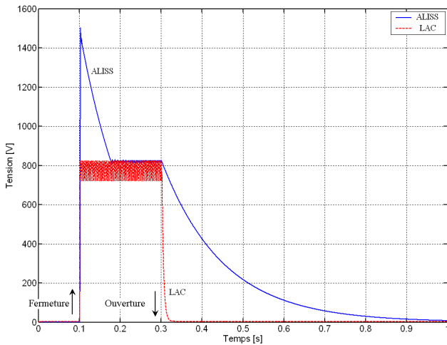
Figure 4-24 : Tension en sortie du disjoncteur de sous-station
