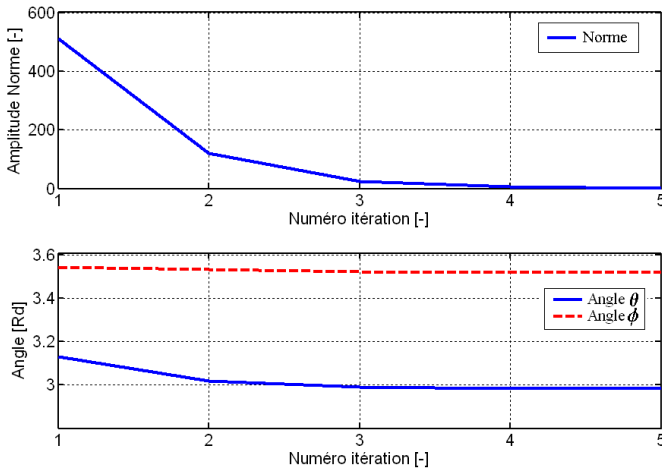
Figure 5-20 : Evolution de la norme de f(X_n) et des angles de conductions des diodes avec les itérations
