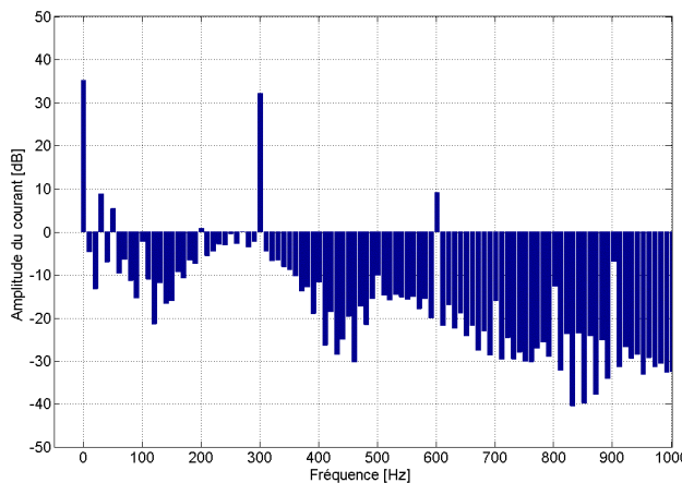
Figure 4-30 : FFT du courant de la sous-station entre les instants t = 0,65 s et t = 0,75 s
