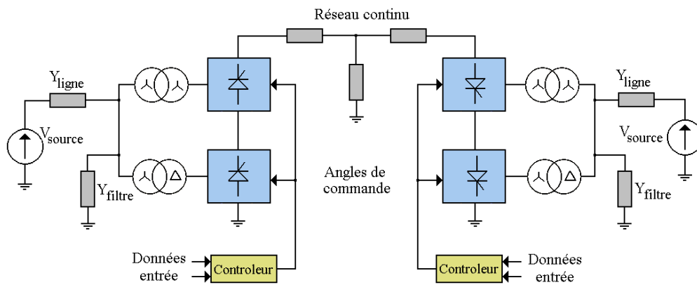
Figure 2-10 : Exemple de liaison HVDC – Schéma unifilaire
