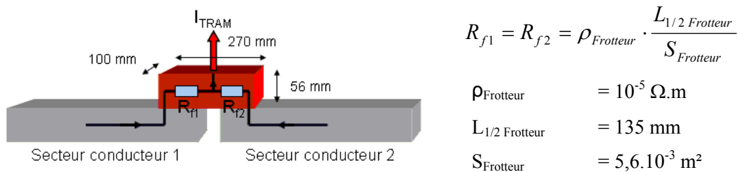
Figure 4-9 : Calcul des résistances R_{f1} et R_{f2}
