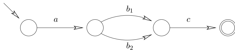
FIG. 2.3 – Automate des observations pour des observations incertaines
