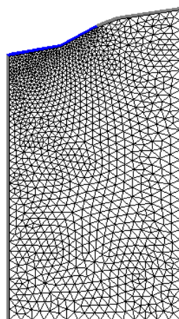
FIG. 1.2.3 – Maillage et conditions aux limites d'HYDRUS-2D en irrigation à la raie
