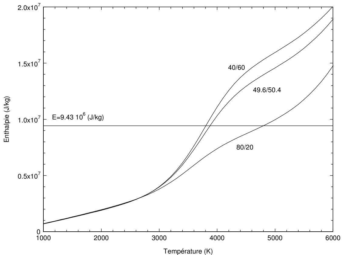
Fig. 5. : Enthalpie en fonction de la température pour plusieurs mélanges de gaz (P=1 atm., θ=1).
