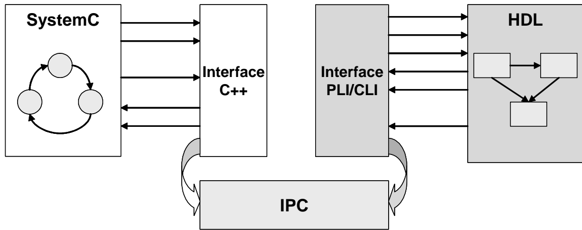
Figure 4. 3 : L'environnement de covérification de HDL et de SystemC.
