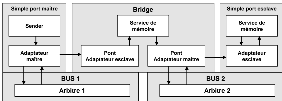
Figure 2.8 : Modèle fonctionnel des services de communication du STBus.
