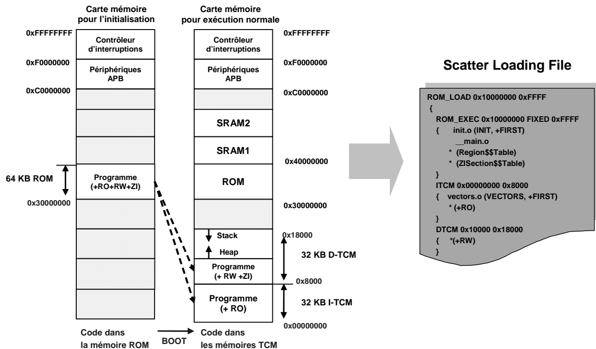
Figure 5.20 : L'implémentation de carte mémoire.
