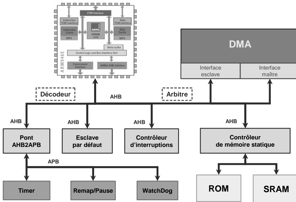
Figure 5.10 : L'architecture du sous-système VLC.
