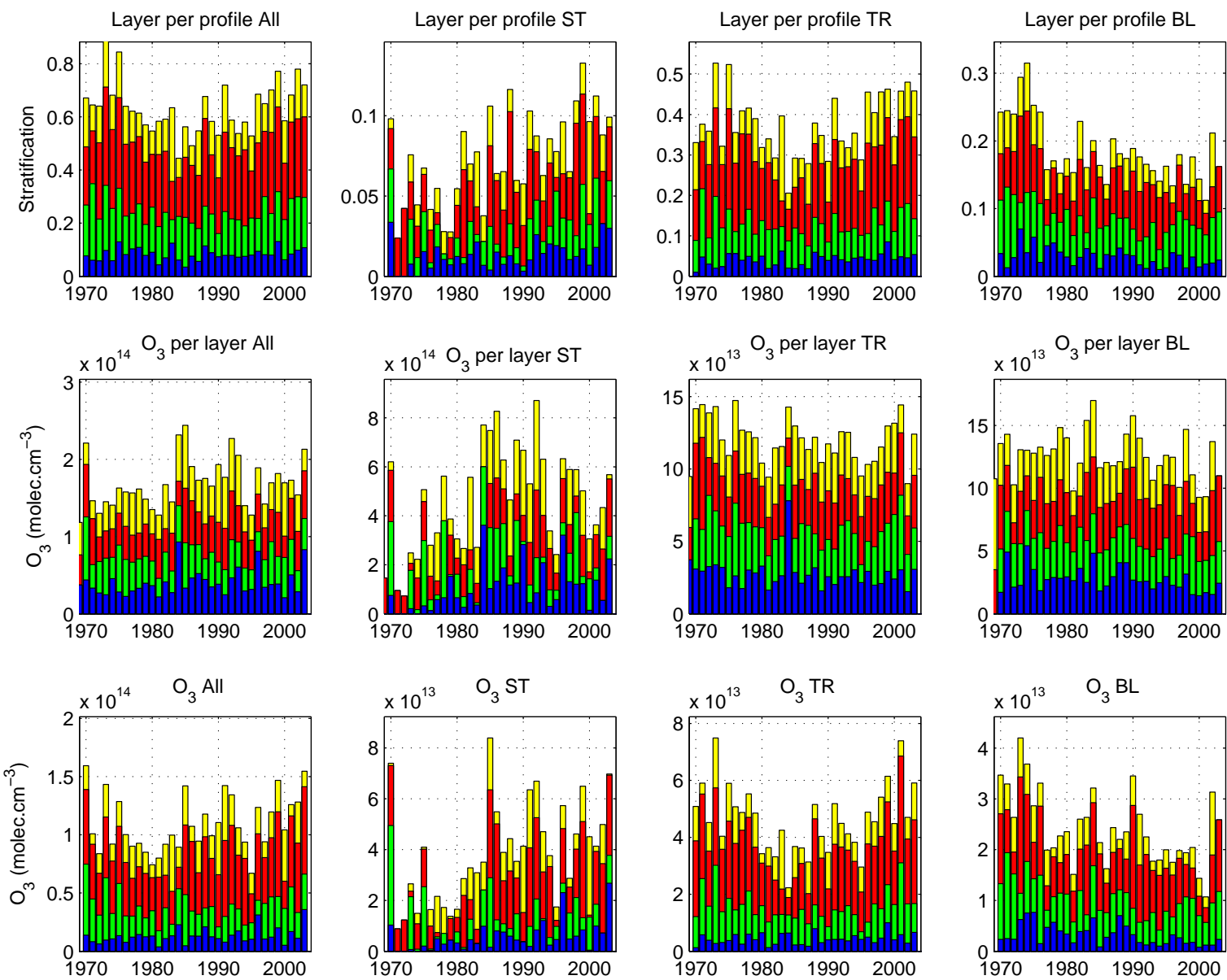
FIG. 3.14 – Tendances à long terme de la stratification en ozone à Uccle et Hohenpeißenberg. 1 ère colonne : ensemble des couches, colonnes suivantes : couches ST, TR et CL (BL pour boundary layer). 1 ère ligne : nombre de couches par profil ; 2 ème ligne : contenu moyen en ozone des couches ; 3 ème ligne : ozone total mesuré dans les couches troposphérique Les couleurs indiquent la saison (bleu : DJF, vert : MMA, rouge : JJA, jaune : SON).
