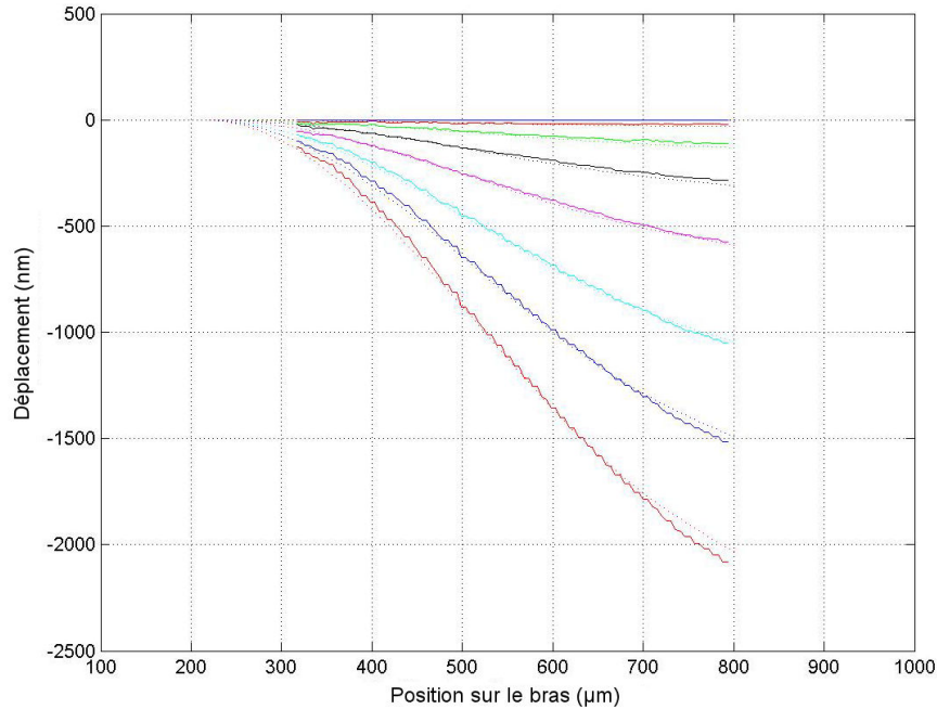
Figure 5-29 Profil le long d'un bras pour différentes tensions
