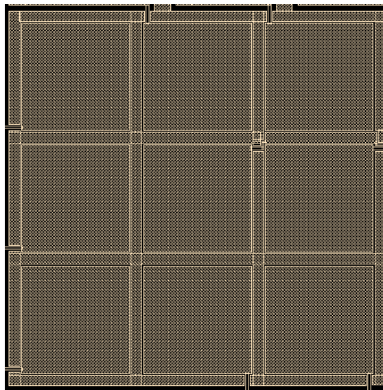
Figure 6-2 Masque de la couche Poly0 (électrodes)
