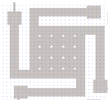
Figure 2-24 Masque de la couche métallique supérieure pour un actionneur
