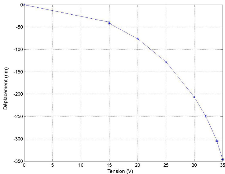
Figure 6-10 Courbe d'actionnement pour l'actionneur central
