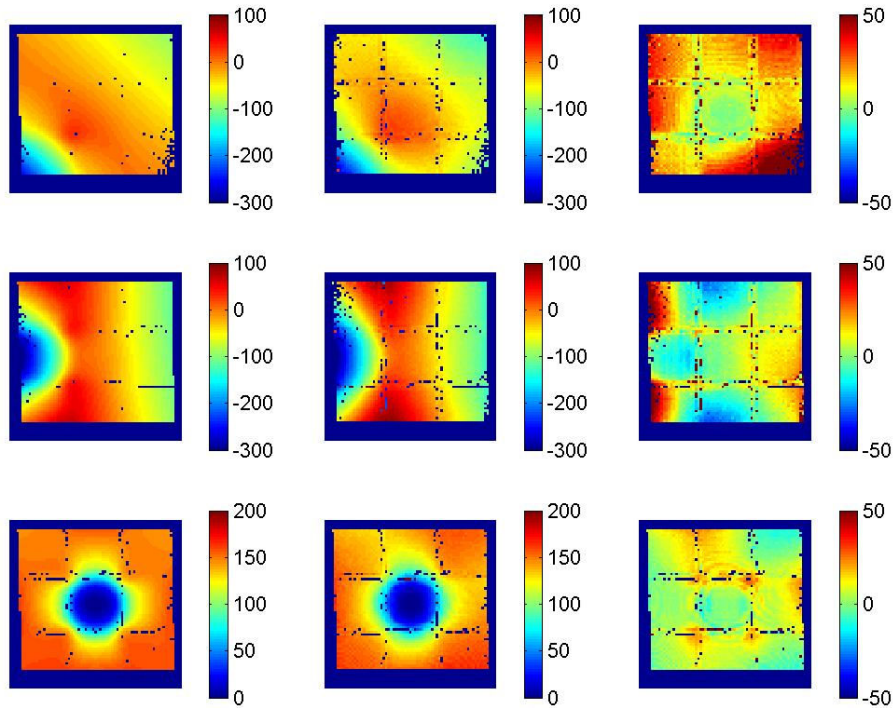
Figure 6-21 Comparaison simulation/caractérisation pour le prototype PolyMUMPS modèle « plaque » en présence de contacts dans le composant Gauche : Cartes mesurées expérimentalement Centre : Cartes simulées par éléments finis (modèle « plaque ») Droite : Différence entre les deux séries de cartes Haut : Comparaison actionneur d'un coin Milieu : Comparaison actionneur latéral Bas : Comparaison actionneur central
