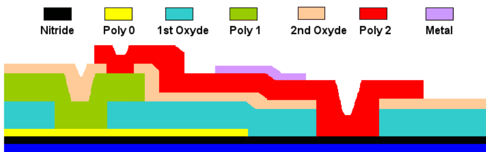
Figure 2-20 Procédé PolyMUMPS de Memscap
