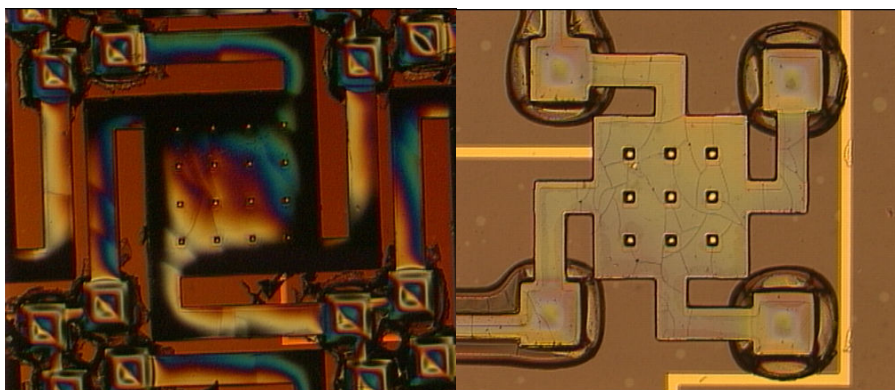
Figure 5-22 Actionneurs avec un plateau de 580\mu\text{m} (gauche) de 300\mu\text{m} (droite)
