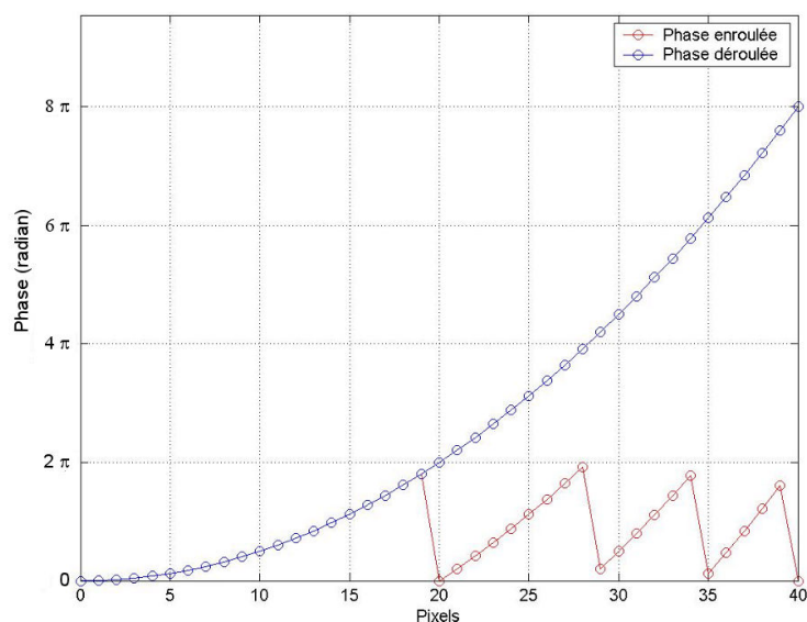
Figure 4-26 Exemple de déroulement de phase mono-dimensionnel
