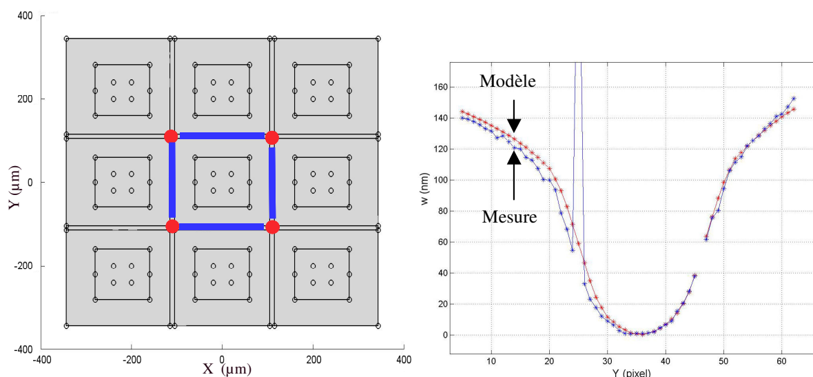
Figure 6-20 Modélisation « plaque » du prototype avec des contacts Gauche : Géométrie de la simulation, les points rouges et les barres bleues représentent les zones de contact
