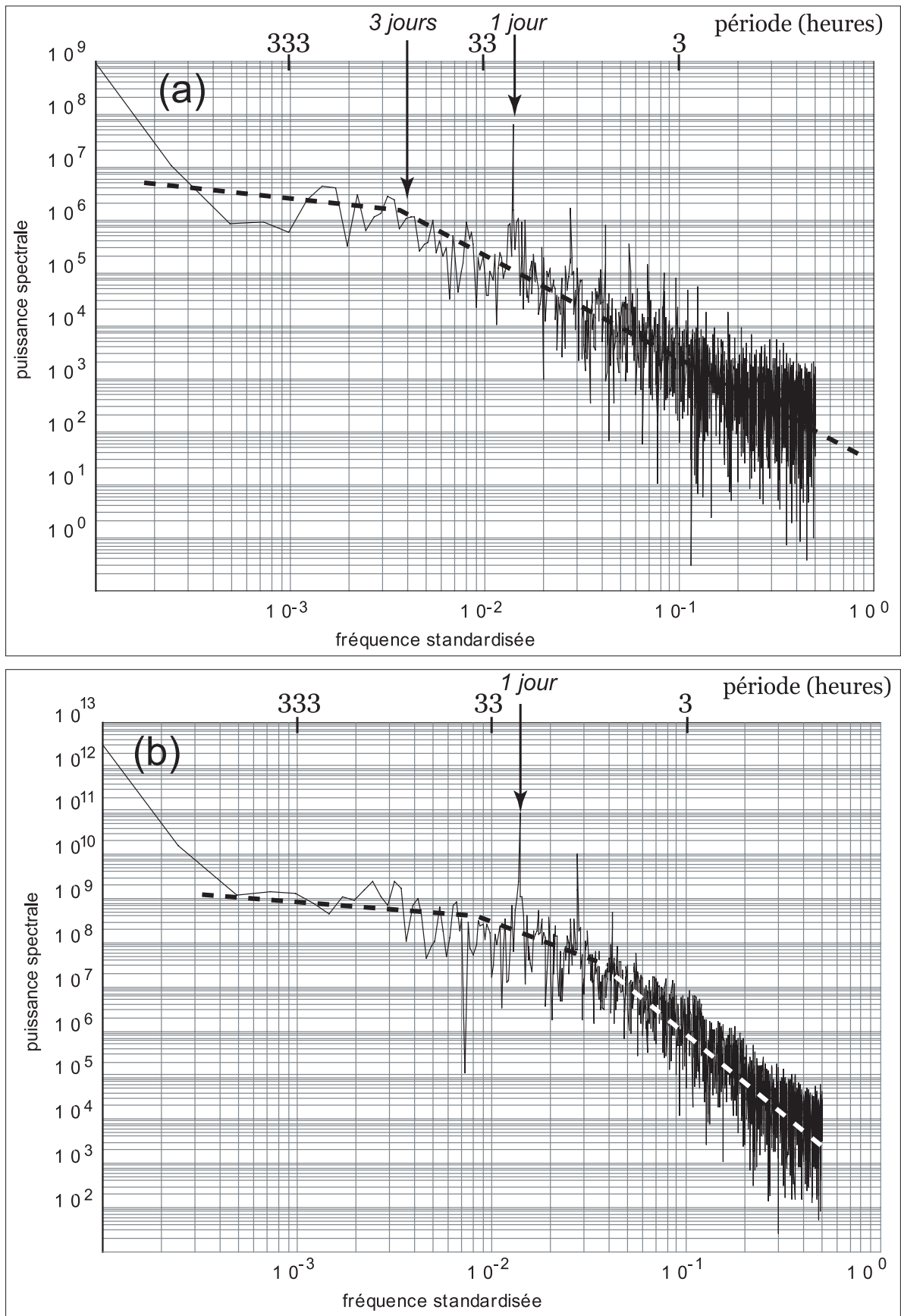
Fig. 2.30 : Spectrogramme obtenu par FFT pour la température de l'air et les débits du torrent émissaire du Gl. du Baounet. a: température de l'air; b: débits du torrent émissaire; calculs sur 4096 valeurs entre le 14/07/04 et le 08/09/04 avec un pas d'enregistrement de 20 minutes.
