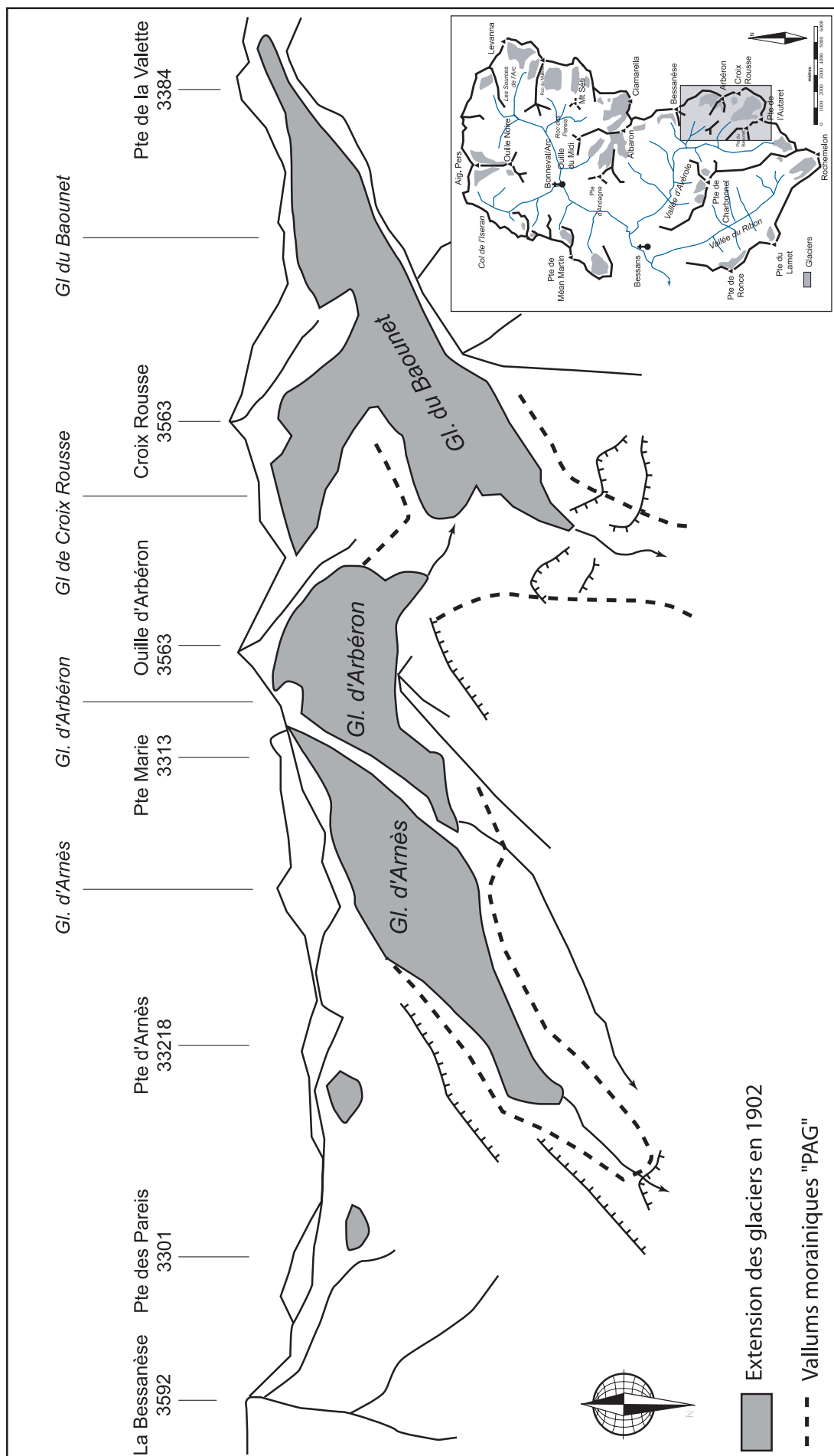
Fig. 3.1 - Le complexe glaciaire « Arnès-Arbéron-Baoumet » en 1909. Les trois principaux glaciers sont déjà bien individualisés et en retrait prononcé depuis le dernier maximum du Petit Age Glaciaire (1850). Les deux glacier-reliques sont encore visibles sous les Pointes d'Arnès et des Pareis. D'après P. Helbronner, 1932. Description géométrique détaillée des Alpes françaises
