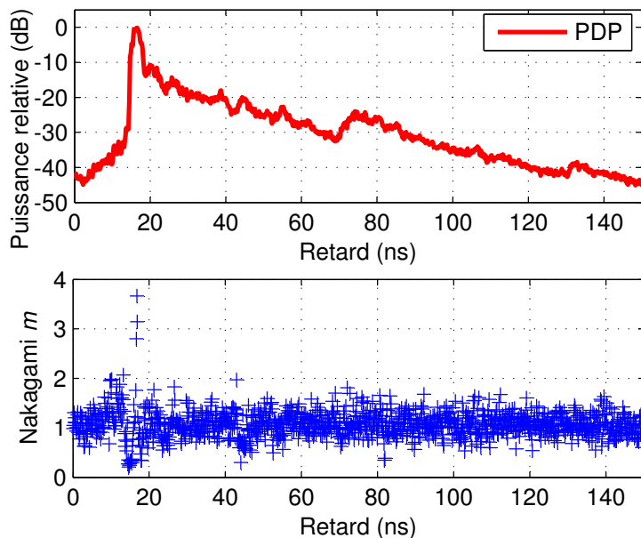
FIG. 3.21 – Exemple d'analyse du paramètre m . PDP mesuré en situation NLOS et valeur du paramètre m associé à chaque retard.
