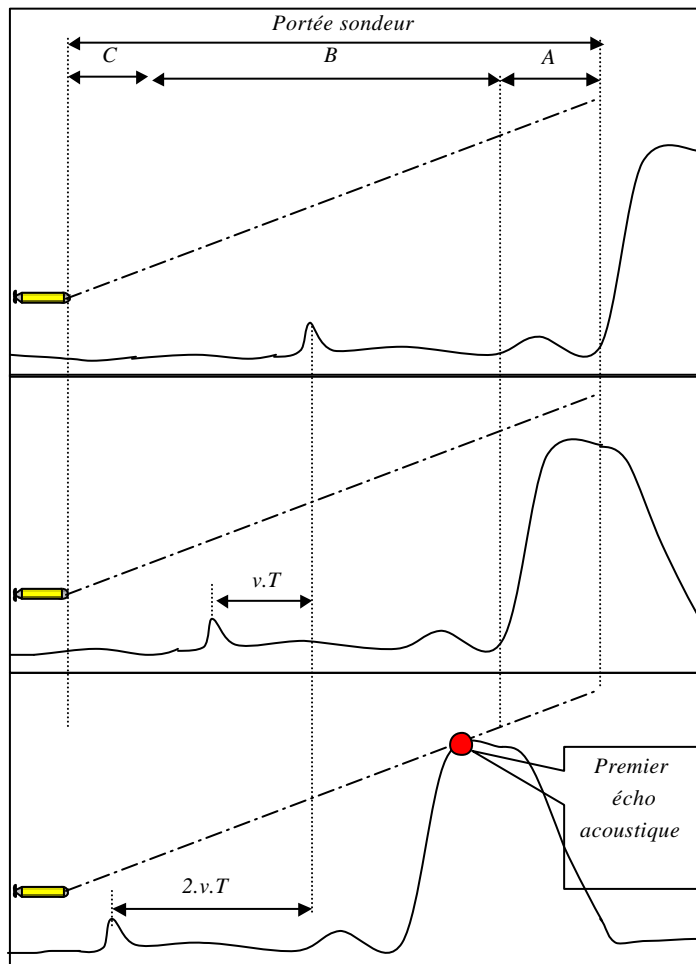
Figure 31 - Trois instants d'échantillonnage : t , t+T , t+2T . Détection de sommet dans la «zone sure» (B).
