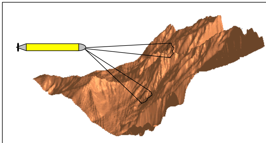
Figure 23 - Orientations des deux transducteurs reliés au sondeur
