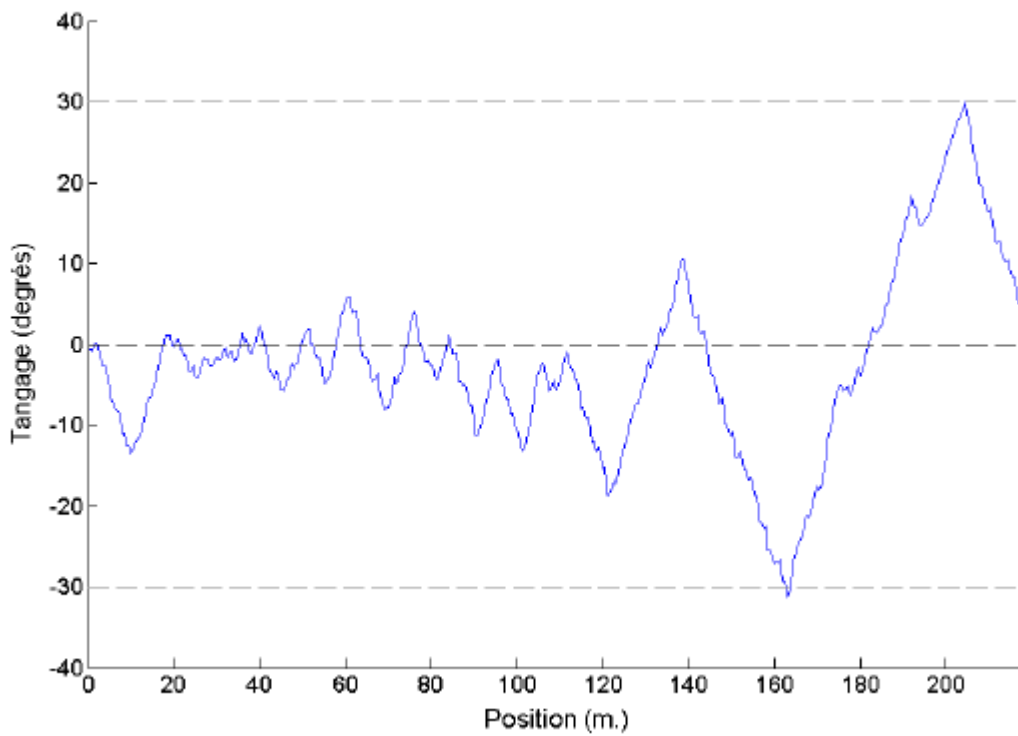
Figure 44 – Evolution de l’angle de tangage le long de la trajectoire précédente
