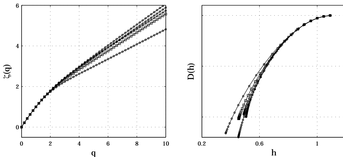
FIG. 9.6 – Cascades de Mandelbrot canoniques. Gauche : exposants estimés \widehat{\zeta_{cmc_i}^a}(q) sur l'ensemble de la réalisation ( \square ) ou sur chacune des 4 parties ( \circ ). Droite : transformées de Legendre correspondantes.
