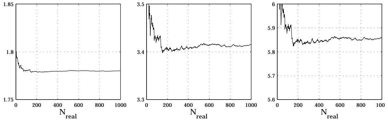
FIG. 9.3 – Cascades de Mandelbrot canoniques. Moyennes \widehat{\zeta}_{cmc_i}^a(q) en fonction du nombre de réalisations indépendantes utilisées, avec N_{réal} variant de 1 à 1000, pour q = 2 (gauche), q = 5 (milieu) et q = 10 (droite).
