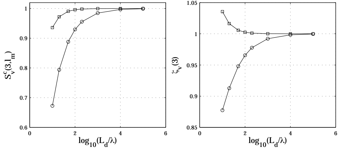
FIG. 13.11 – Valeurs maximales de S_v^c(3, l) et exposants \zeta_v(3) prédits par les modélisations correspondant à la turbulence en déclin homogène (13.10) (o) et à la turbulence forcée (13.19) (□).
