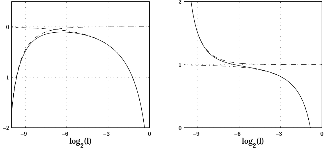
FIG. 13.8 – Modélisation de la fonction de structure d'ordre 3 ( L_d = 1 m et \lambda = 0.01 m ). Gauche : \log_2(S_v^c(3, l)) (trait continu), [1 - \zeta_v(2) \left(\frac{\lambda}{L_d}\right)^2 \left(\frac{l}{L_d}\right)^{\zeta_v(2)-2}] (---) et [1 - \frac{5}{5+\zeta_v(2)} \left(\frac{l}{L_d}\right)^{\zeta_v(2)}] (.-). Droite : exposants locaux correspondants.
