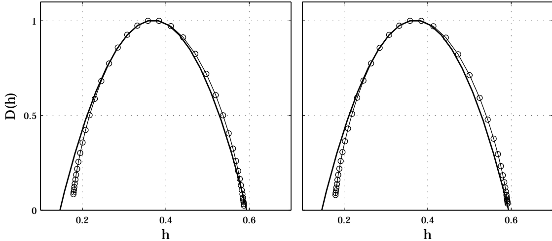
FIG. 7.4 – Cascades d'ondelette aléatoires. Trait continu : D_{rwc}(h) . \circ : TL[\widehat{\zeta_{rwc_i}^l}](h) (gauche) et TL[\widehat{\zeta_{rwc_i}^m}](h) (droite).
