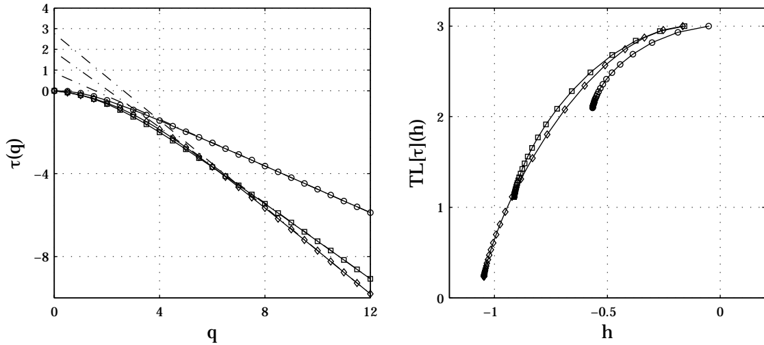
FIG. 12.9 – Données de dissipation DNS, R_\lambda \simeq 140 . Gauche : \widehat{\tau}_{DNS_i}^{d',3D}(q) (o), \widehat{\tau}_{DNS_i}^{d',2D}(q) (□), \widehat{\tau}_{DNS_i}^{d',1D}(q) (◇) et comportements linéaires asymptotiques associés (trait en pointillés). Droite : TL[\widehat{\tau}_{DNS_i}^{d',3D}](h) (o), TL[\widehat{\tau}_{DNS_i}^{d',2D}](h) (□), TL[\widehat{\tau}_{DNS_i}^{d',1D}](h) (◇). Toutes les transformées de Legendre sont définies selon TL[f](h) = 3 + \min_q(qh - f(q)) .
