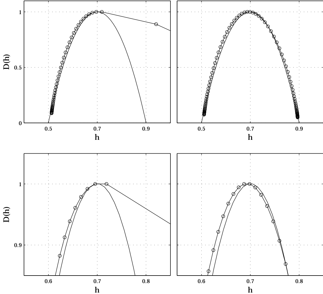
FIG. 7.1 – Cascades d'ondelette aléatoires. Trait continu : D_{rwc}(h) . \circ : TL[\widehat{\zeta_{rwc_i}^d}](h) (gauche) et TL[\widehat{\zeta_{rwc_i}^l}](h) (droite). Haut : totalité du spectre de singularités et bas : zoom sur la partie supérieure.
