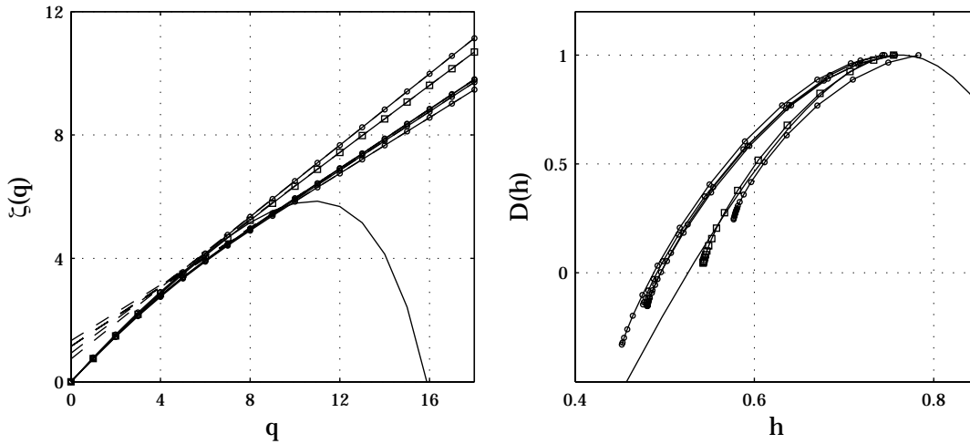
FIG. 10.5 – Mouvement brownien fractionnaire en temps multifractal. Gauche : exponents \widehat{\zeta_{fbmmt_i}^d}(q) pour 5 réalisations (o) et \widehat{\zeta_{fbmmt_i}^d}(q) (□), moyenne des \widehat{\zeta_{fbmmt_i}^d}(q) sur N_{réal} = 1000 réalisations, trait continu : fonction \varphi_{fbmmt}(q) et trait en pointillé : comportement linéaire asymptotique. Droite : TL[\widehat{\zeta_{fbmmt_i}^d}](h) (o) et leur moyenne (□), transformée de Legendre de \varphi_{fbmmt}(q) (trait continu).
