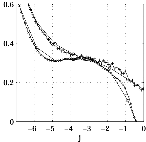
FIG. 8.6 – Données de l'ÉNSL , R_\lambda \simeq 380 . Exposants locaux correspondant aux fonctions de structure construites à l'aide des coefficients d'ondelette discrets ( \square ), des coefficients dominants ( \circ ), des coefficients d'ondelette continus ( \times ) et des coefficients mmto ( + ).
