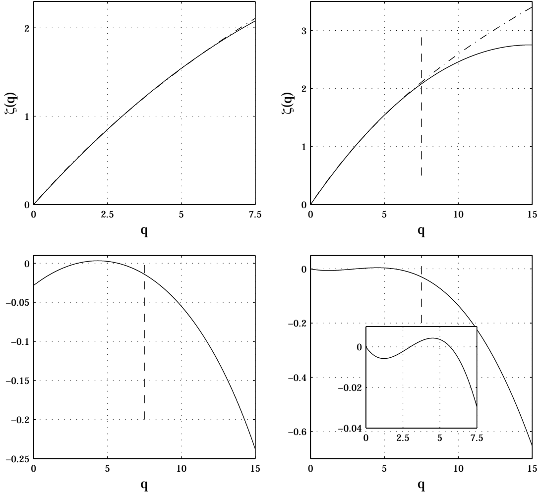
FIG. 12.6 – Comparaisons entre les modèles log-normal ( C_2 = 0.025 ) et de She-Lévêque. En haut : \varphi_{v,ln}(q) (trait continu) et \varphi_{v,SL}(q) (trait en pointillés). En bas : écarts relatif : (\varphi_{v,ln}(q) - \varphi_{v,SL}(q))/\varphi_{v,ln}(q) (à gauche) et absolu : \varphi_{v,ln}(q) - \varphi_{v,SL}(q) (à droite). La barre verticale en pointillés représente la valeur estimée de l'ordre critique : q_*^+ \simeq 7.5 .
