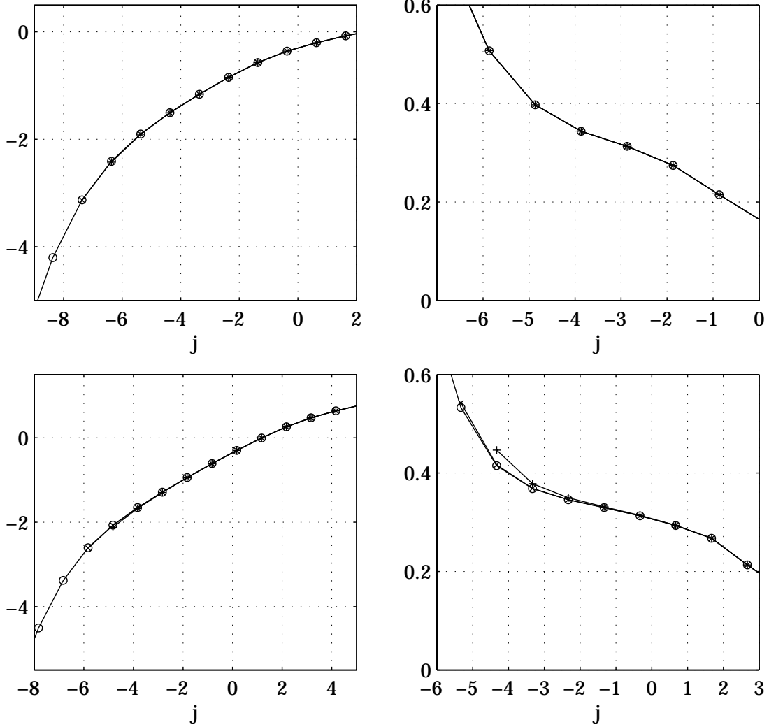
FIG. 8.3 – Fonctions de structure ”classiques” et ”réduites” (gauche) et exposants locaux correspondants (droite). \log_2 S_v^l(q, j) (o) et \log_2 S_v^{l'}(q, j) , pour les données de l’ENSL (haut) : j_{min} = j_0 + 5 ( \times ) et j_{min} = j_0 + 6 (+), et pour les données de Modane (bas) : j_{min} = j_0 + 4 ( \times ) et j_{min} = j_0 + 5 (+).
