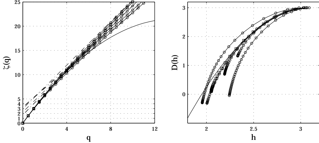
FIG. 11.1 – Cascades de Mandelbrot canoniques. Gauche : exposants \widehat{\zeta_{cmc_i}^d}(q) pour 5 réalisations (o) et \widehat{\zeta_{cmc_i}^d}(q) ( \square ), moyenne des \widehat{\zeta_{cmc_i}^d}(q) sur N_{réal} = 100 réalisations, trait continu : fonction \varphi_{cmc}(q) et trait en pointillé : comportement linéaire asymptotique. Droite : TL[\widehat{\zeta_{cmc_i}^d}](h) (o) et leur moyenne ( \square ), transformée de Legendre de \varphi_{cmc}(q) (trait continu).
