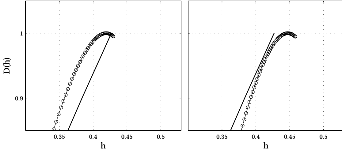
FIG. 7.5 – Séries d’ondelette aléatoires. Trait continu : D_{rws}(h) . \circ : TL[\widehat{\zeta_{rws_i}^l}](h) (gauche) et TL[\widehat{\zeta_{rws_i}^m}](h) (droite).
