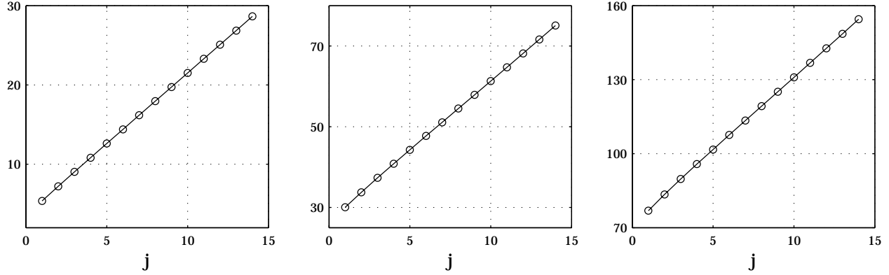
FIG. 9.2 – Cascades de Mandelbrot canoniques. Moyennes de \log_2 S_{cmc_i}^a(q, j) sur les N_{réal} = 1000 réalisations indépendantes, en fonction de l’octave j , pour q = 2 (gauche), q = 5 (milieu) et q = 10 (droite).
