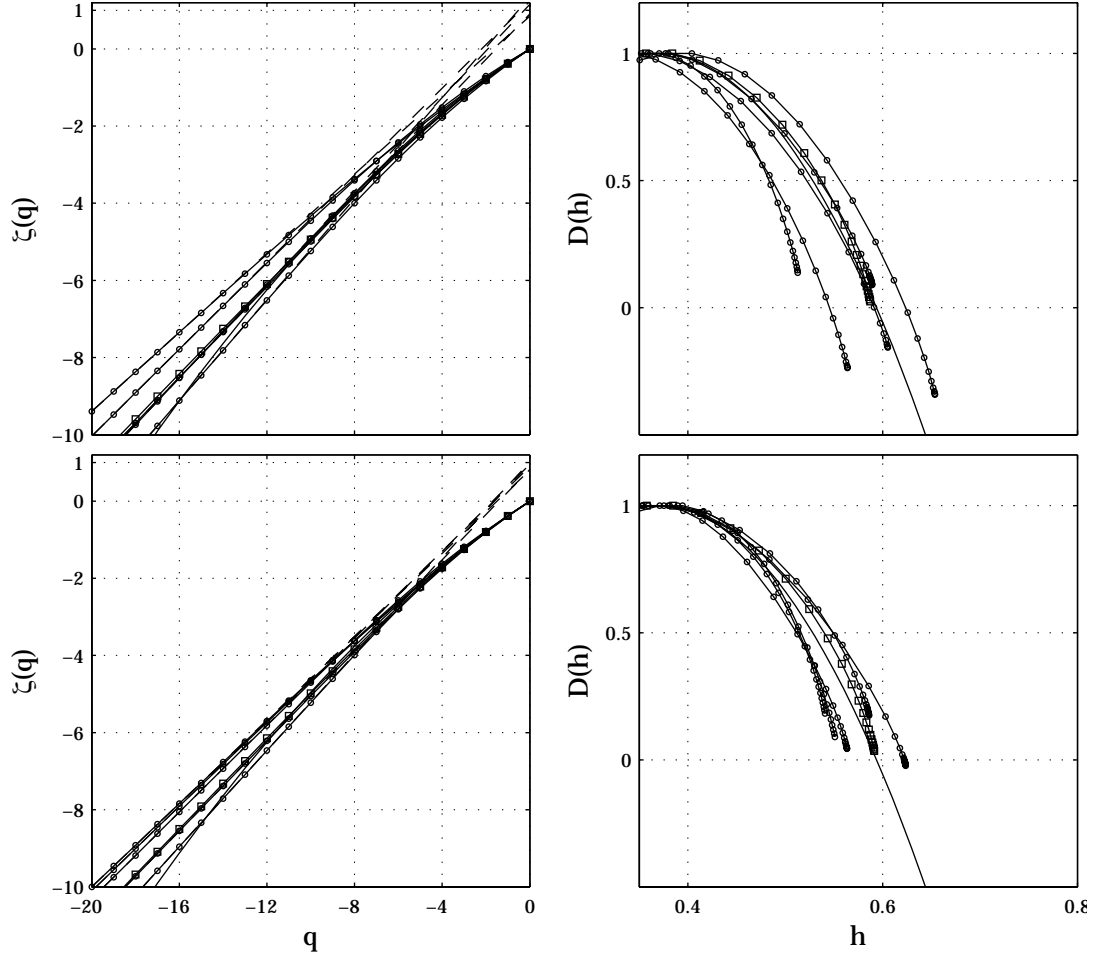
FIG. 10.13 – Cascade d’ondelette aléatoire. Gauche : exposants \widehat{\zeta}_{rwc_i}^p(q) pour 5 réalisations (o) et \widehat{\zeta}_{rwc_i}^p(q) ( \square ), moyenne des \widehat{\zeta}_{rwc_i}^p(q) sur N_{réal} = 400 réalisations, trait continu : fonction \varphi_{rwc}(q) et trait en pointillé : comportement linéaire asymptotique. Droite : TL[\widehat{\zeta}_{rwc_i}^p](h) (o) et leur moyenne ( \square ), transformée de Legendre de \varphi_{rwc}(q) (trait continu). Formalismes multifractals basés sur les coefficients dominants (haut) et coefficients mmt (bas)
