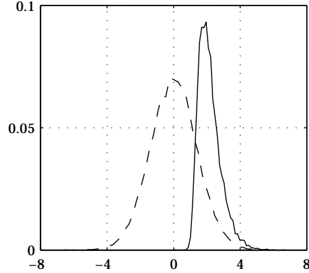
FIG. 6.2 – Histogrammes des coefficients d'ondelette discrets d_f(j = 5, k) (trait en pointillés) et des coefficients dominants l_f(j = 5, k) (trait continu) calculés sur une réalisation du processus marche aléatoire multifractal (se reporter à l'annexe D).
