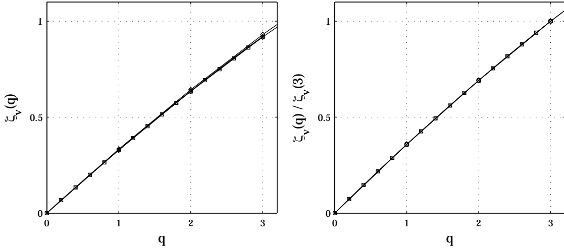
FIG. 13.3 – Exposants \widehat{\zeta}_v^p(q) (droite) et \widehat{\zeta}_v^p(q) = \widehat{\zeta}_v^p(q)/\widehat{\zeta}_v^p(3) (gauche) pour les données de Modane ( R_\lambda \simeq 2000 ), construits à partir des coefficients d’ondelette discrets ( \square ), des coefficients dominants ( \times ), des coefficients d’ondelette continus ( \diamond ) et des coefficients mmt0 ( \circ ).
