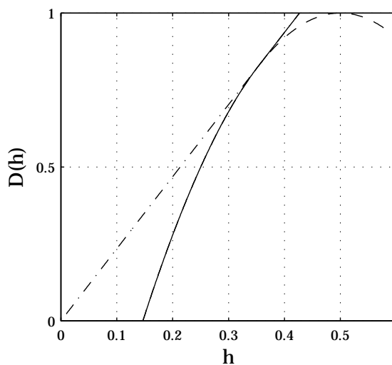
FIG. 4.2 – Spectre de singularités D_{rws}(h) (trait continu) et fonction \rho(h) (trait tiret-tiret) d'une série d'ondelette aléatoire construite à l'aide d'un générateur gaussien de paramètres m = 0.5 et \sigma = 0.3 .
