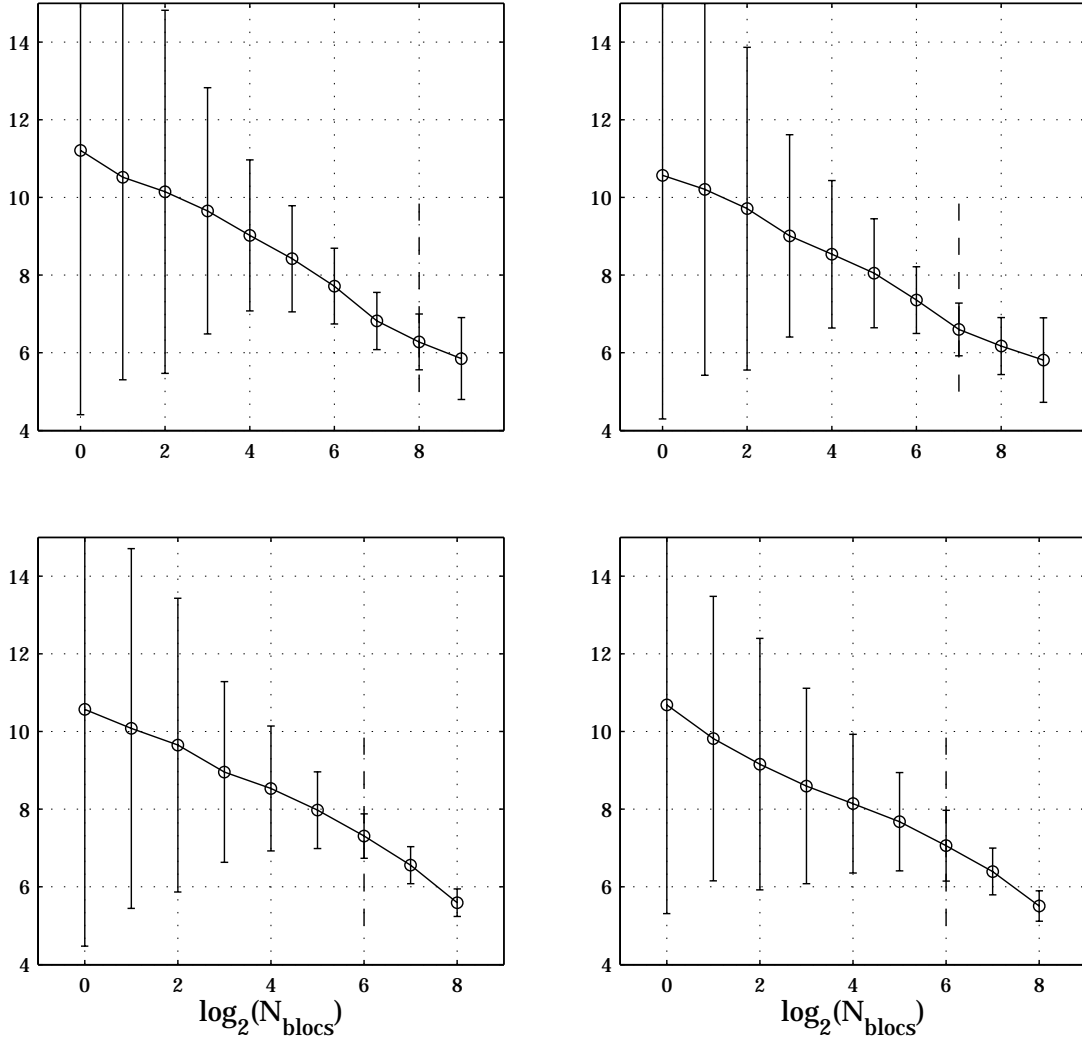
FIG. 12.5 – Estimateur \widehat{q}_*^+(N_{\text{blocs}}) : données de l'ÉNSL, R_\lambda \simeq 380 (en haut à gauche) et R_\lambda \simeq 580 (en haut à droite), données de Modane (en bas à gauche) et données GREC (en bas à droite). Les intervalles de confiance correspondent à \pm 2 écarts-type estimés. La droite verticale signale la valeur de N_{\text{blocs}} pour laquelle chaque sous-bloc a pour longueur une échelle intégrale.
