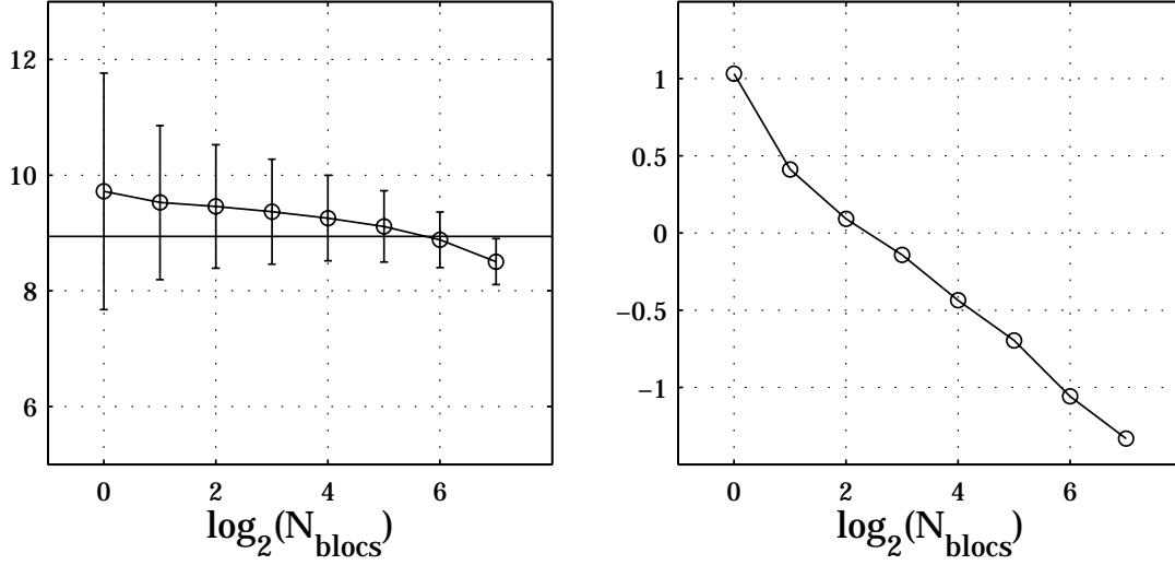
FIG. 10.9 – Cascade d’ondelette aléatoire. Gauche : moyenne des \widehat{q}_*^+(N_{\text{blocs}}) sur les N_{\text{réal}} = 400 réalisations en fonction de \log_2 N_{\text{blocs}} . Les intervalles de confiance correspondent à \pm 2 écarts-type estimés. La droite horizontale rappelle q_*^+ \simeq 8.94 . Droite : écart-type de \widehat{q}_*^+(N_{\text{blocs}}) en fonction de N_{\text{blocs}} , dans un diagramme log-log.
