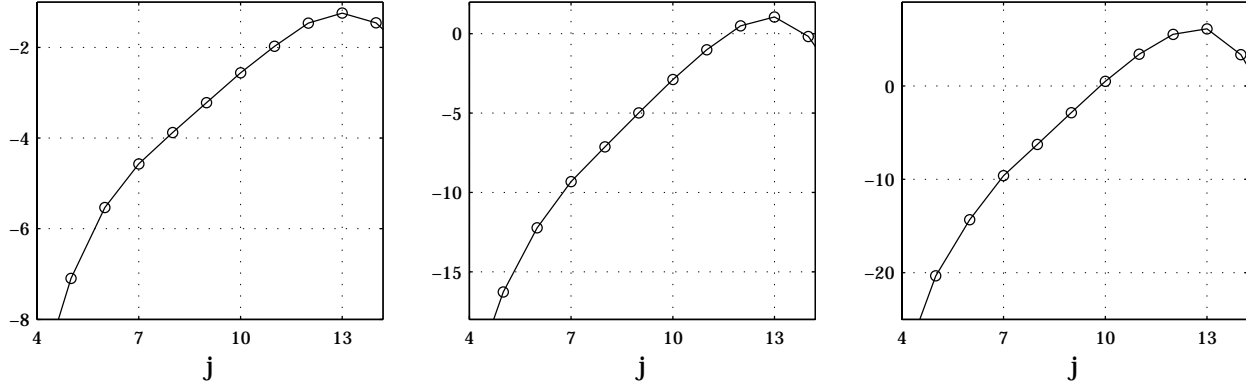
FIG. 12.2 – Données de l'ÉNSL , R_\lambda \simeq 580 . Moyennes de \log_2 S_v^d(q, j) sur les 80 runs, en fonction de l'octave j , pour q = 2 (gauche), q = 8 (milieu) et q = 15 (droite).
