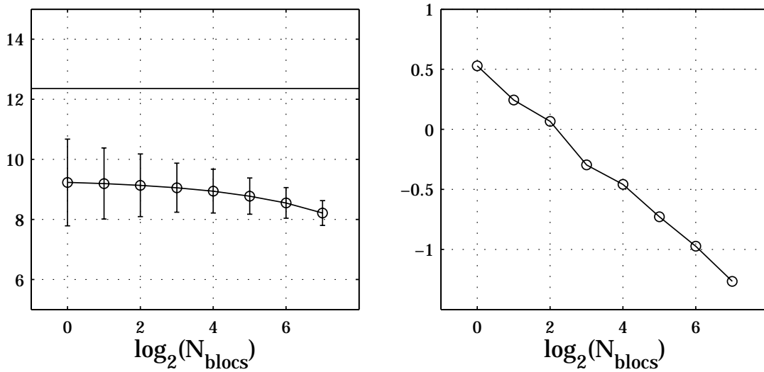
FIG. 10.11 – Cascade d'ondelette aléatoire correspondant au modèle de She-Lévêque. Gauche : moyenne des \widehat{q}_*^+(N_{blocs}) sur les N_{réal} = 400 réalisations en fonction de \log_2 N_{blocs} . Les intervalles de confiance correspondent à \pm 2 écarts-type estimés. La droite horizontale rappelle q_*^+ \simeq 12.36 . Droite : écart-type de \widehat{q}_*^+(N_{blocs}) en fonction de N_{blocs} , dans un diagramme log-log.
