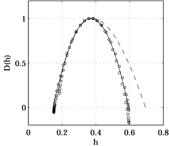
FIG. 8.7 – Données de Modane , R_\lambda \simeq 2000 . \overline{TL[\widehat{\zeta}_v^l]}(h) (o) et \overline{TL[\widehat{\zeta}_v^m]}(h) . Modèle log-normal (avec C_2 = 0.025 ) (trait continu) et modèle de She-Lévy (trait discontinu).
