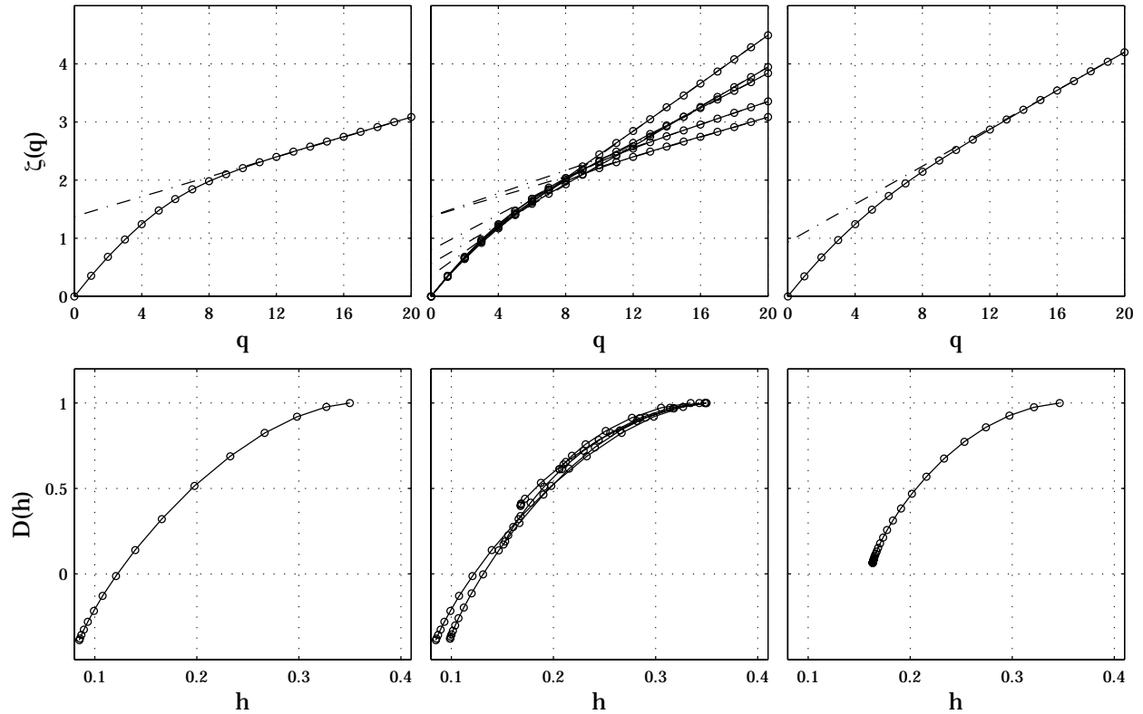
FIG. 12.1 – Données de l'ÉNSL , R_\lambda \simeq 580 . Haut : exposants \widehat{\zeta}_{X_i}^d(q) pour 1 run (gauche), 5 runs (milieu) et moyenne \overline{\zeta}_{X_i}^d(q) sur les 80 runs. Trait en pointillé : comportements linéaires asymptotiques. Bas : transformées de Legendre des exposants \widehat{\zeta}_{X_i}^d(q) pour 1 run (gauche), 5 runs (milieu) et moyenne des transformées de Legendre des \widehat{\zeta}_{X_i}^d(q) sur les 80 runs.
