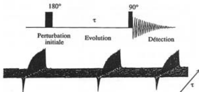
Figure A-III-8 : Séquence d'acquisition « inversion-récupération » (figure tirée de la référence [79]).
