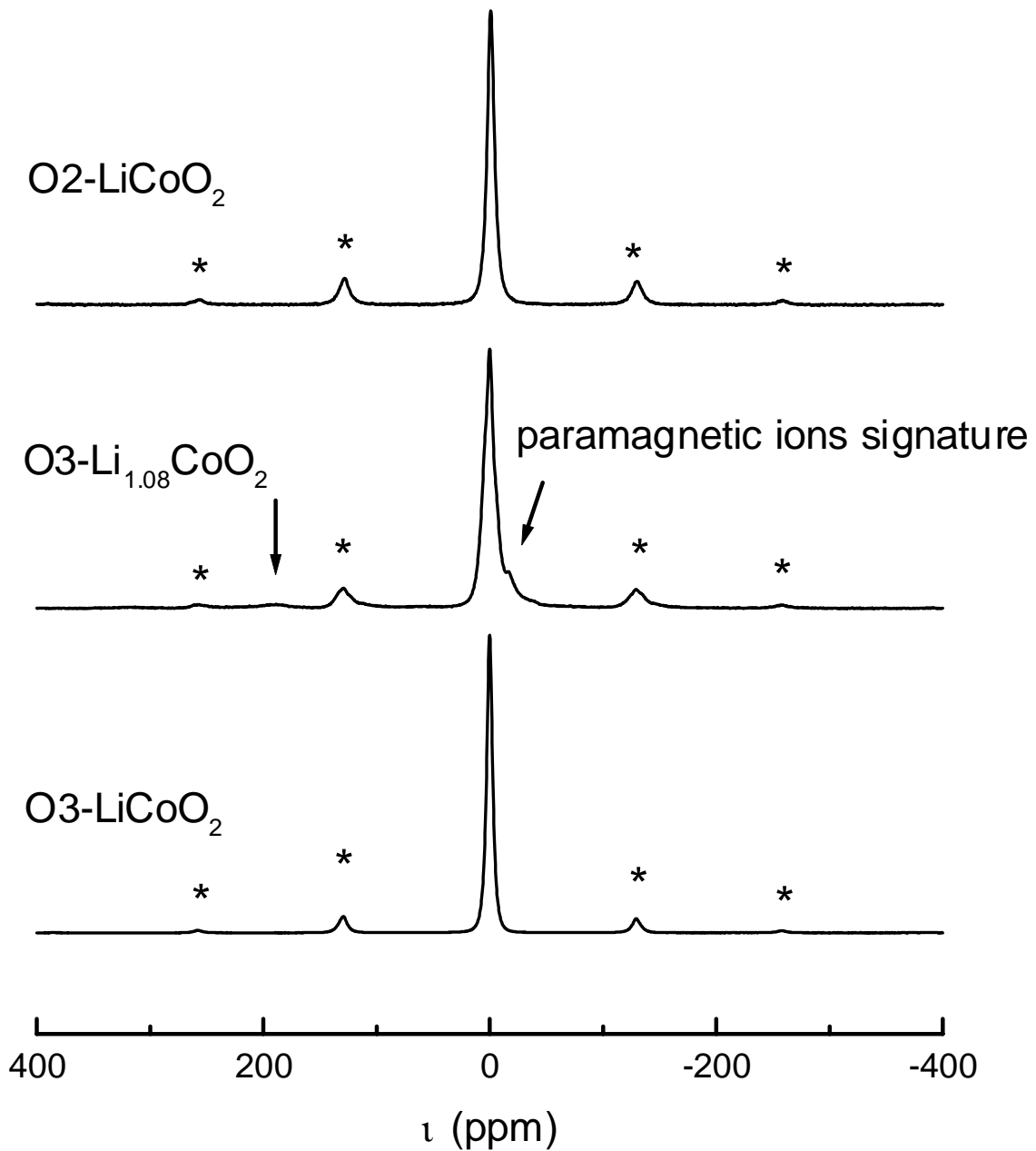
Figure B-I-8 : Spectres de RMN de ^7\text{Li} des phases O2- \text{LiCoO}_2 , O3- \text{LiCoO}_2 , et O3- \text{Li}_{1.08}\text{CoO}_2 enregistrés en rotation à l'angle magique ( \tau_r = 10 kHz) à l'aide d'une séquence d'écho de Hahn.
