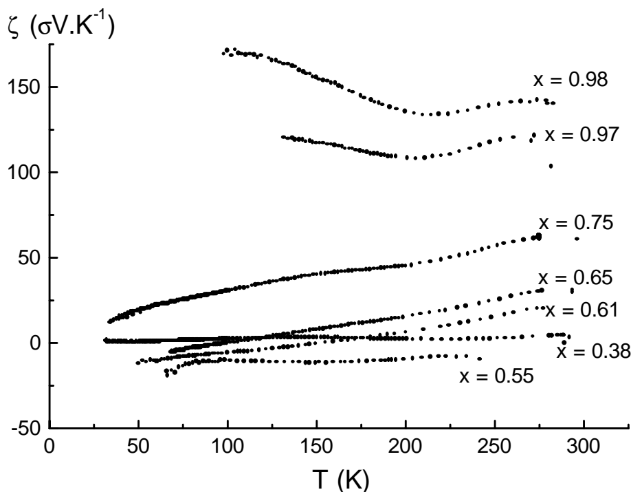
Figure B-III-20 : Variation thermique du coefficient Seebeck des phases \text{Li}_x\text{CoO}_2 ( 0.38 \leq x \leq 0.98 ).
