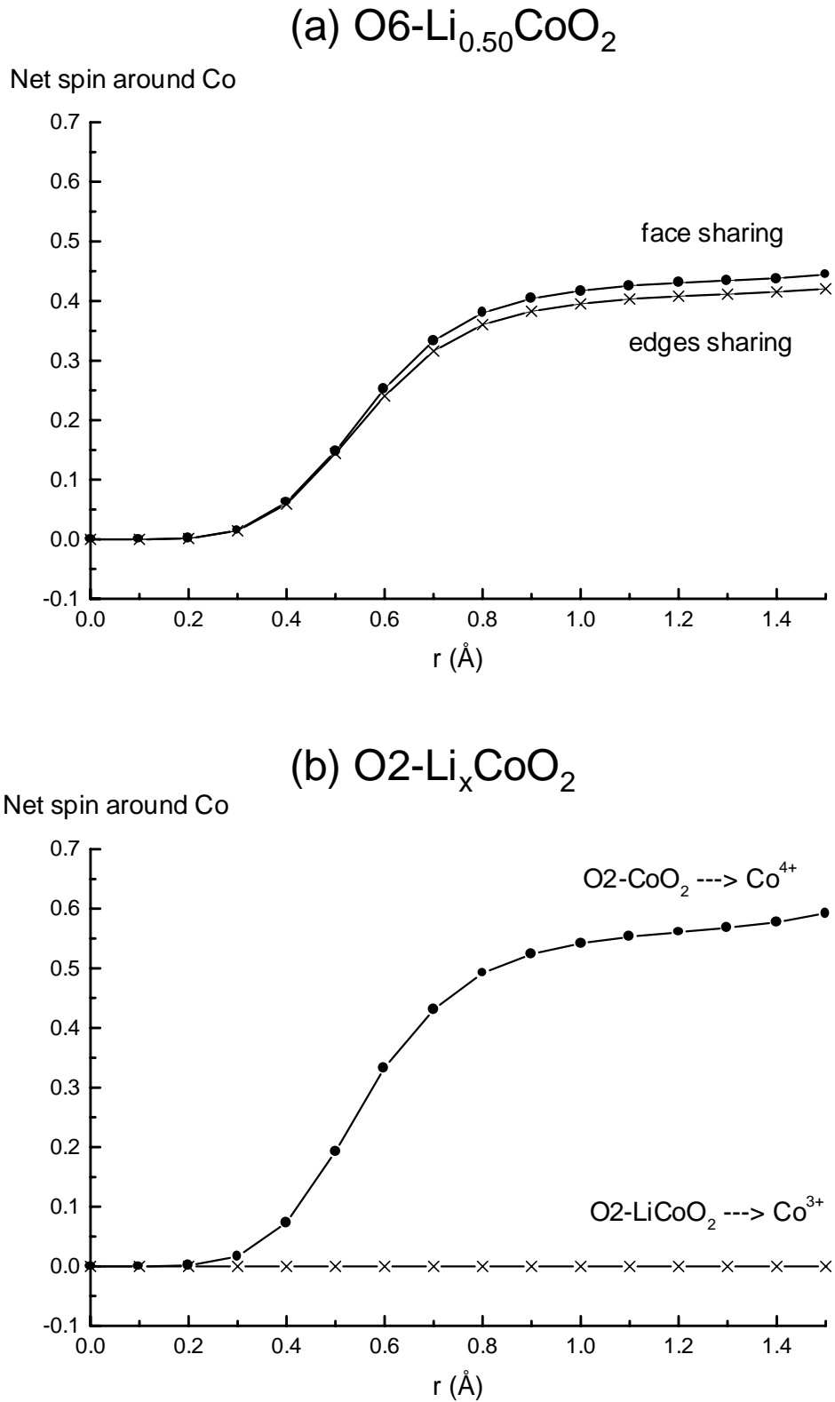
Figure B-IV-10 : Intégration de la densité de spin autour du cobalt dans (a) \text{O6-Li}_{0.50}\text{CoO}_2 et dans (b) \text{O2-CoO}_2 et \text{O2-LiCoO}_2 .
