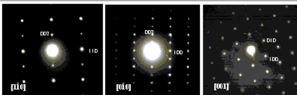
Fig. III-37 Clichés de diffraction électronique de l'hydrure \text{CeNiSnH}_{1,8(1)} selon les axes de zone [1\bar{1}0] , [0\bar{1}0] et [001] .
