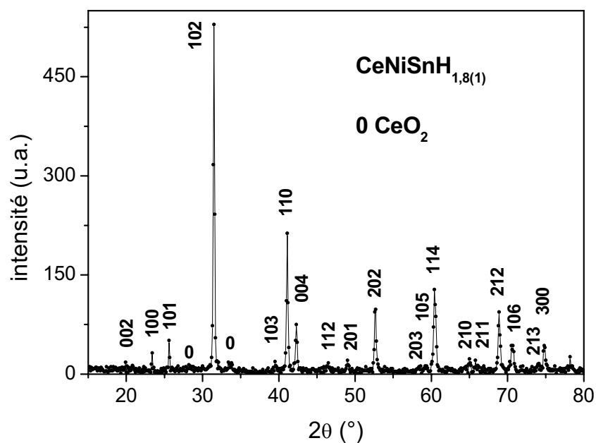
Fig. III-36 Diffractogramme de rayons X de l'hydrure \text{CeNiSnH}_{1,8(1)} .
