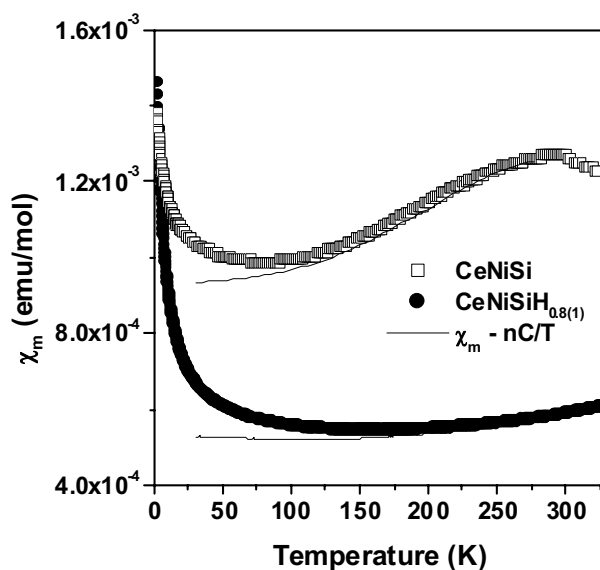
Fig. III-56 Dépendance thermique de la susceptibilité magnétique de CeNiSi et de CeNiSiH 0,8(1) .
