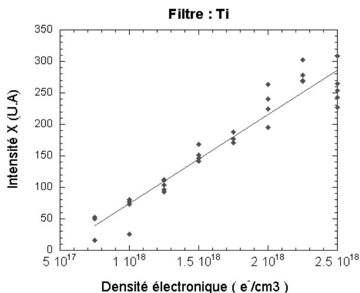
FIG. 5.19 – Evolution de l'intensité du rayonnement X en fonction de la densité électronique du plasma pour la bande spectrale passant du titane ( \sim 350\text{eV} ).
