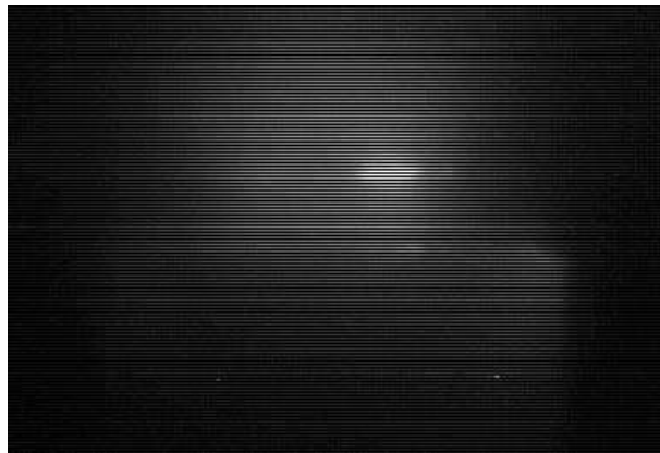
FIG. 5.2 – Image de l'émission propre lorsque le laser est focalisé sur le bord avant de jet de gaz.
