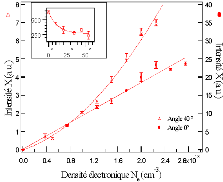
FIG. 5.20 – Evolution de l'intensité du rayonnement X en fonction de la densité électronique du plasma pour deux angles d'observation : selon l'axe de propagation du laser 0^\circ et hors axe à 40^\circ .
