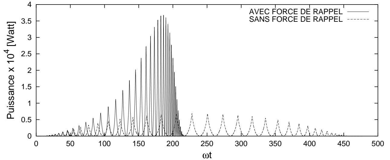
FIG. 2.21 – La courbe en trait plein représente la puissance instantanée lorsque la force de rappel des ions est prise en compte. Les conditions sont a_0 = 5 , \tau = 30 fs, n_e = 1 \times 10^{19} cm ^{-3} . Le laser est polarisé linéairement. La courbe en trait discontinu représente la puissance émise lorsque l'effet de la force de rappel des ions n'est pas pris en compte.
