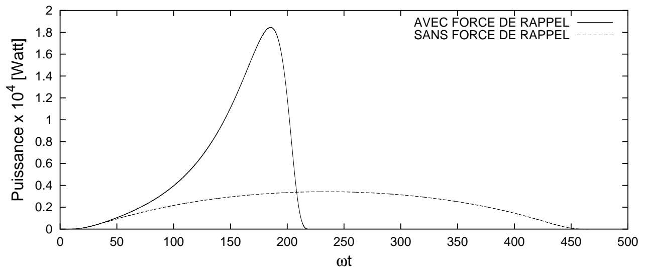
FIG. 2.22 – La courbe en trait plein représente la puissance instantanée lorsque la force de rappel des ions est prise en compte. Les conditions sont a_0 = 5 , \tau = 30 fs, n_e = 1 \times 10^{19} cm ^{-3} . Le laser est polarisé circulairement. La courbe en trait discontinu représente la puissance émise lorsque l'effet de la force de rappel des ions n'est pas pris en compte.
