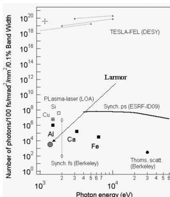
FIG. 6.1 – Sources de rayonnement X ultra-brèves.
