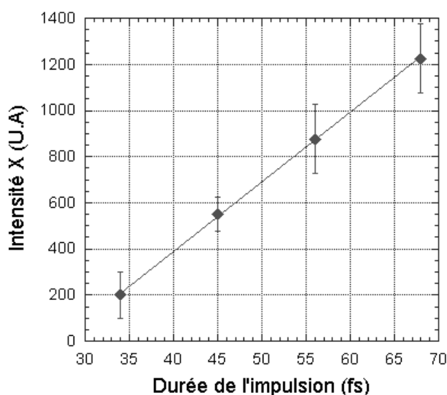
FIG. 5.26 – Evolution de l'intensité du rayonnement X en fonction la durée de l'impulsion laser à intensité laser constante.
