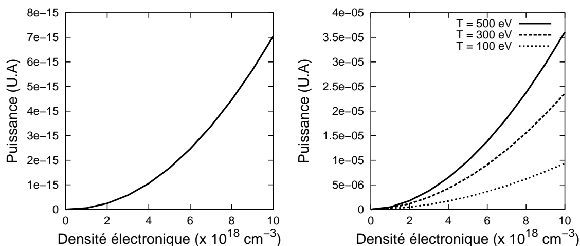
FIG. 5.28 – Puissance des rayonnements de recombinaisons radiatives (à gauche) et Bremsstrahlung (à droite) en fonction de la densité électronique du plasma. Le refroidissement par conduction thermique du plasma est pris en compte.
