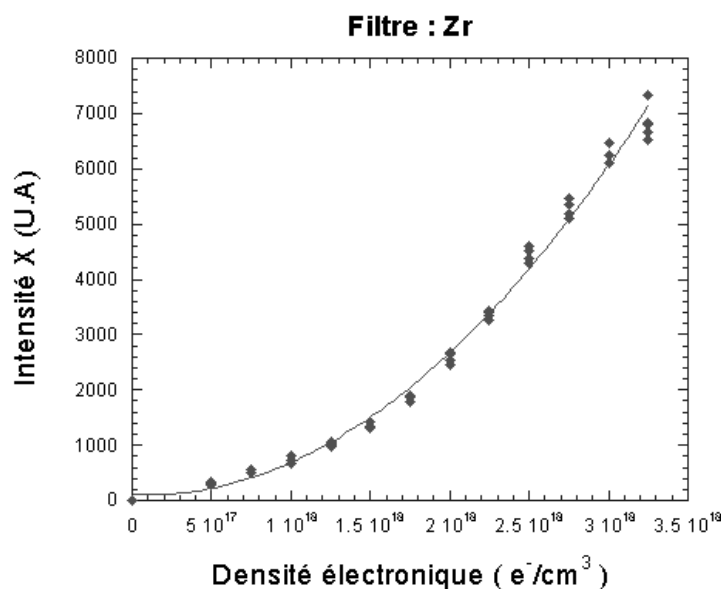
FIG. 5.29 – Evolution de l'intensité du rayonnement X en fonction de la densité électronique du plasma pour la bande spectrale passante du zirconium ( \sim 150\text{eV} ). Parabole f=1000\text{ mm} défocalisée.
