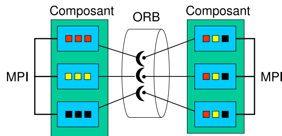
FIG. 3.1 – GRIDCCM : des composants CORBA parallèles utilisent CORBA et MPI.
