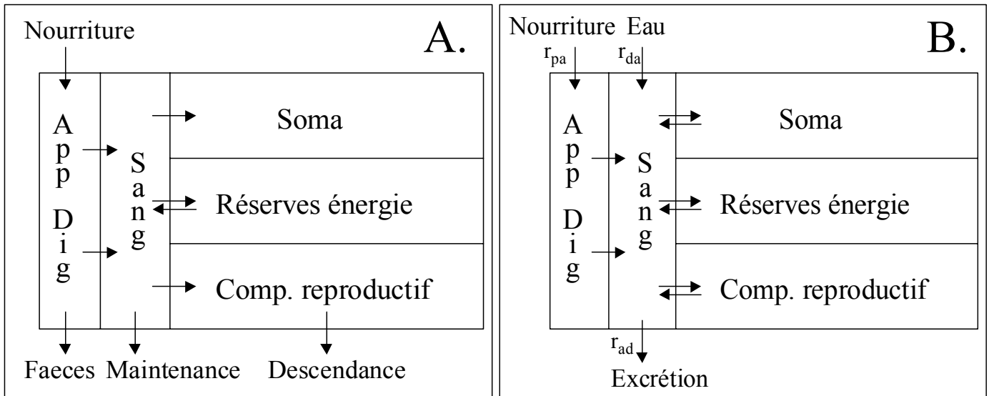
Figure 6.35: Représentation schématique des différents compartiments et flux de l'individu (A.) et du processus de bioaccumulation (B.) (d'après van Haren & Kooijman, 1994). r_{da} et r_{pa} : taux d'entrée du contaminant sous forme dissoute et particulaire, r_{ad} : taux d'élimination du contaminant.
