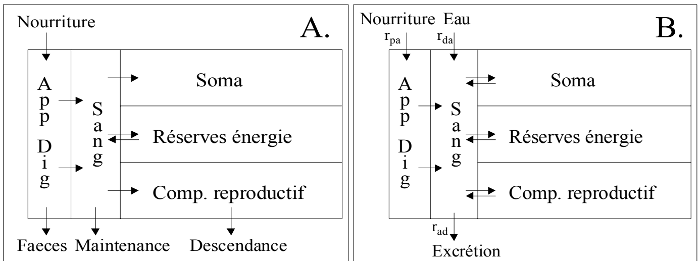
Figure 6.1: Représentation schématique des différents compartiments et flux de l'individu (A.) et du processus de bioaccumulation (B.) (d'après van Haren & Kooijman, 1994). r_{da} et r_{pa} : taux d'entrée du contaminant sous forme dissoute et particulaire, r_{ad} : taux d'élimination du contaminant.
