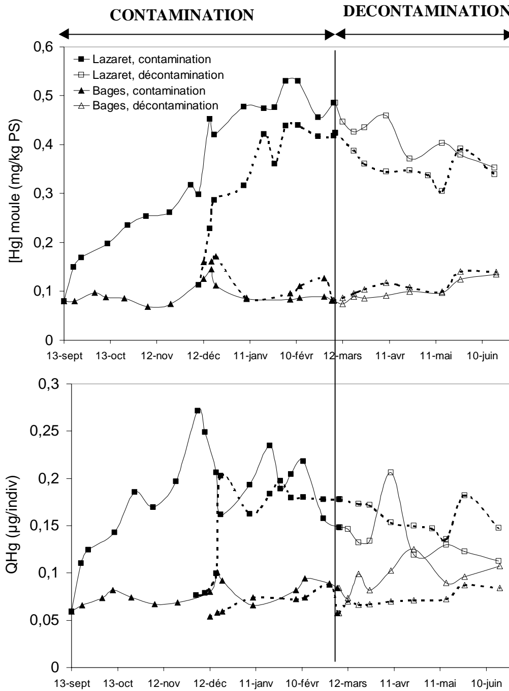
Figure 3.8: Cinétiques de bioaccumulation du mercure chez la moule, Mytilus galloprovincialis , sur les différents suivis réalisés. Concentrations exprimées en \text{mg}\cdot\text{kg}^{-1} (p.s.) et quantités en \mu\text{g}\cdot\text{individu}^{-1} :
