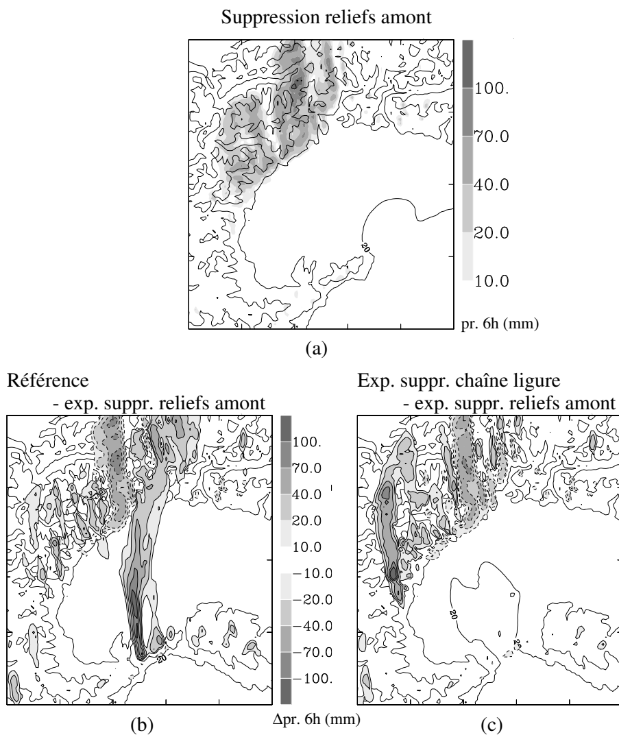
FIG. 6.3: Simulations en flux de sud uniforme (résolution : 2.5 km). (a) Simulation avec suppression des principaux reliefs amont : précipitations cumulées sur 6 h (échelle grisée, en mm). (b) Différence des précipitations sur 6 h entre l'expérience de référence et celle sans reliefs amont. (c) Différence des précipitations sur 6 h entre l'expérience sans chaîne ligure et celle sans reliefs amont.
