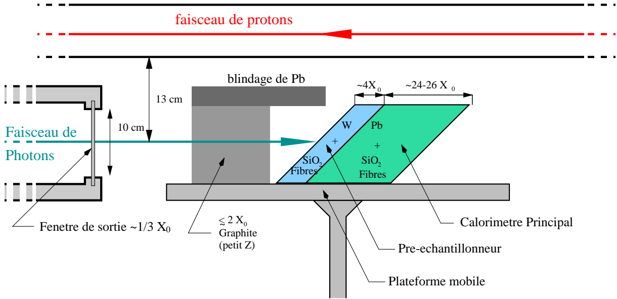
FIG. 4.20: Schéma du luminomètre dans le tunnel dans le plan y - z .
