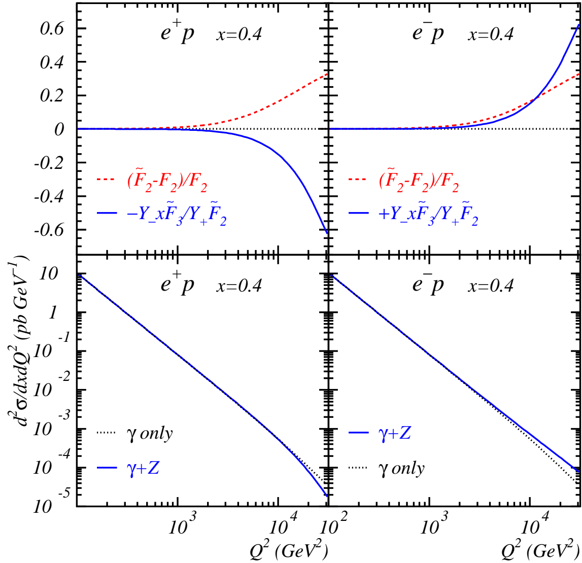
FIG. 2.3: En haut on voit l'effet de l'interférence \gamma Z et de l'échange de Z pour F_2 , et le poids relatif de Y_x \tilde{F}_3 par rapport à Y_+ \tilde{F}_2 . En bas la figure illustre la déviation de la section efficace par rapport à l'échange pur d'un photon.
