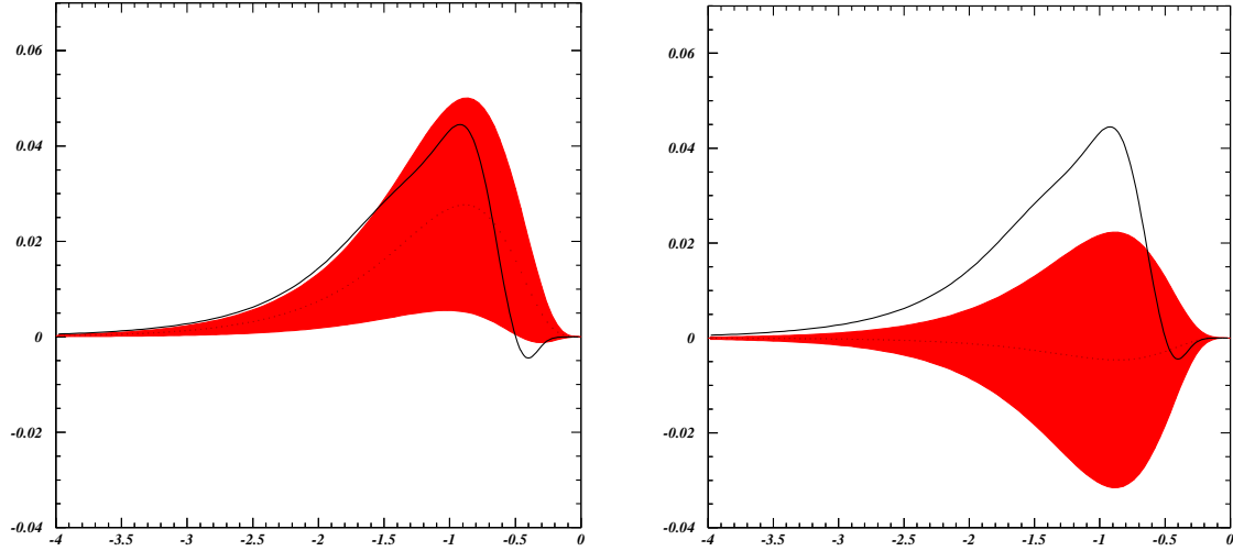
FIG. C.1: Asymétrie x(\bar{d} - \bar{u}) (enveloppe à 1 \sigma ) en fonction de \log_{10} x obtenue avec l'ajustement H1 seul pour les ajustements à 10 (à gauche) et 11 (à droite) paramètres libres. La ligne noire est le résultat de CTEQ6 pour x(\bar{d} - \bar{u}) .
