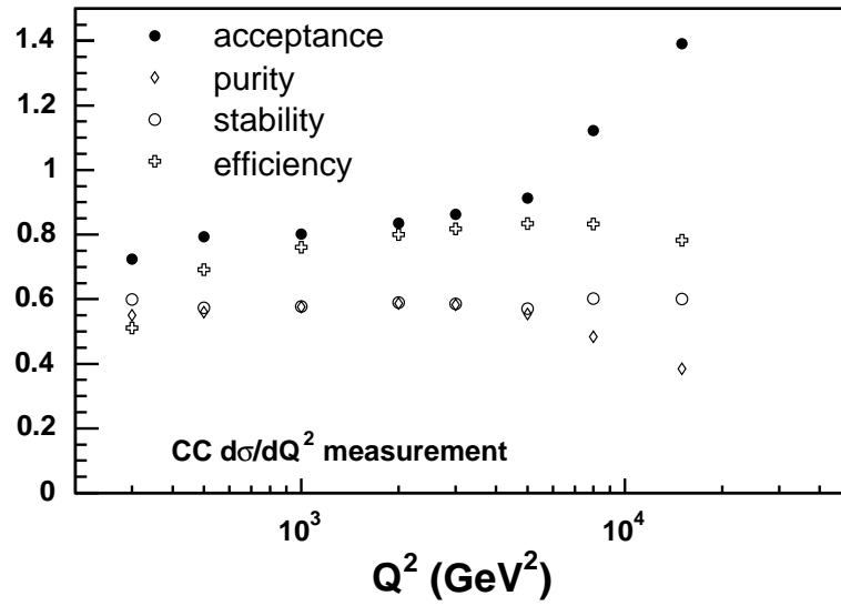
FIG. 7.13: Acceptance, pureté, stabilité et efficacité pour la mesure des sections efficaces CC d\sigma/dQ^2 .
