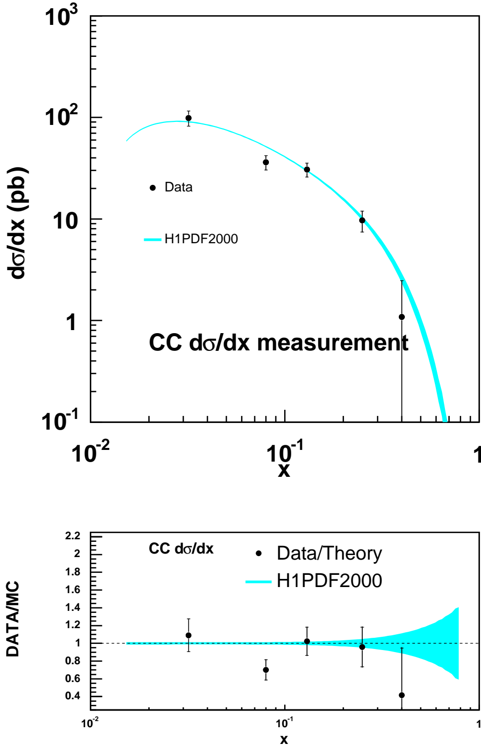
FIG. B.11: Sections efficaces d\sigma/dx ( y < 0,9 , Q^2 > 1000 GeV 2 ) pour la période L. Les bandes et barres d'erreurs sont définies comme sur la figure B.8.
