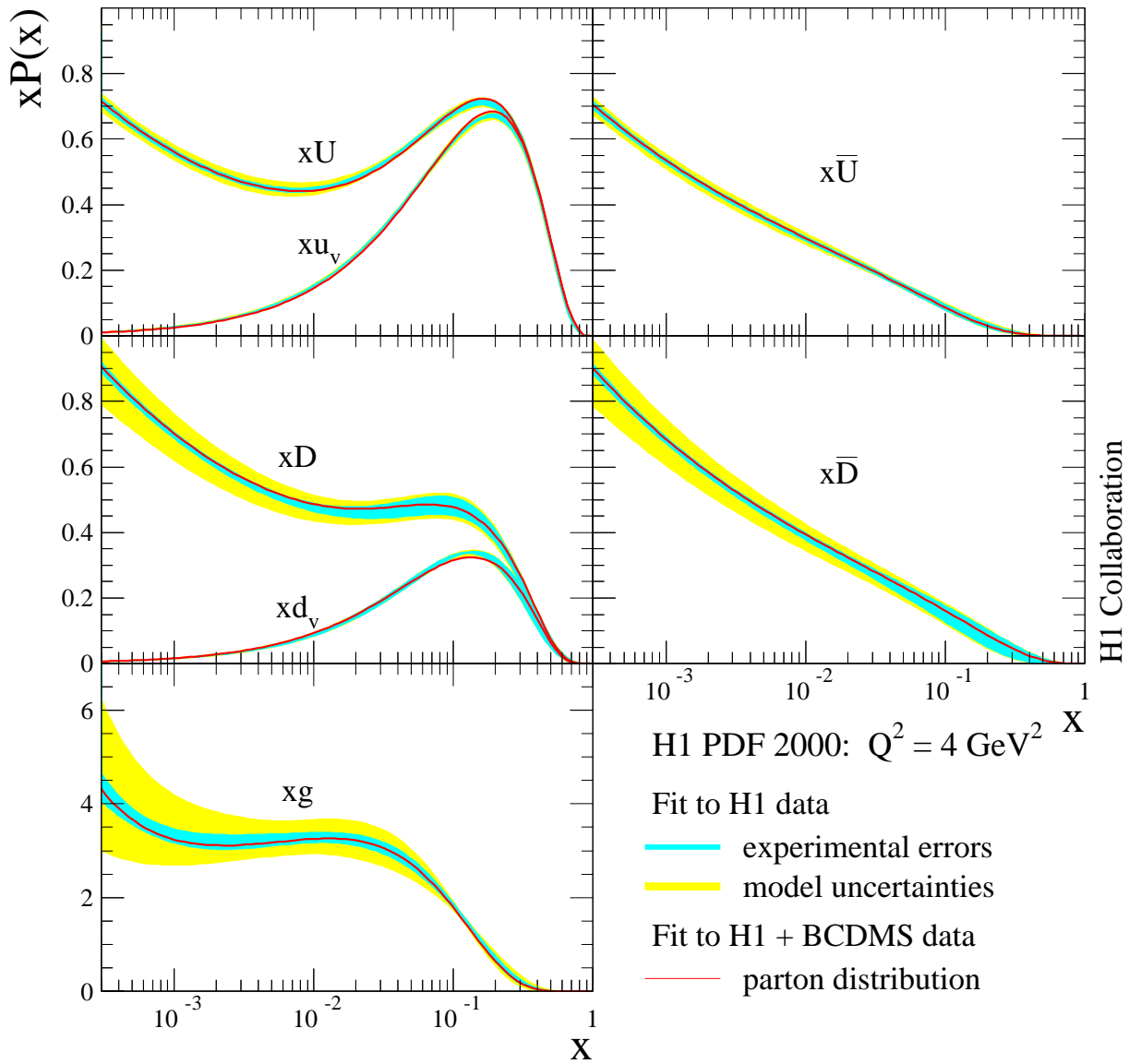
FIG. 8.2: Distributions de partons xg , xU , xD , x\bar{U} , x\bar{D} ainsi que xu_v = x(U - \bar{U}) , xd_v = x(D - \bar{D}) à l'échelle Q_0^2 = 4 \text{ GeV}^2 pour les données H1 seules. La bande d'erreur interne comprend les incertitudes expérimentales et la bande externe comprend l'ajout en quadrature des incertitudes expérimentales et de modélisation. La valeur centrale de l'ajustement aux données de H1+BCDMS est montrée à titre de comparaison.
