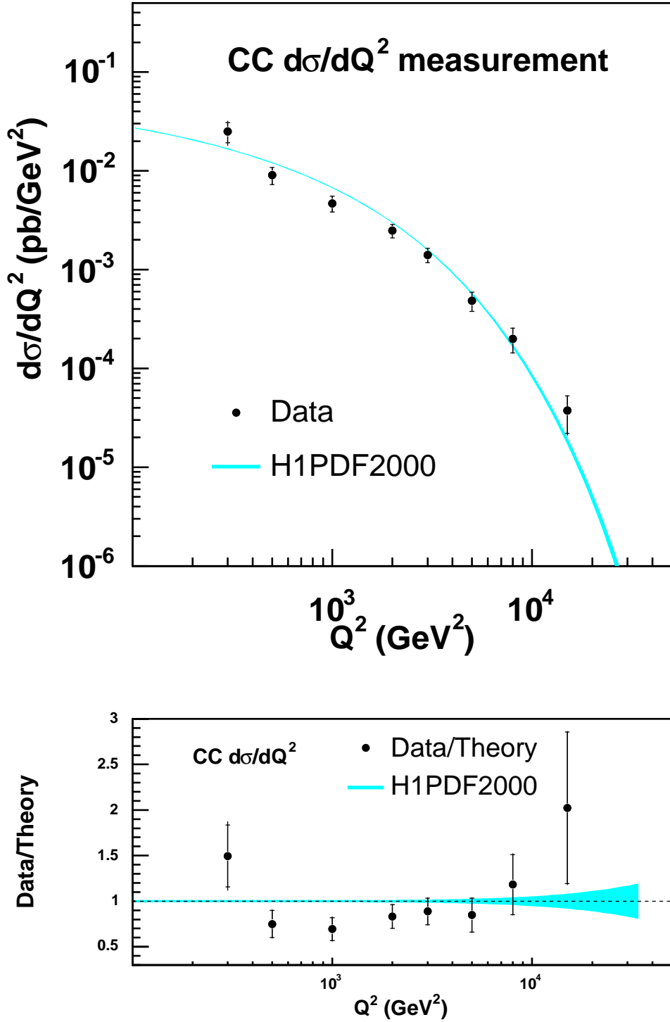
FIG. B.9: Sections efficaces d\sigma/dQ^2 ( y < 0,9 ) pour la période L. Les bandes et barres d'erreurs sont définies comme sur la figure B.8.
