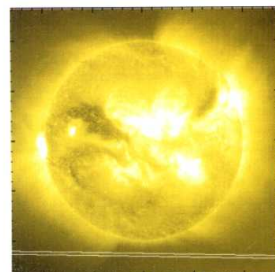
Trajectoire prévue de Vénus, vue par l'instrument EIT du satellite SoHO. Le principal instigateur de EIT est chercheur à IAS ; l'instrument a d'ailleurs été étalonné à l'Institut.
